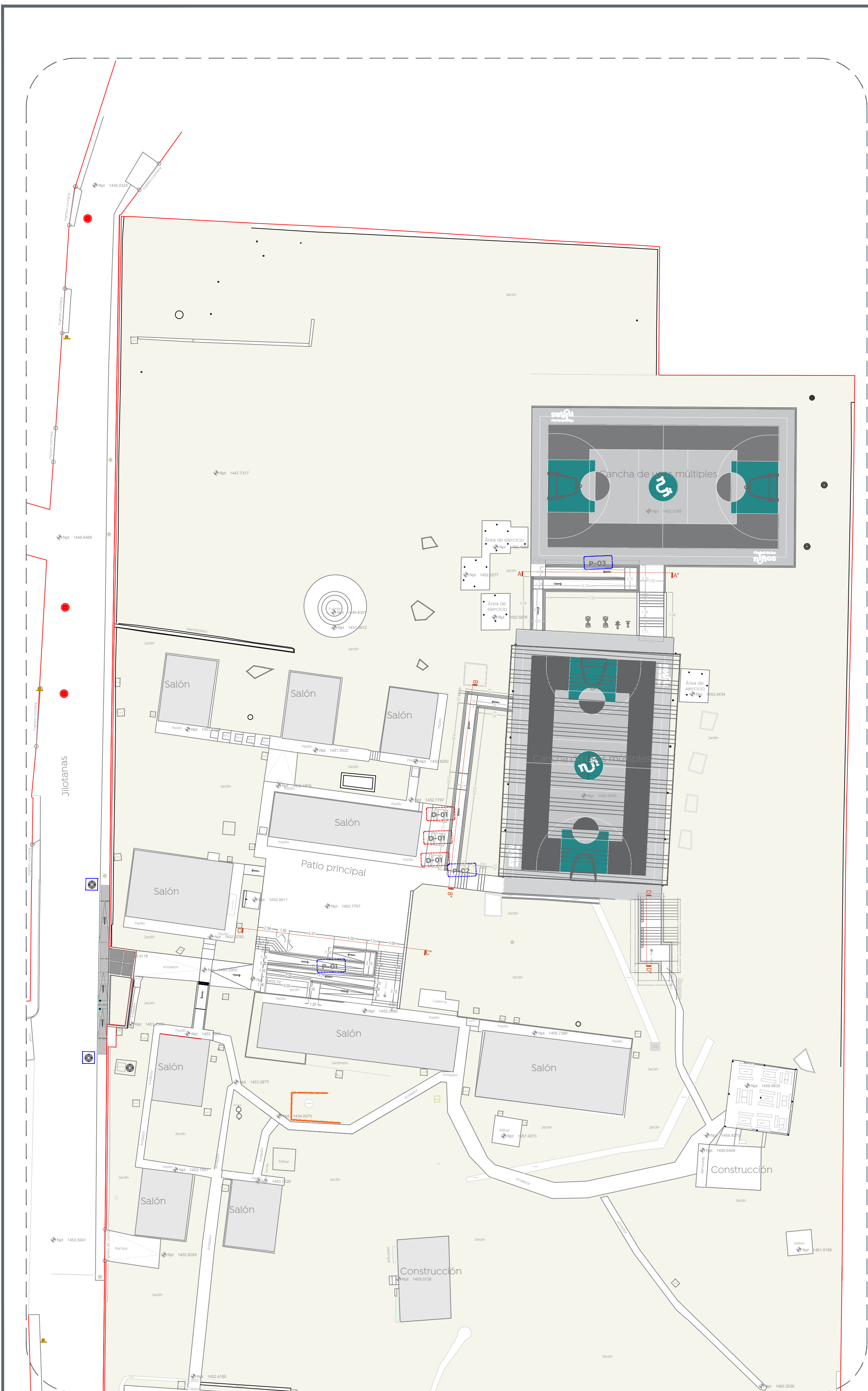
01 Planta de conjunto Albañilería 1:300
