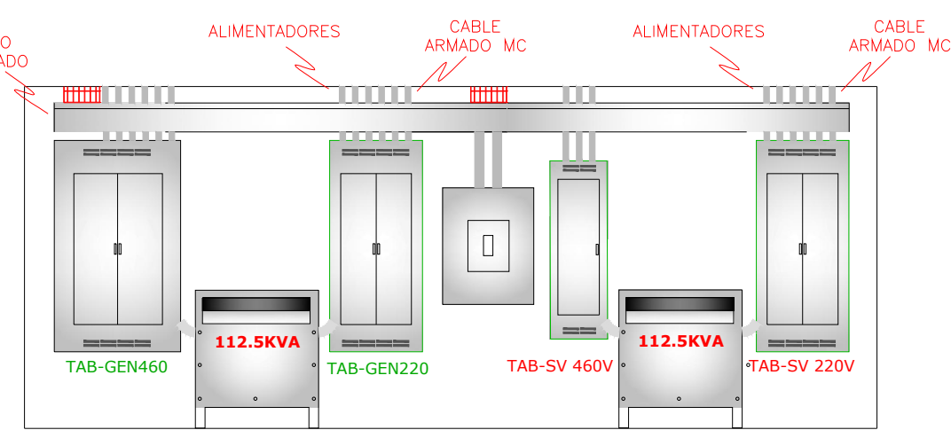
Detalle del Cuarto Eléctrico Cruz Verde Sur Sin escala
