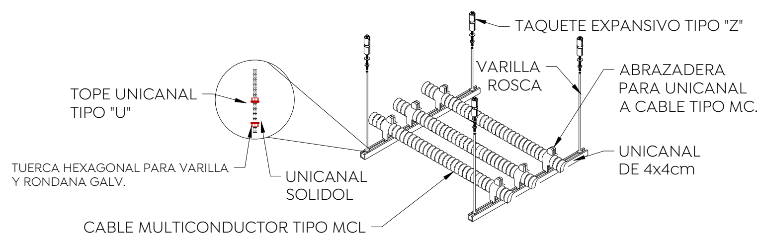
CÉDULA DE CABLEADO ALIMENTADORES
