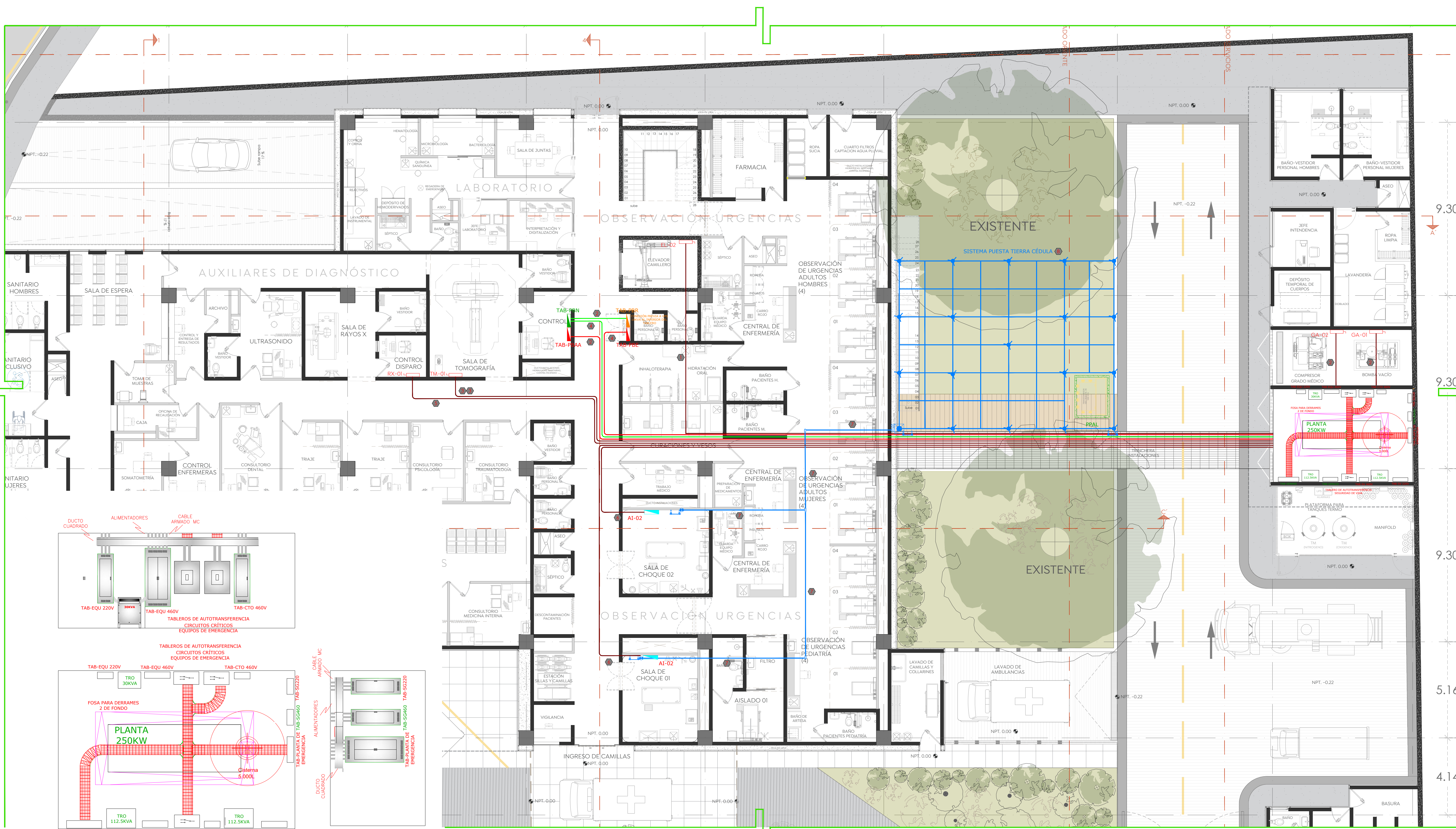
Planta Planta Baja_Alimentadores Cruz Verde Sur Esc. 1:100
