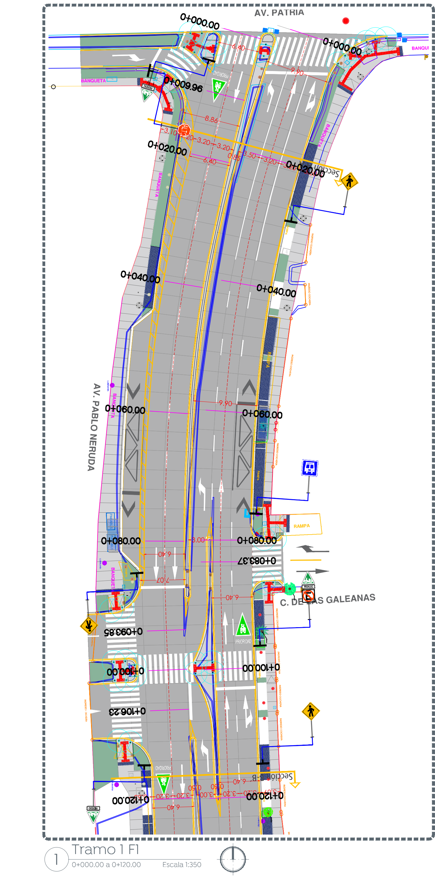
Planta general Escala 1:1000
