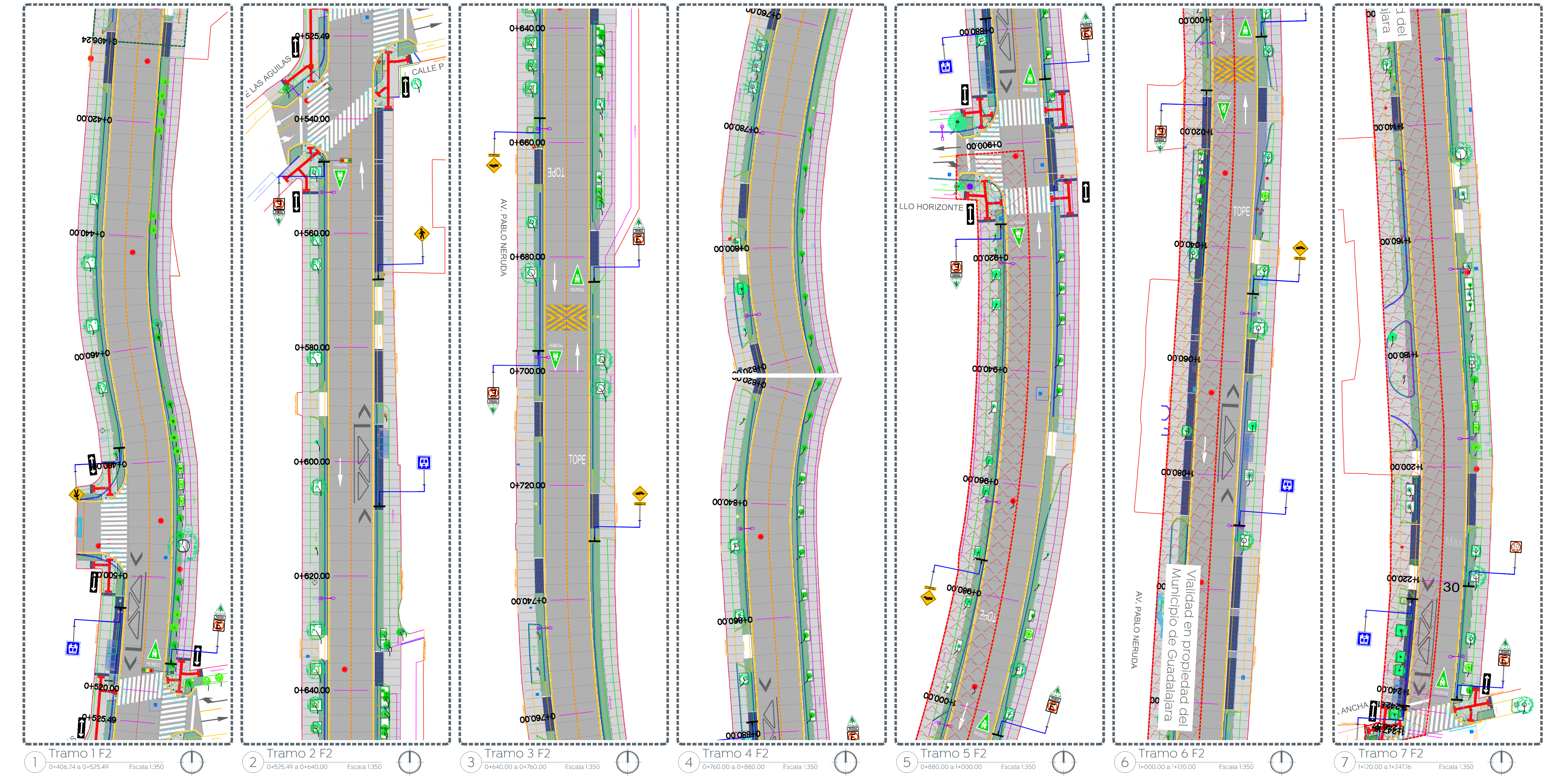
Planta general Escala 1:1000
