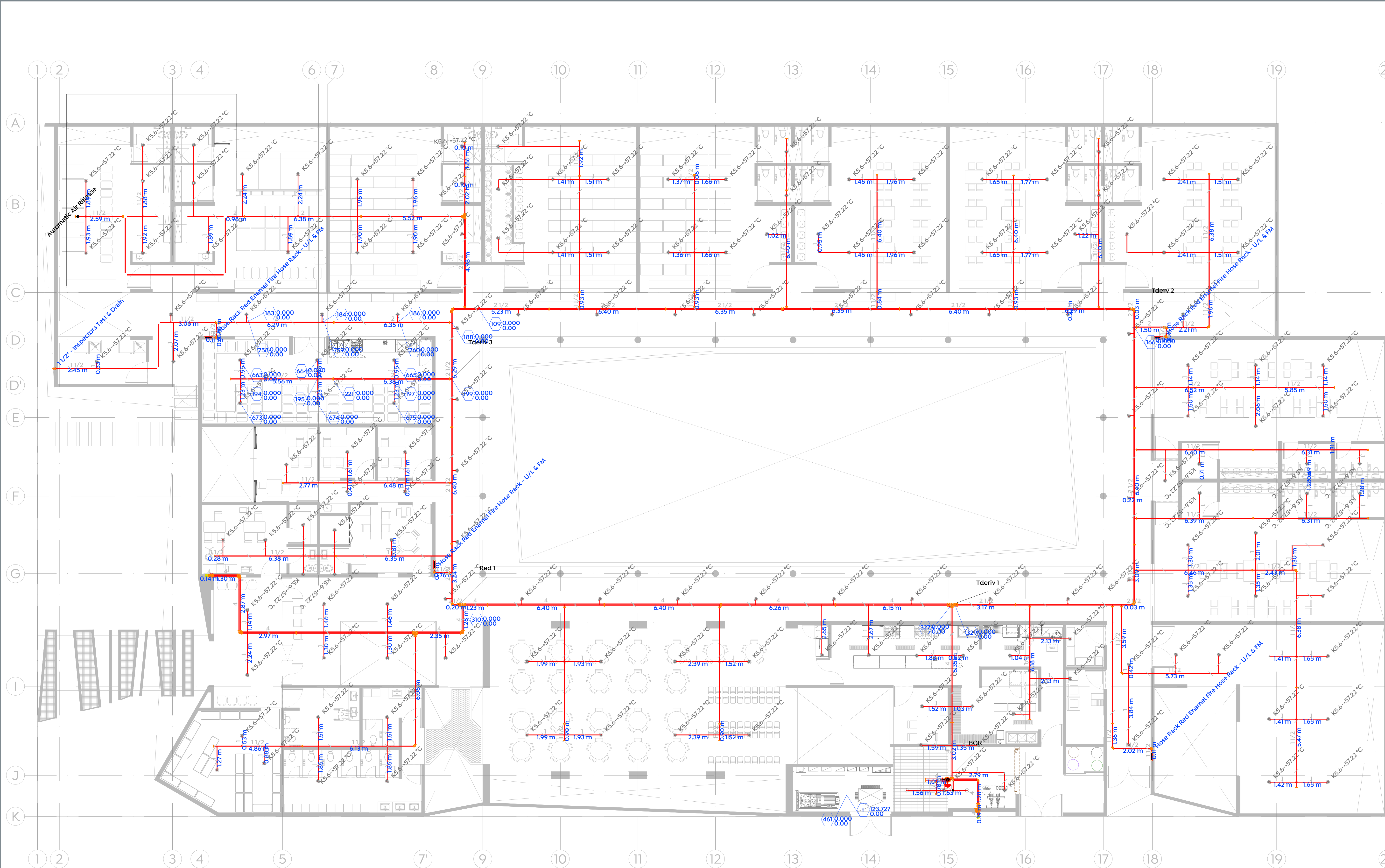
Red de Hidrantes Vista en planta ESCALA 1:100
