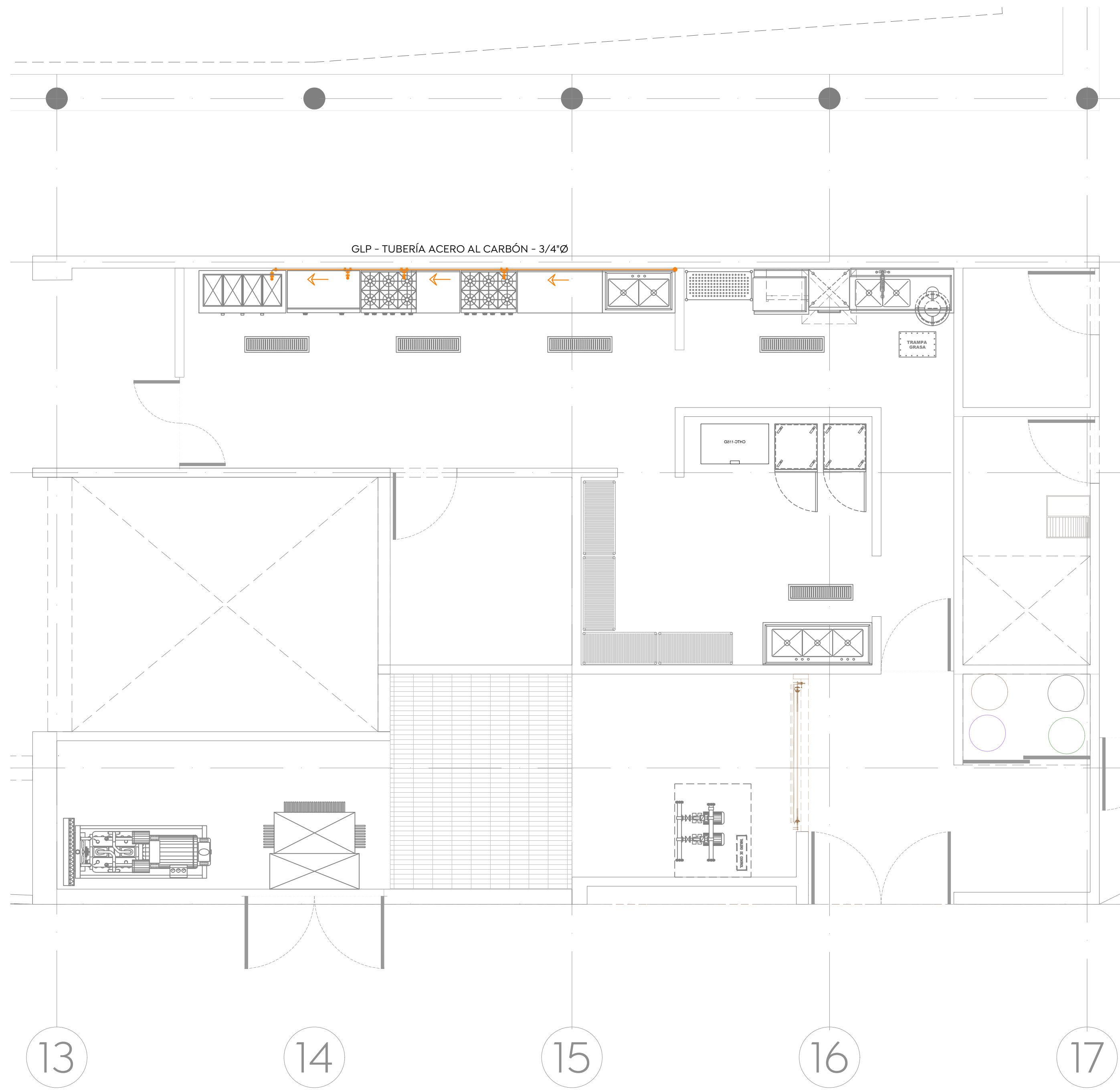
Planta Baja Instalación de Gas L.P. ESCALA 1:50
