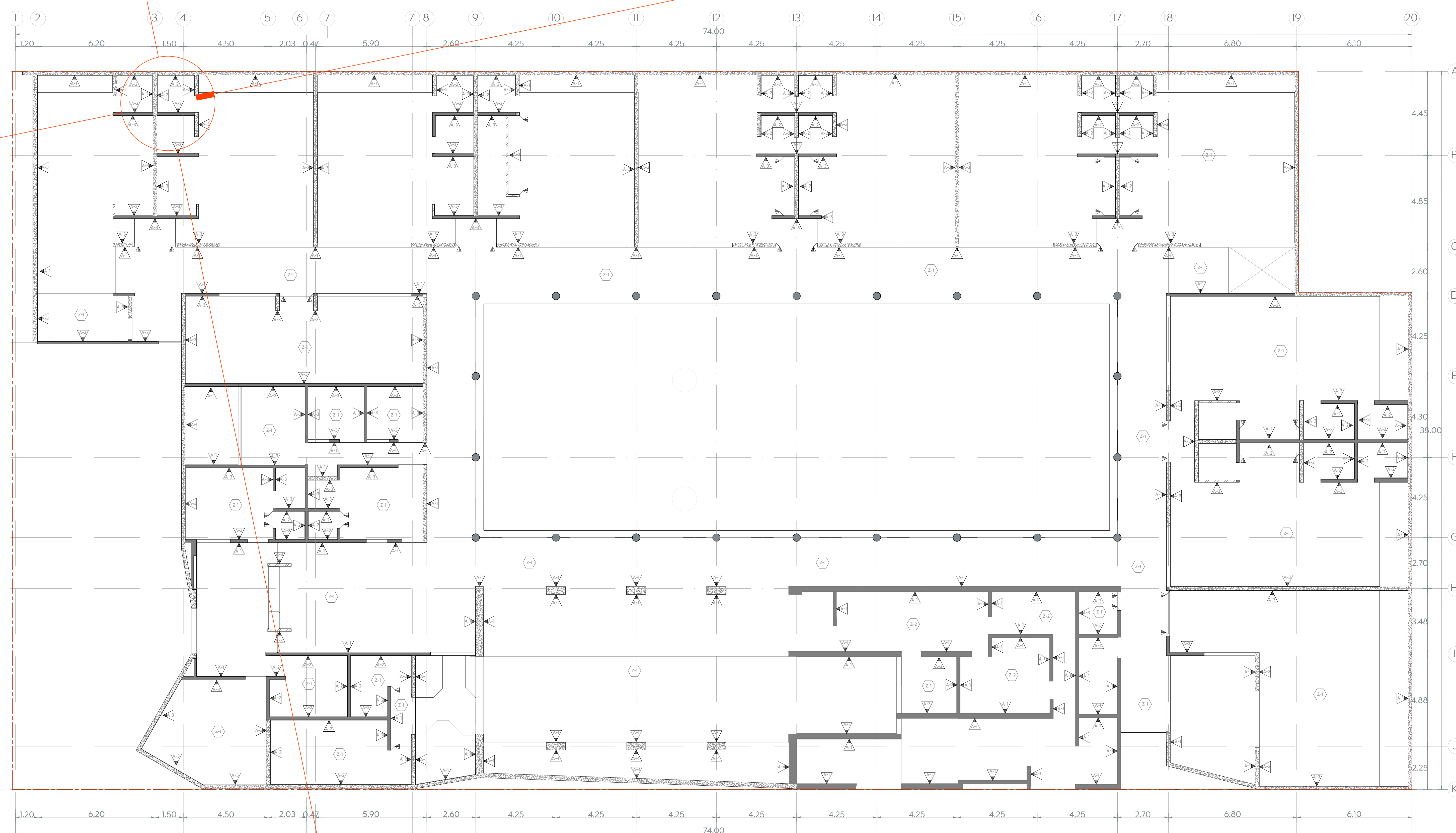
Planta de Acabados en Muros y Lambrines ESCALA 1:100
