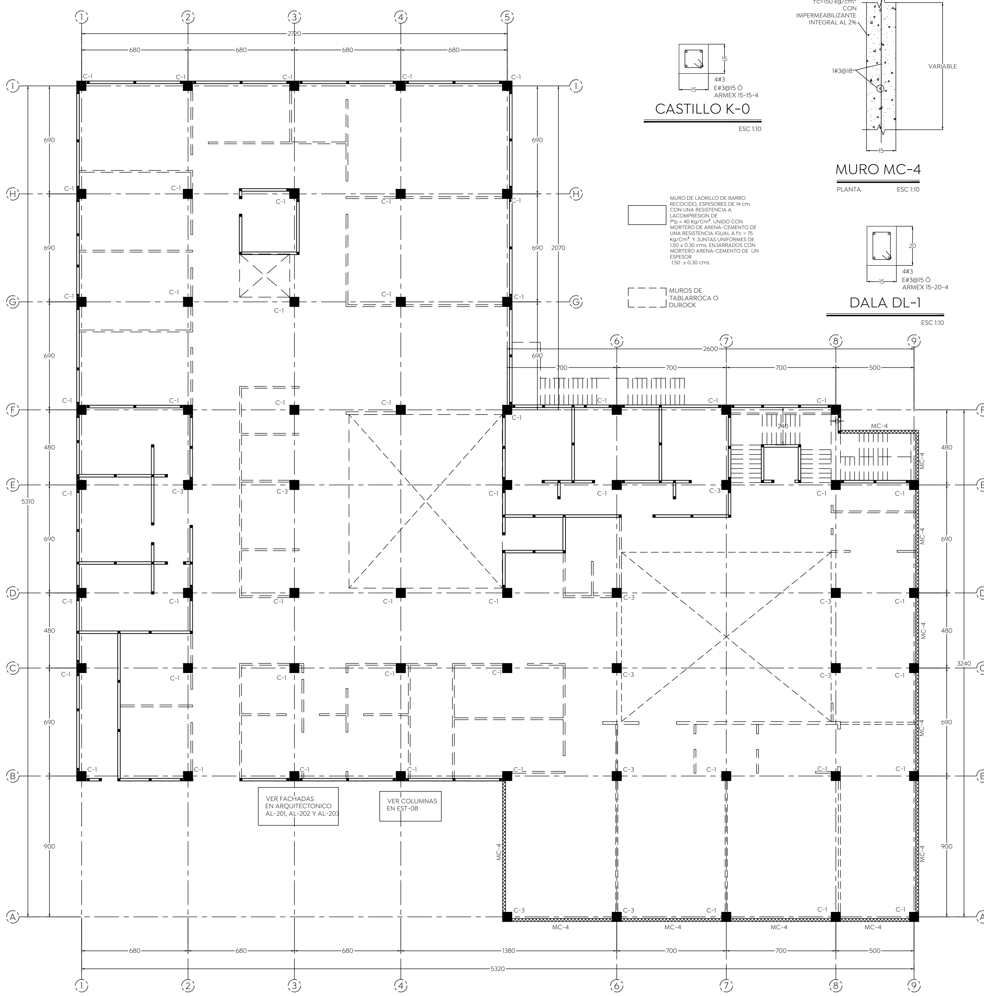
ESTRUCTURACION DE MUROS PLANTA BAJA TODOS LOS CASTILLOS NO NOMBRADOS SON TIPO K-0 ESC 1:25
