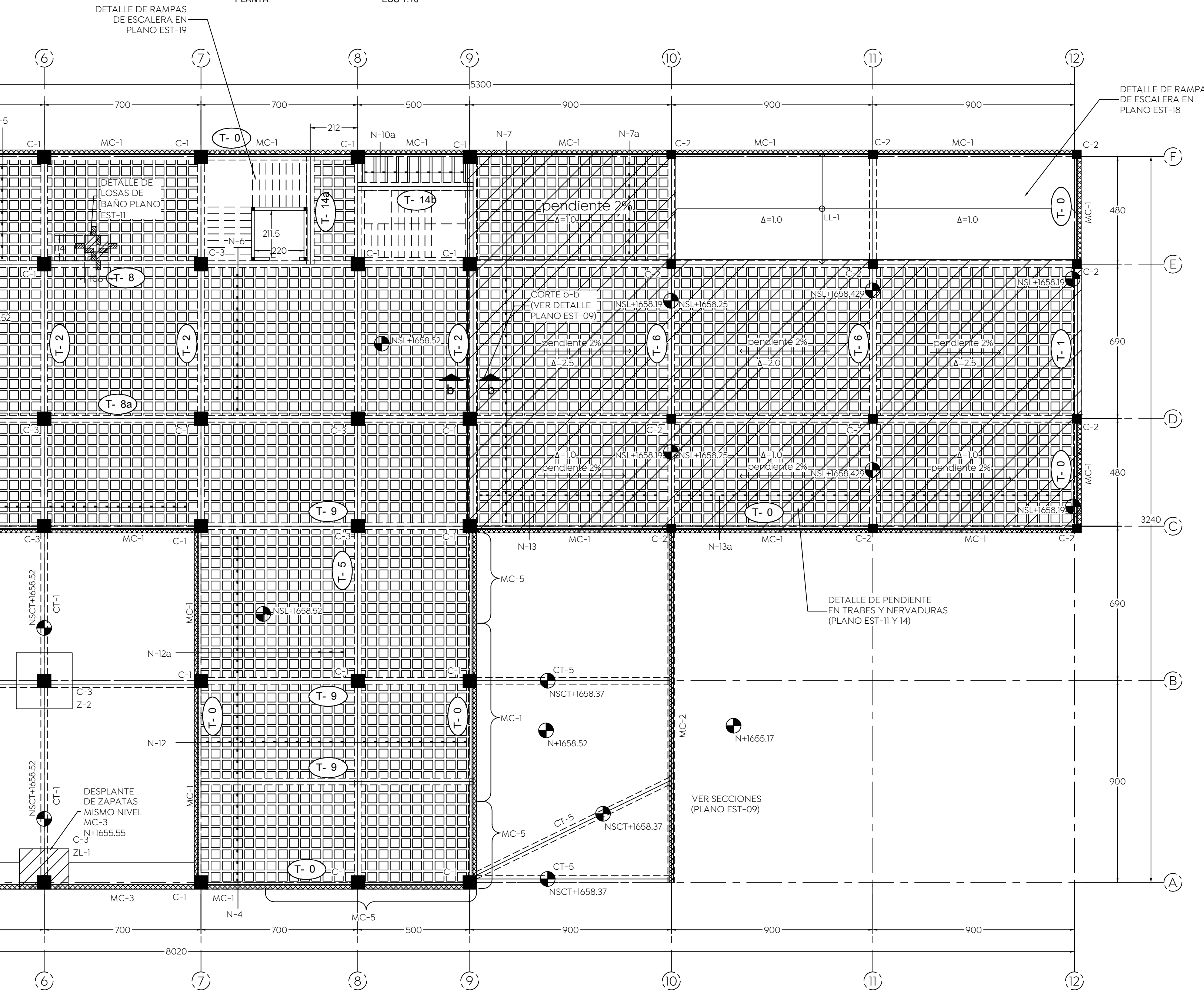
ESTRUCTURACION DE LOSA DE SOTANO N+1658.52 ESC 1:25
