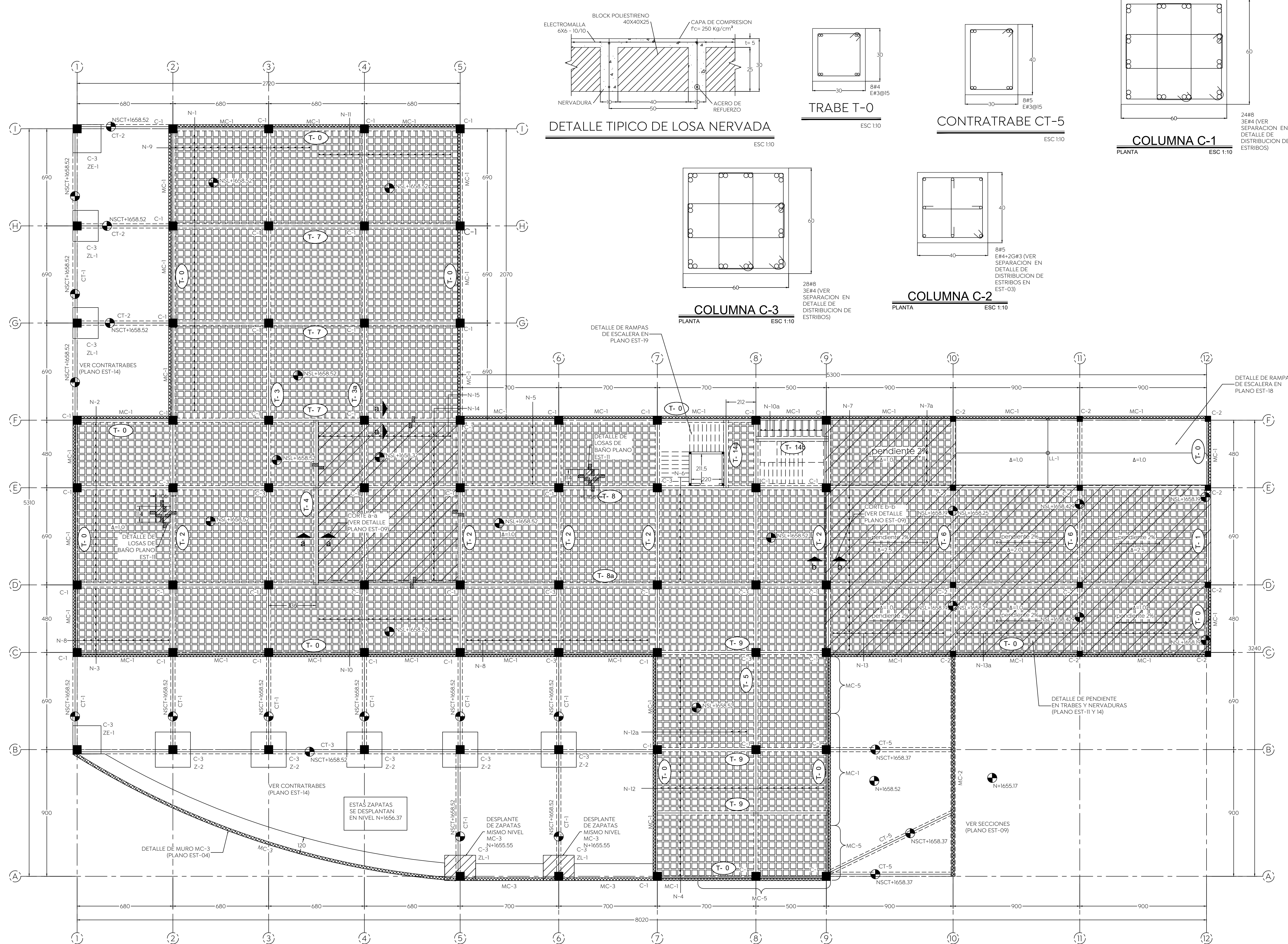
ESTRUCTURACION DE LOSA DE SOTANO N+1658.52 ESC 1:25
