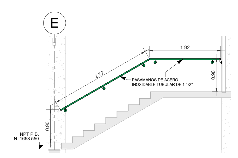
6 SECCION 1-PASAMANOS ESCALA 1 : 50
