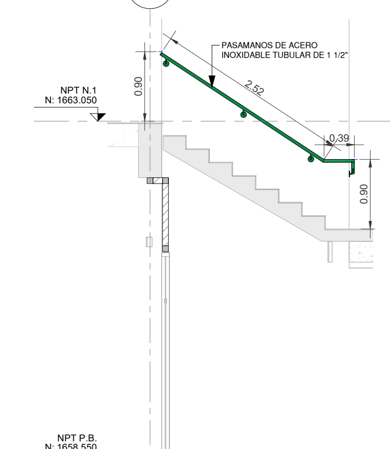
11 SECCION 6-PASAMANOS ESCALA 1 : 50
