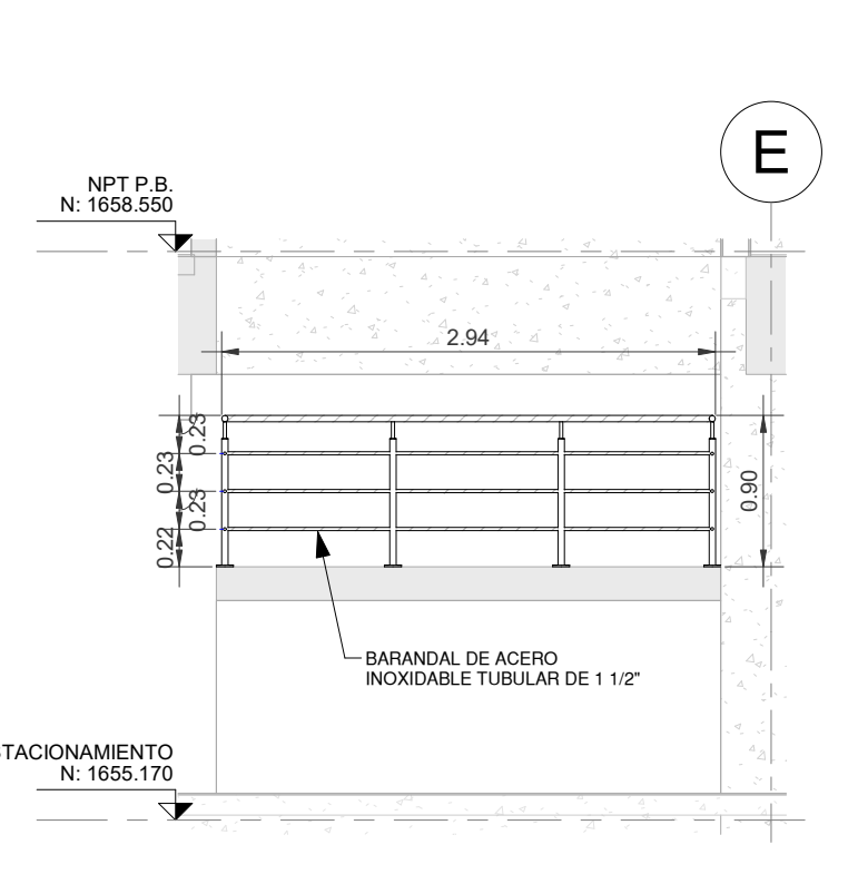
14 SECCION 3-BARANDAL ESCALA 1 : 50
