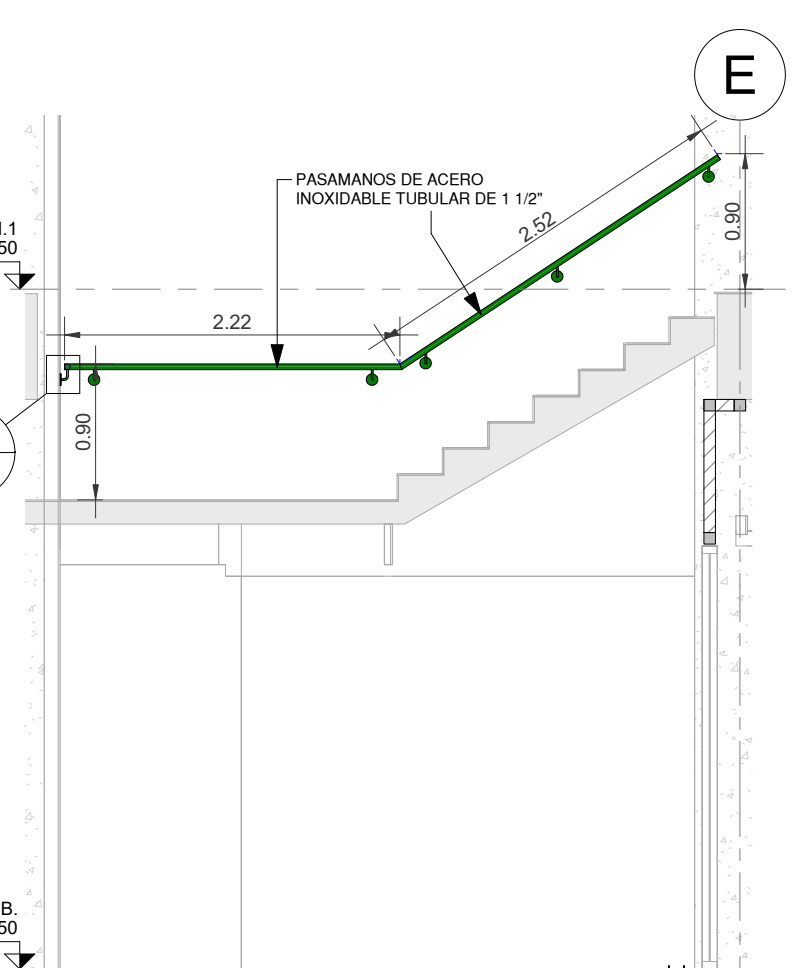
8 SECCION 3-PASAMANOS ESCALA 1 : 50
