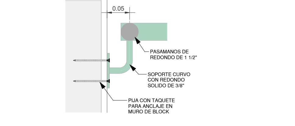
19 ANCLAJE PASAMANOS ESCALA 1 : 5
