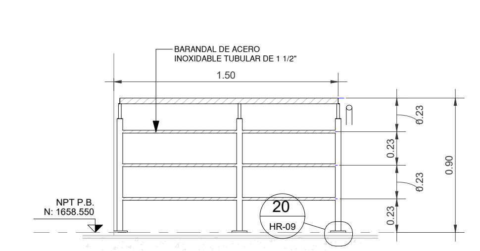
12 SECCION 1-BARANDAL ESCALA 1 : 25
