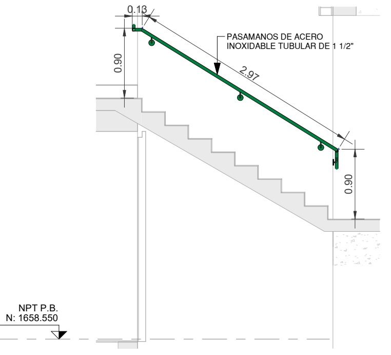
10 SECCION 5-PASAMANOS ESCALA 1 : 50
