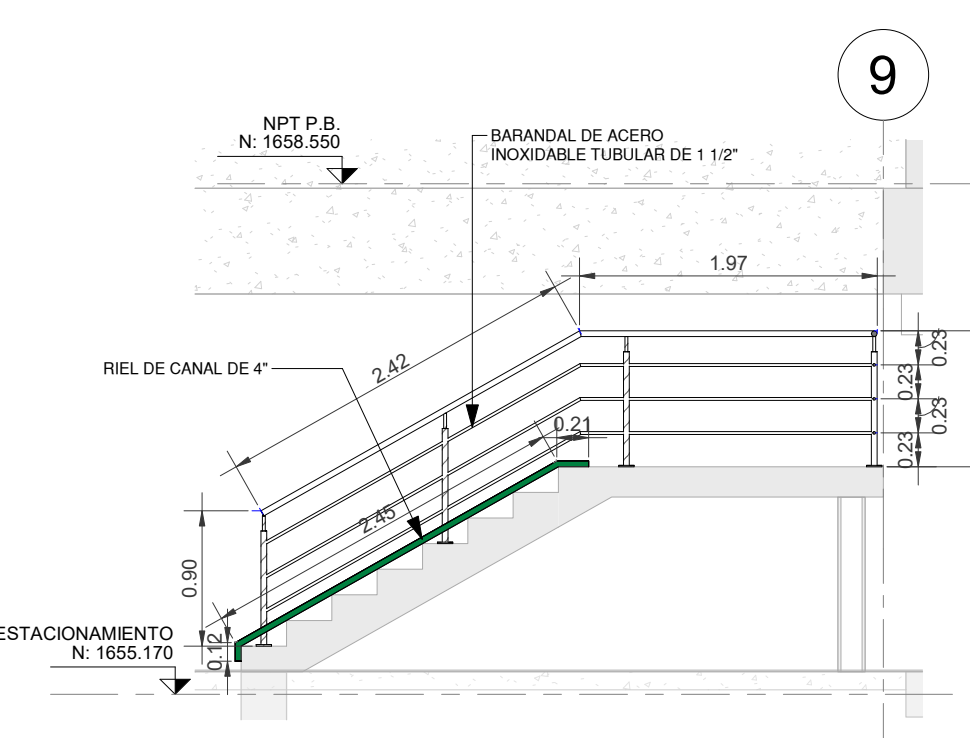
15 SECCION 4-BARANDAL ESCALA 1 : 50
