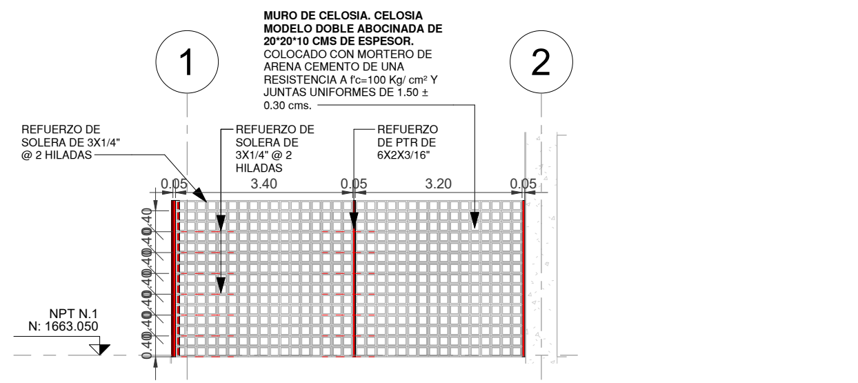
2 ALZADO 2-REFUERZOS CELOSIAS ESCALA 1 : 100
