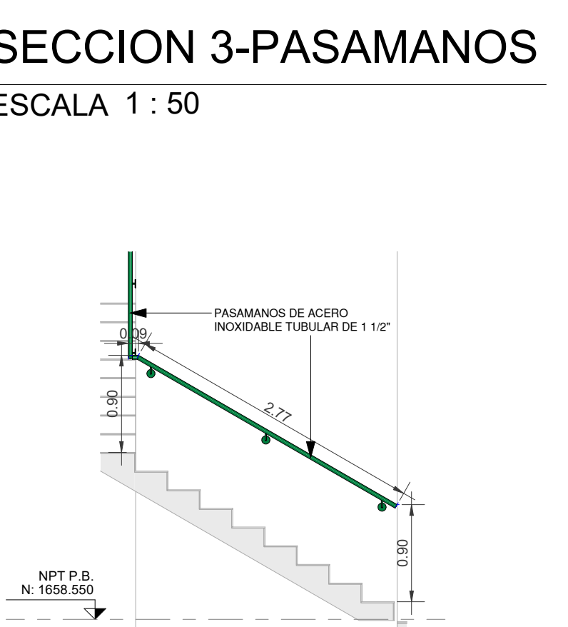
9 SECCION 4-PASAMANOS ESCALA 1 : 50
