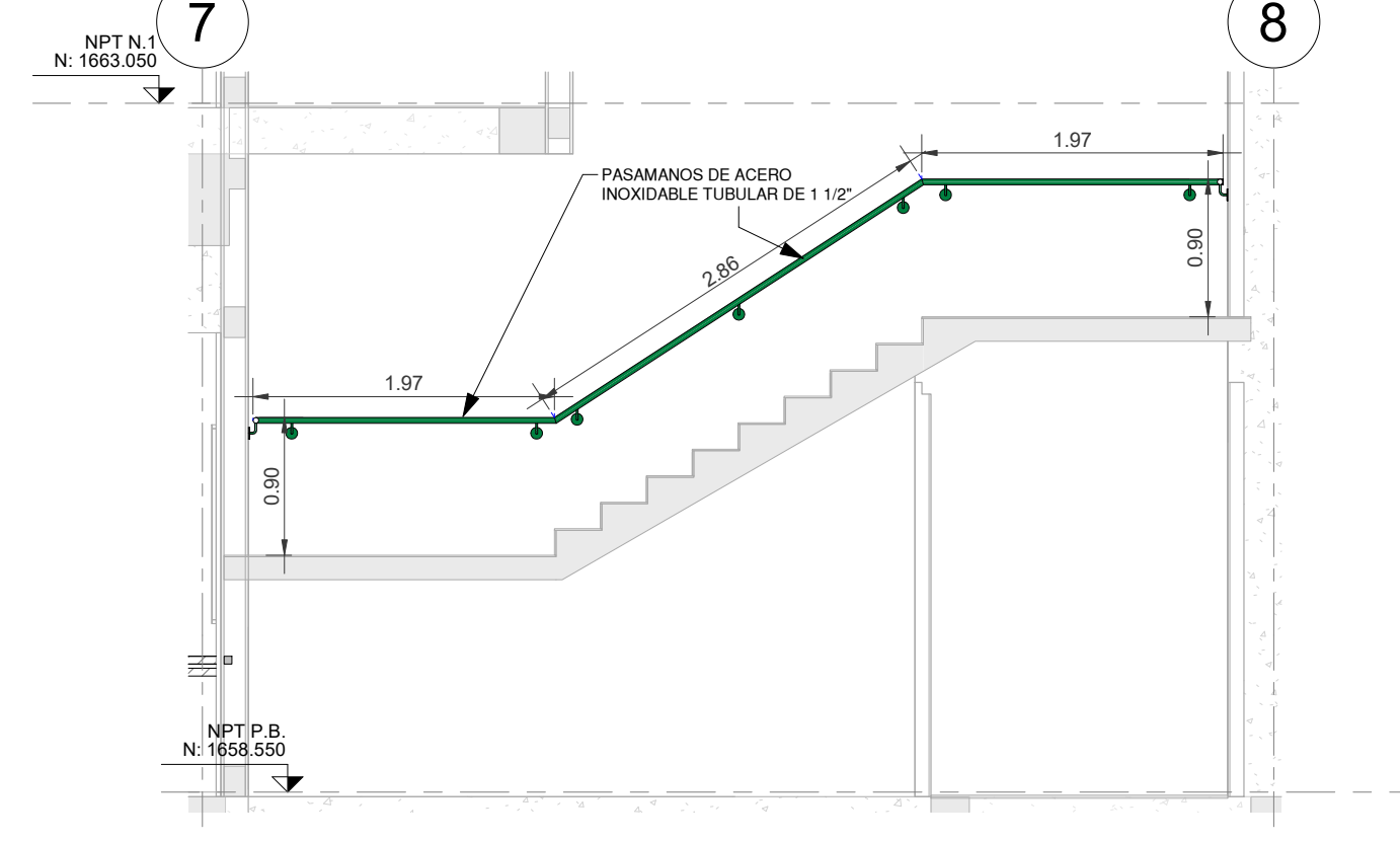
7 SECCION 2-PASAMANOS ESCALA 1 : 50
