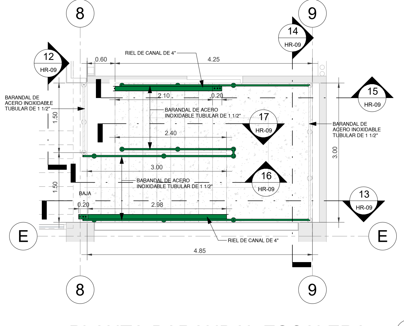
5 PLANTA-BARANDAL ESCALERA ESCALA 1 : 50
