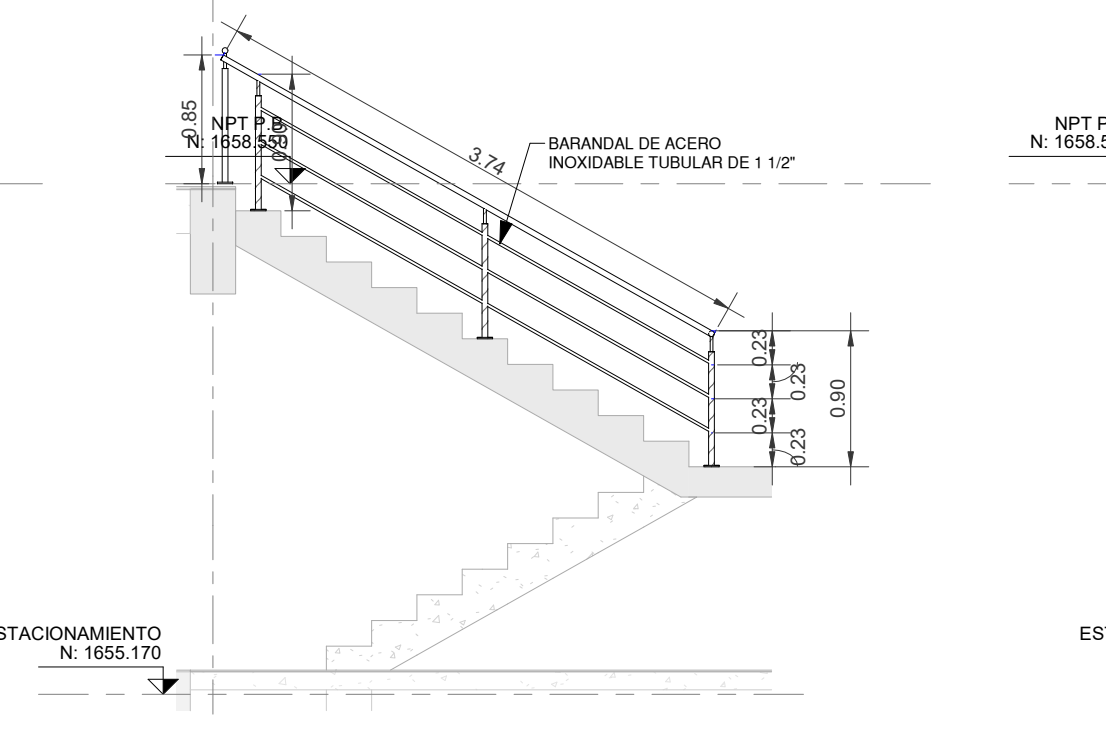
16 SECCION 5-BARANDAL ESCALA 1 : 50
