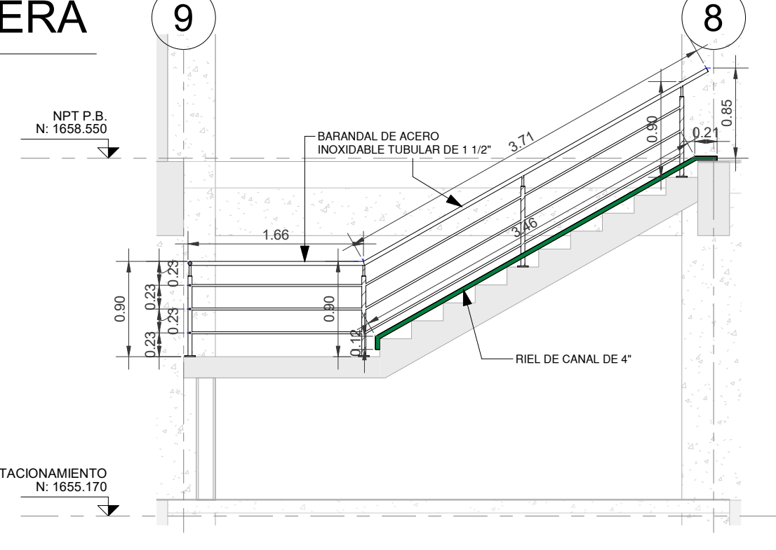
13 SECCION 2-BARANDAL ESCALA 1 : 50
