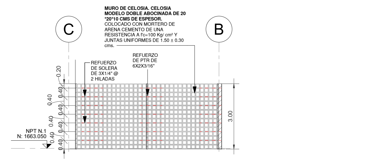
3 ALZADO 3-REFUERZOS CELOSIAS ESCALA 1 : 100
