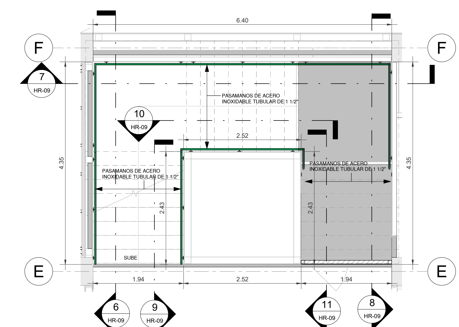
4 PLANTA-PASAMANOS ESCALERA ESCALA 1 : 50
