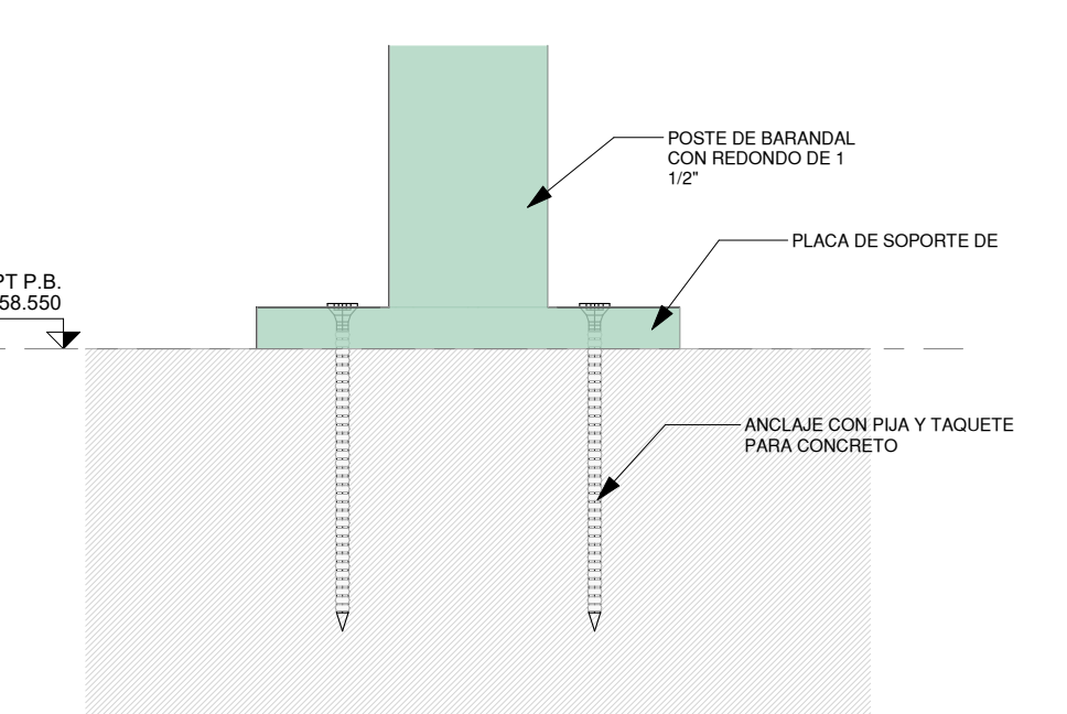
20 ANCLAJE BARANDAL ESCALA 1 : 2
