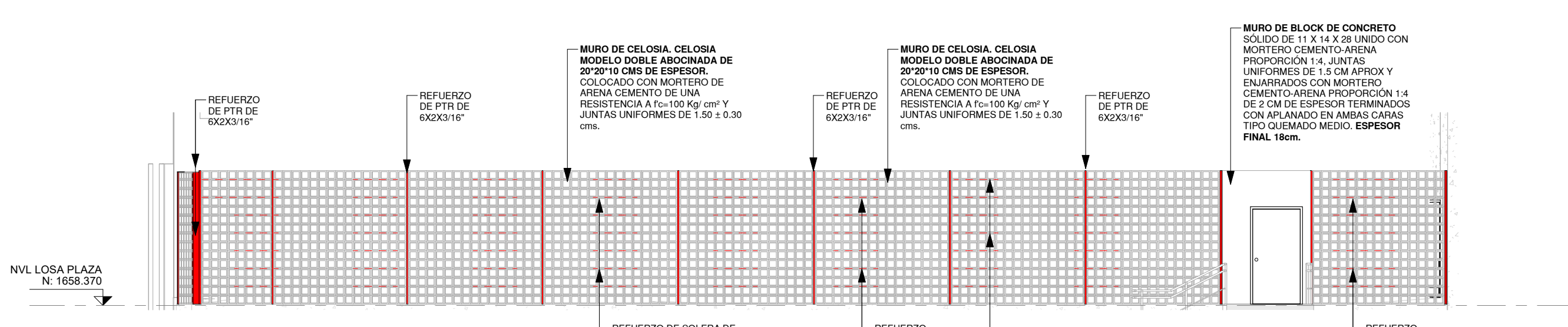
1 ALZADO 1-REFUERZOS CELOSIAS ESCALA 1 : 100
