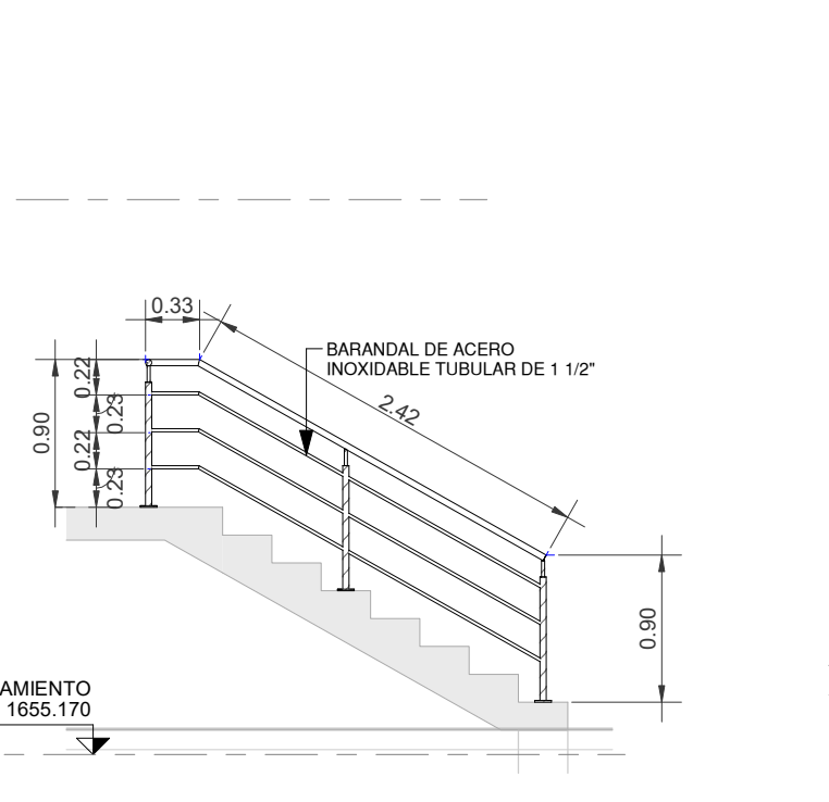
17 SECCION 6-BARANDAL ESCALA 1 : 50
