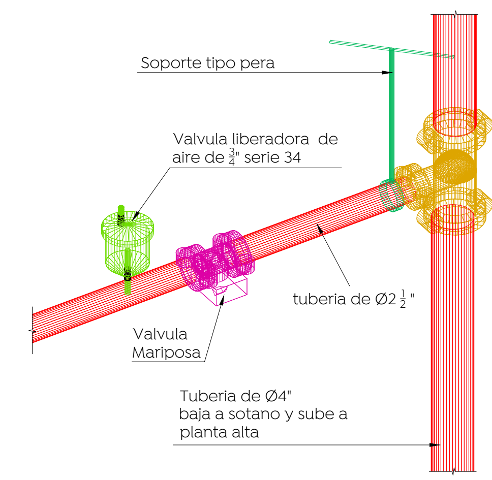
Detalle Válvulas Escala :1:10
