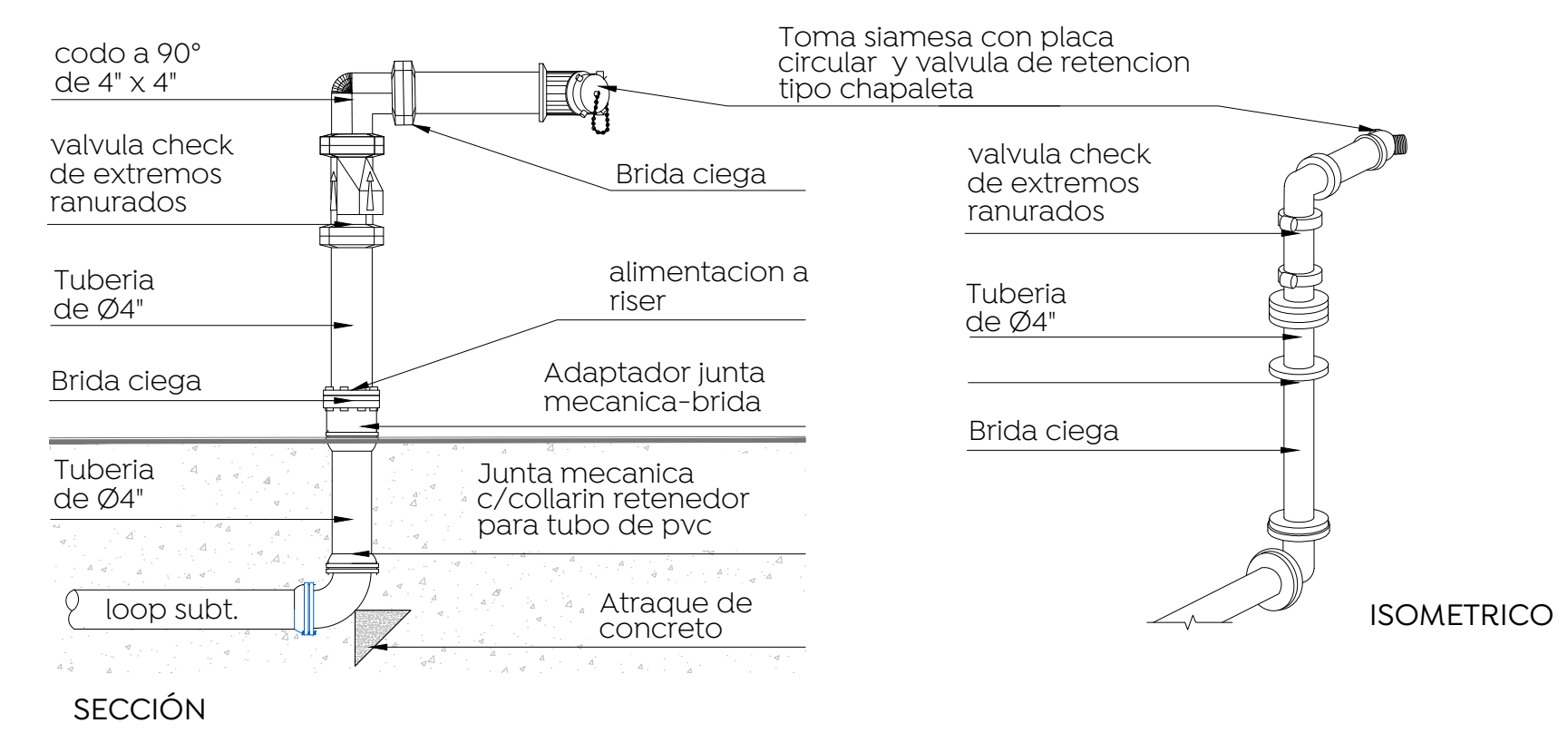
Detalle Toma siamesa Esc. Sin
