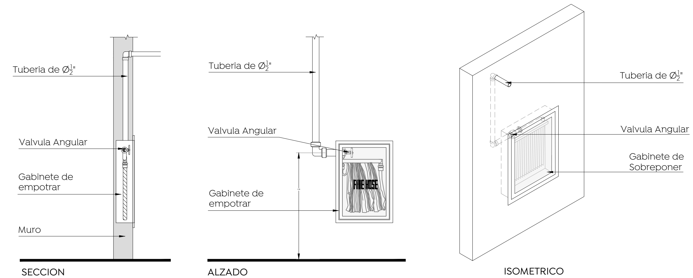
Detalle Hidrante de Empotrar Esc. Sin
