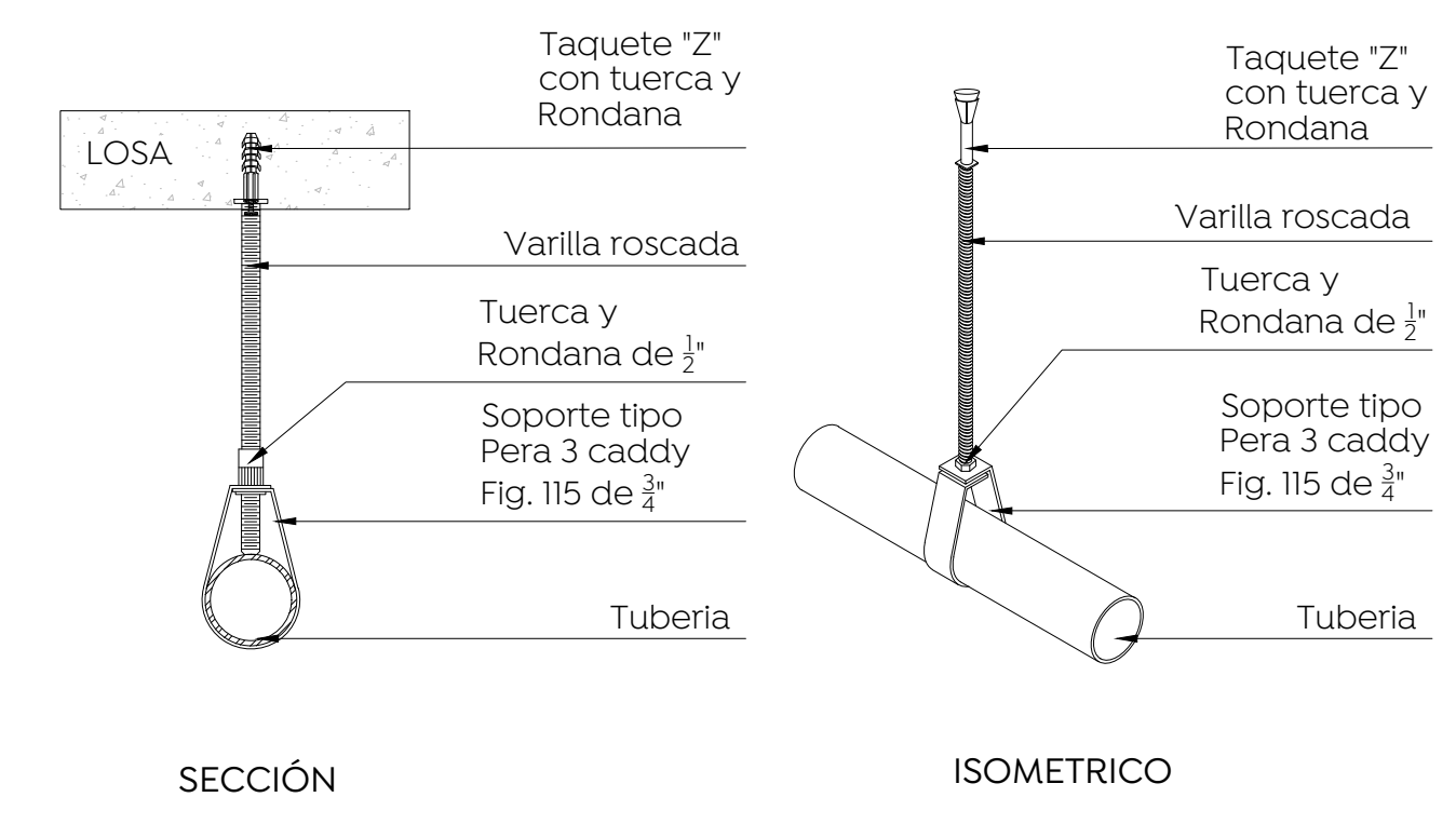
Detalle Soporte tipo pera Esc. Sin
