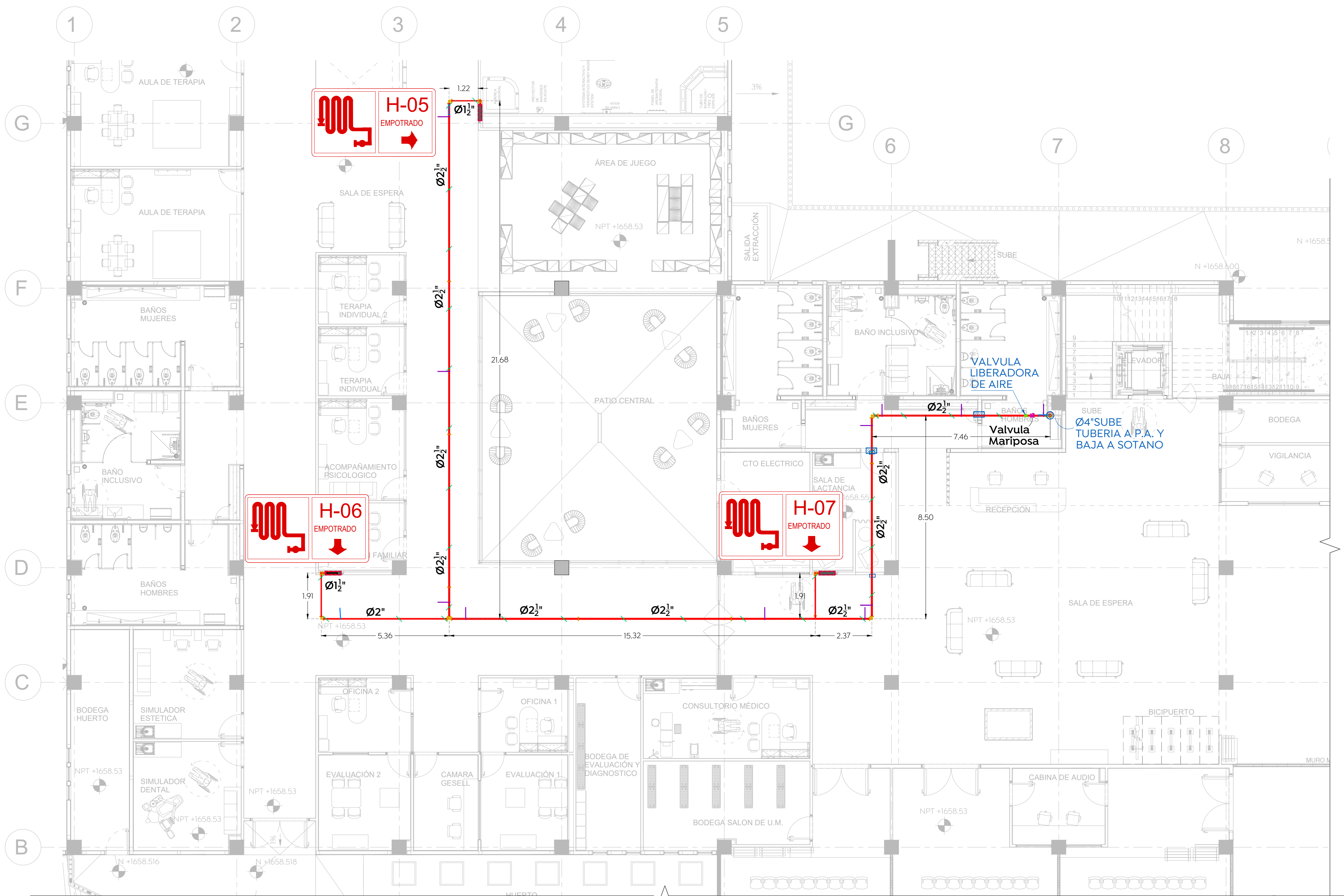
Planta Baja Planta de Protección Contra Incendios Esc. 1:100
