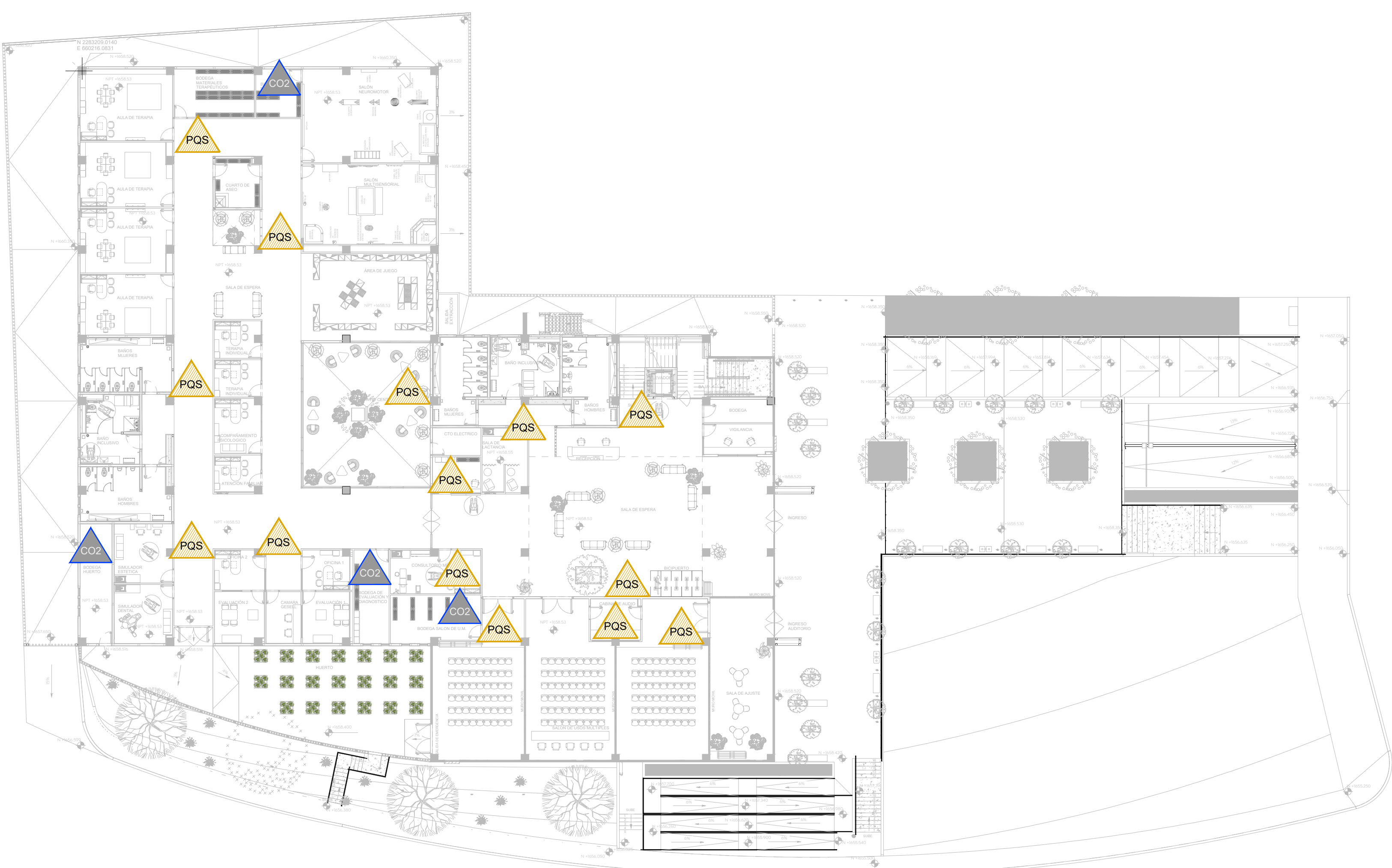
Planta Baja Planta de Distribución de Extintores Esc. 1:250
