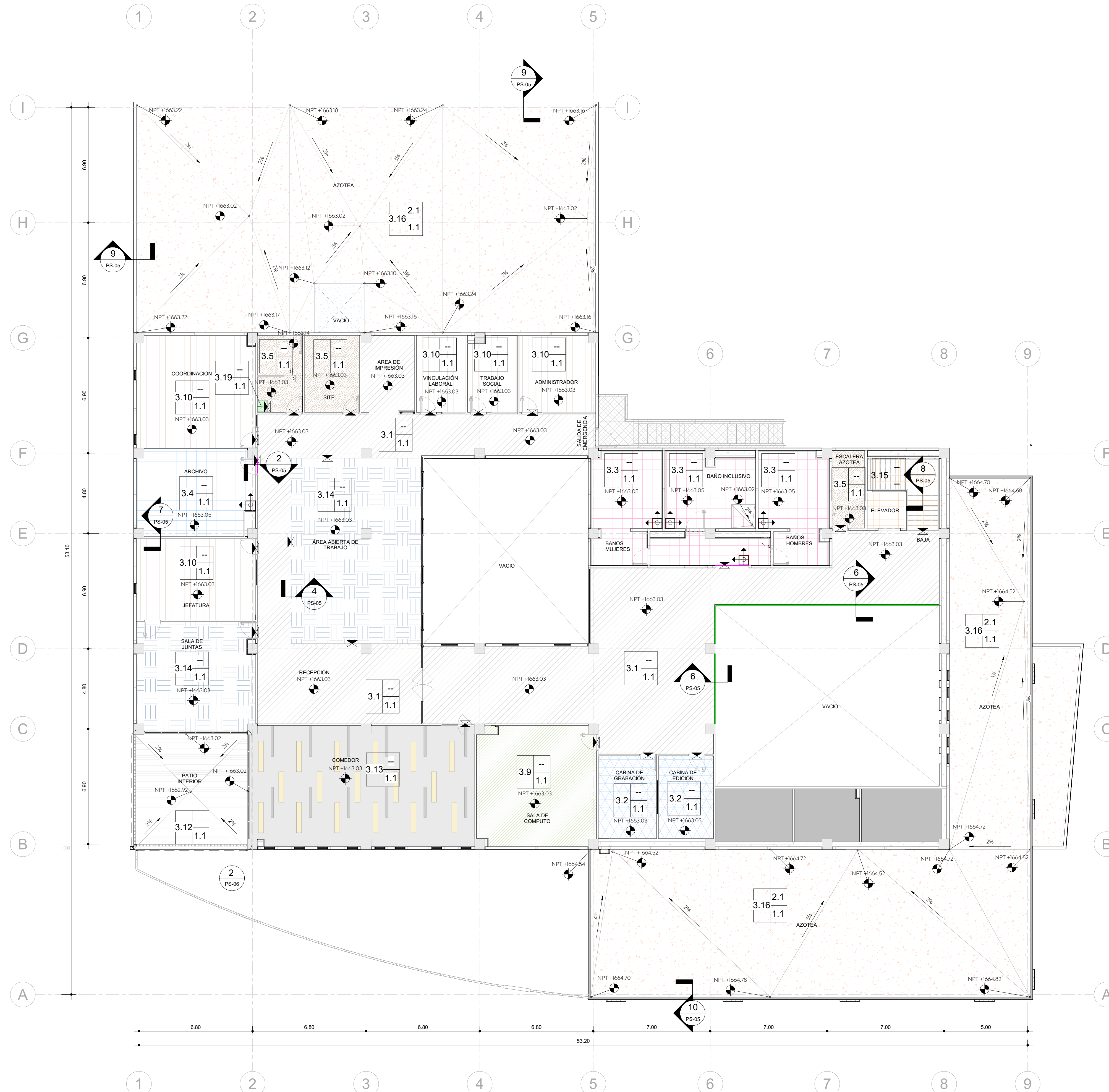
1 ACABADOS PISOS PLANTA NIVEL 1 ESCALA 1 : 125
