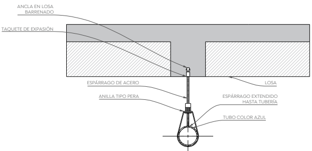
SCALL-06 Sujeción de bajantes a losa (Alzado frontal) Cruz verde Esc. 1:10
