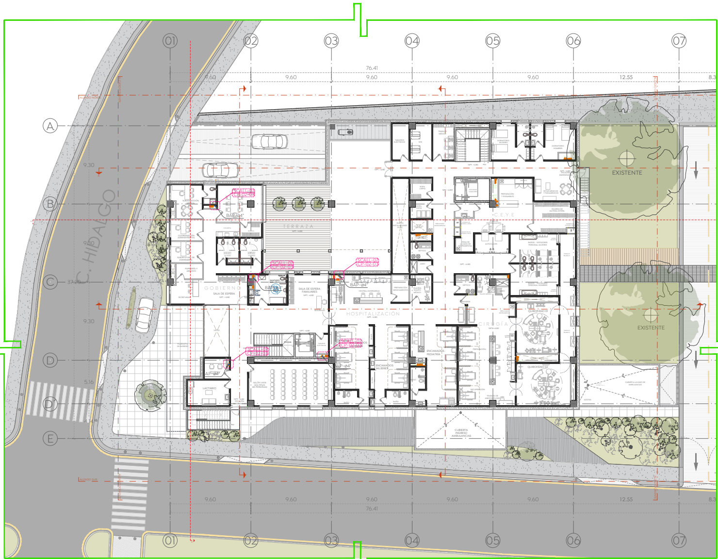
Planta Baja_Conсульта Cruz Verde Sur Esc. 1:200
