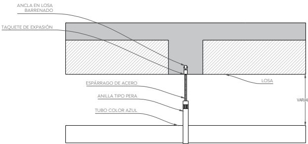
SCALL-06 Sujeción de bajantes a losa (Alzado lateral) Cruz verde Esc. 1:10
