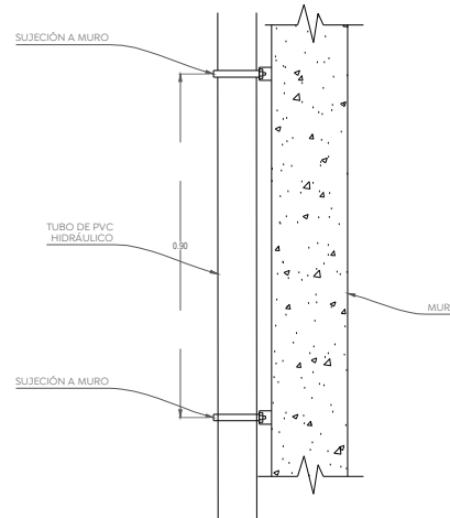
SCALL-07 Sujeción de bajantes a muro (Alzado) Cruz verde Esc. 1:10
