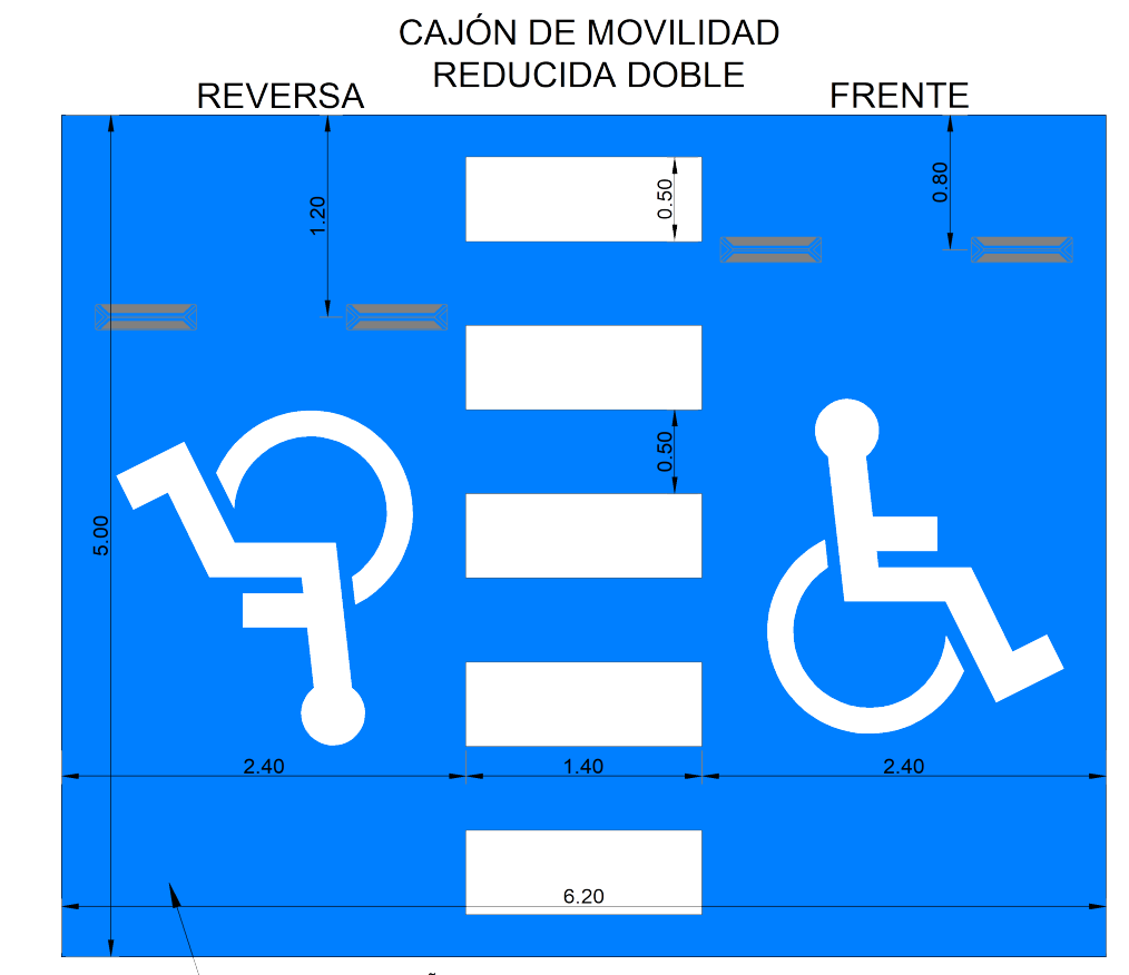
02 - DETALLES DE CAJONES ESC: 1:50
