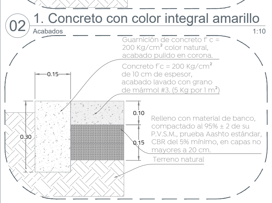
02 2. Concreto lavado 1:10
