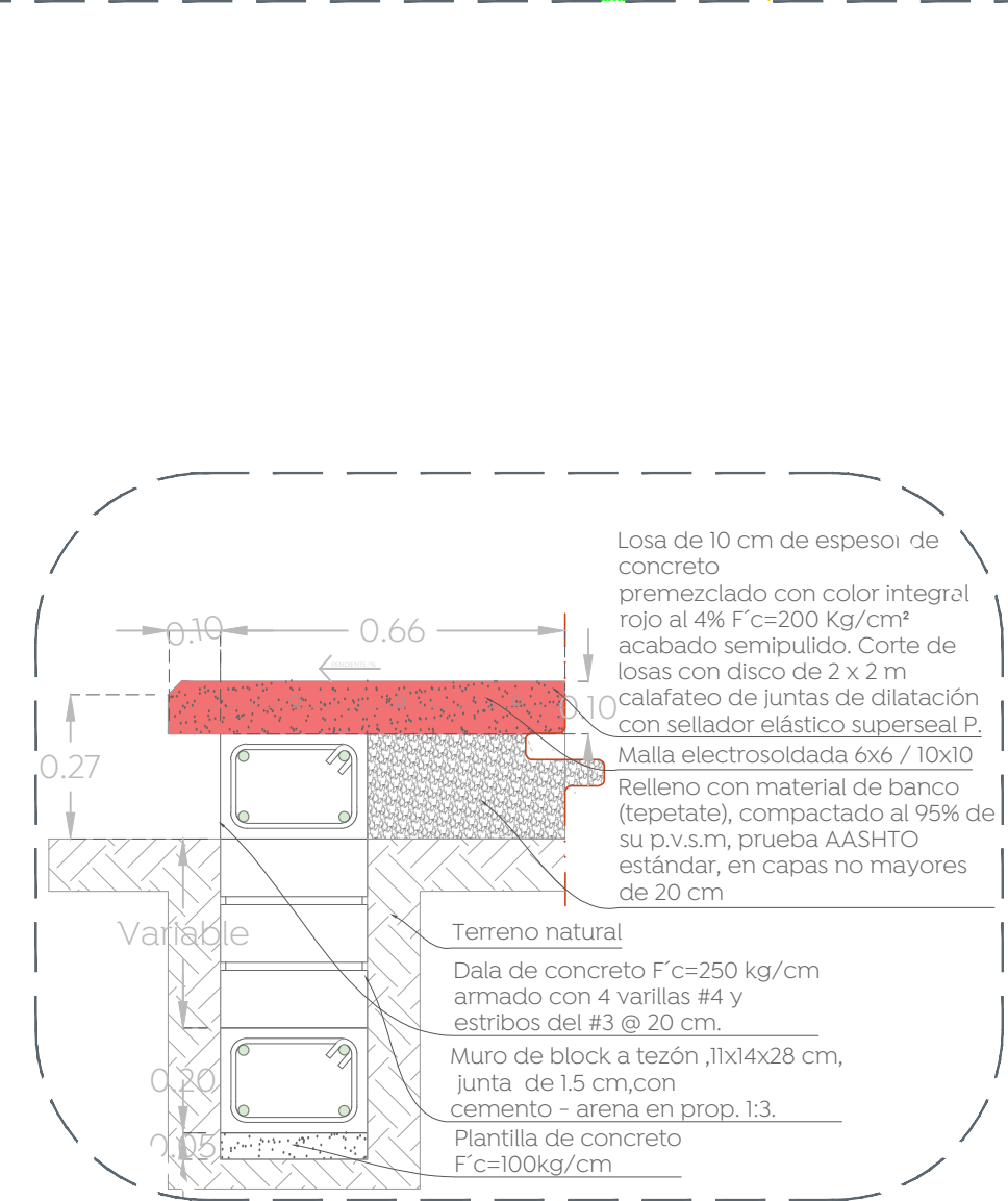
05 4. Concreto en cancha de usos múltiples 1:10
