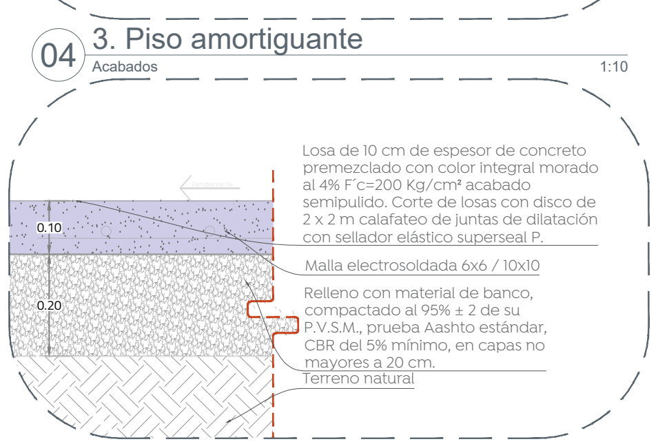
04 3. Piso amortiguante 1:10
