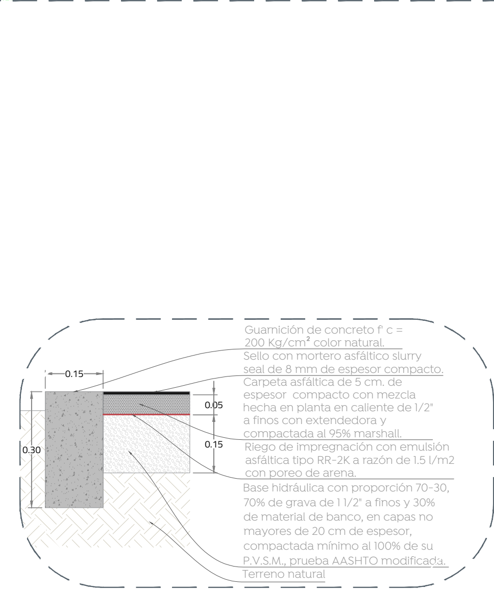
06 5. Concreto en cancha de usos múltiples 1:15
