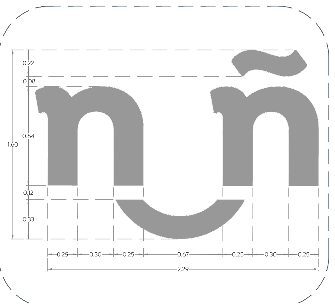
03 Detalle de balizamiento d.2 1:20
