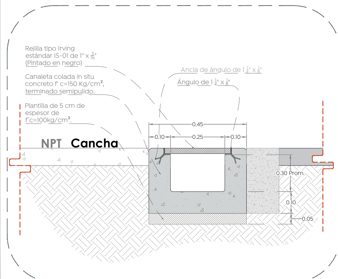
02 Detalle de canaleta d.1 1:10
