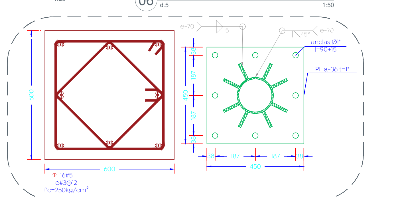
08 Detalle de canasta
