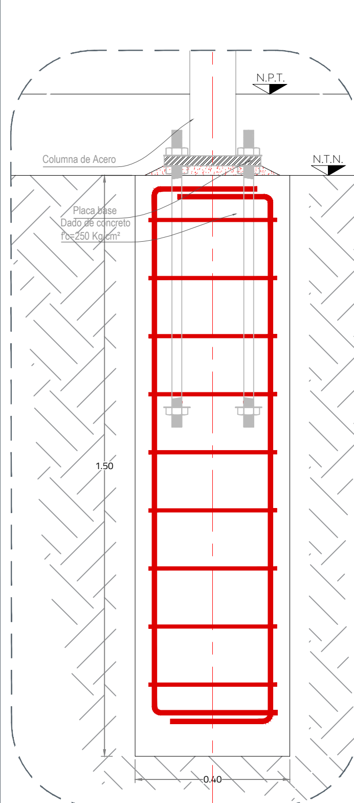
02 Detalle de backstop
