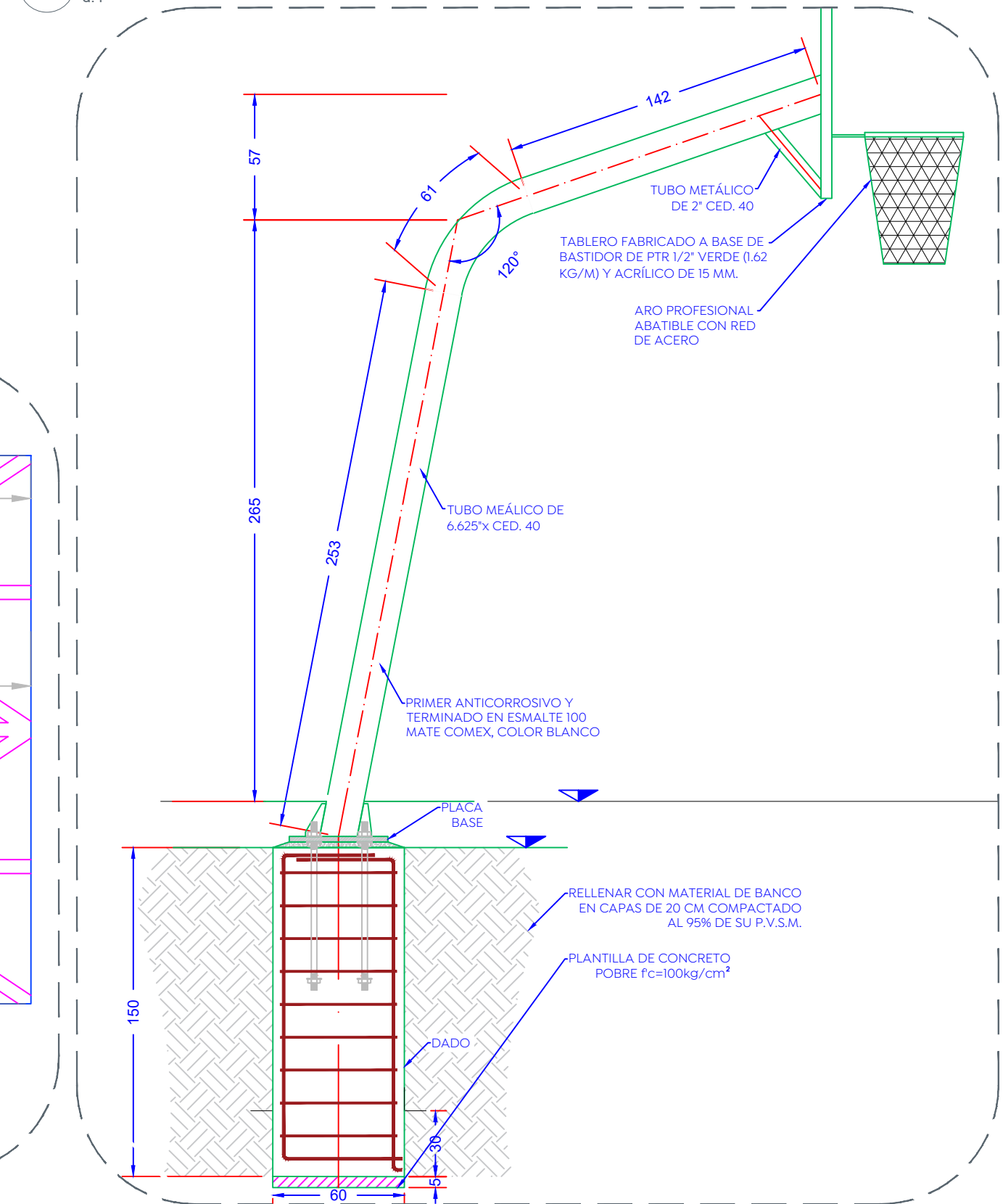
07 Alzado de canasta
