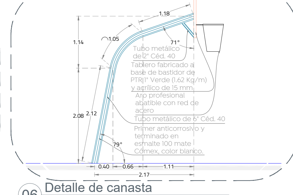
06 Detalle de canasta
