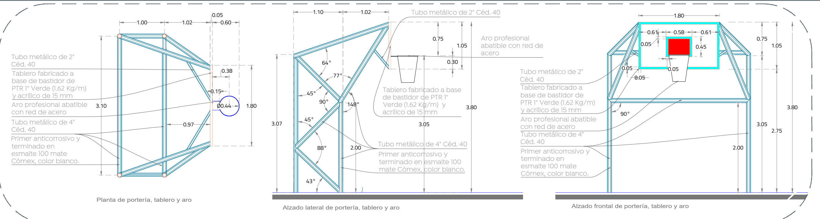
04 Detalle de portería de usos múltiples
