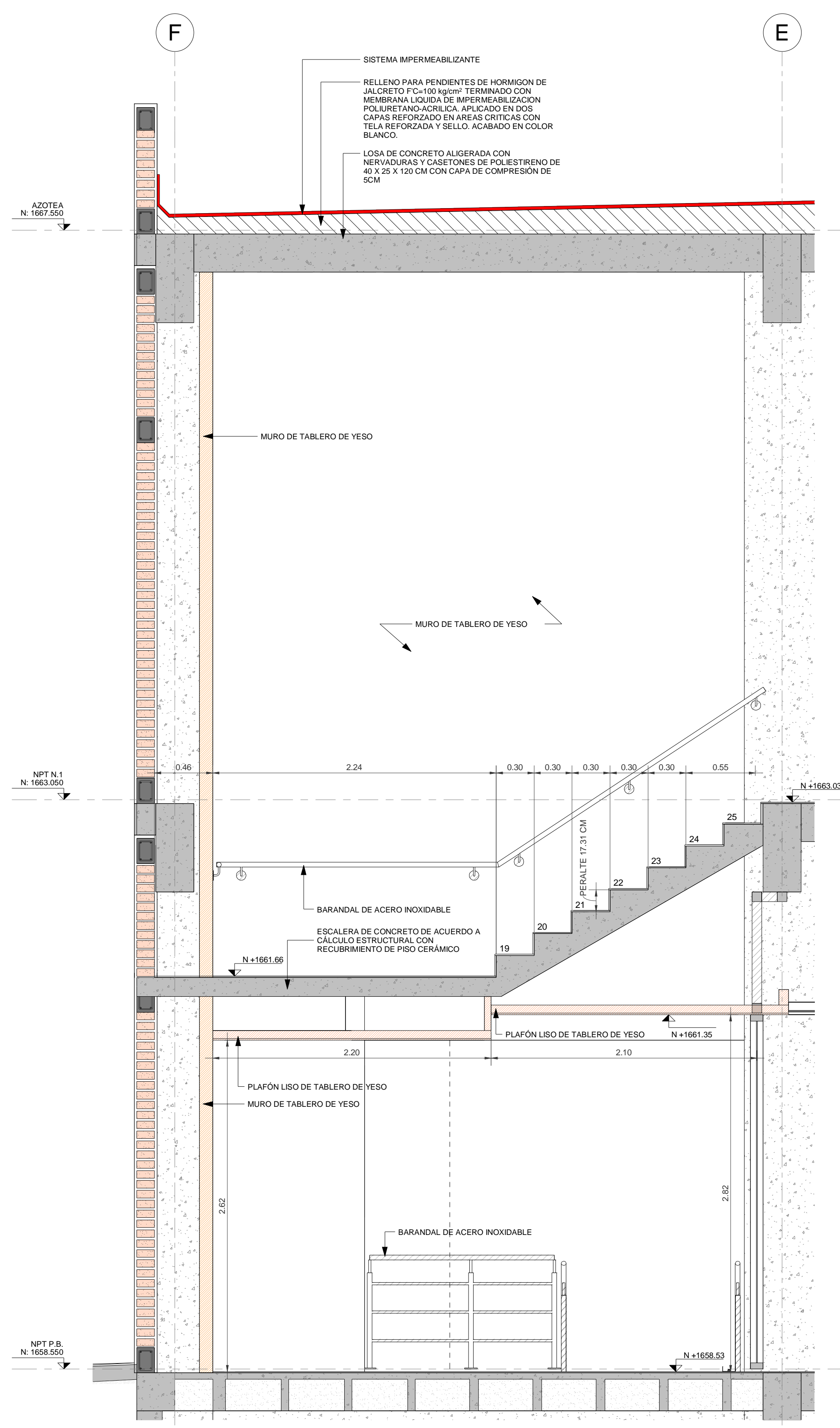
2 SECCIÓN A DETALLE ESCALERA -3- ESCALA 1 : 25
