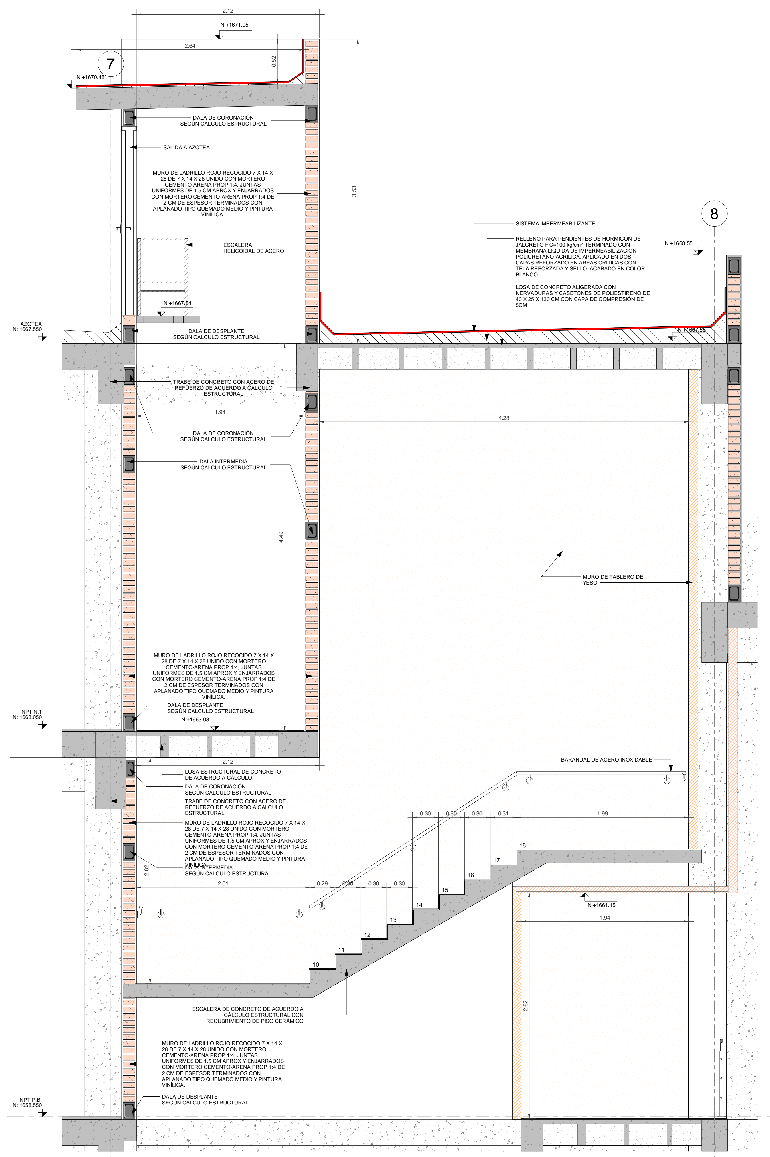
1 SECCIÓN A DETALLE ESCALERA -2- ESCALA 1 : 25
