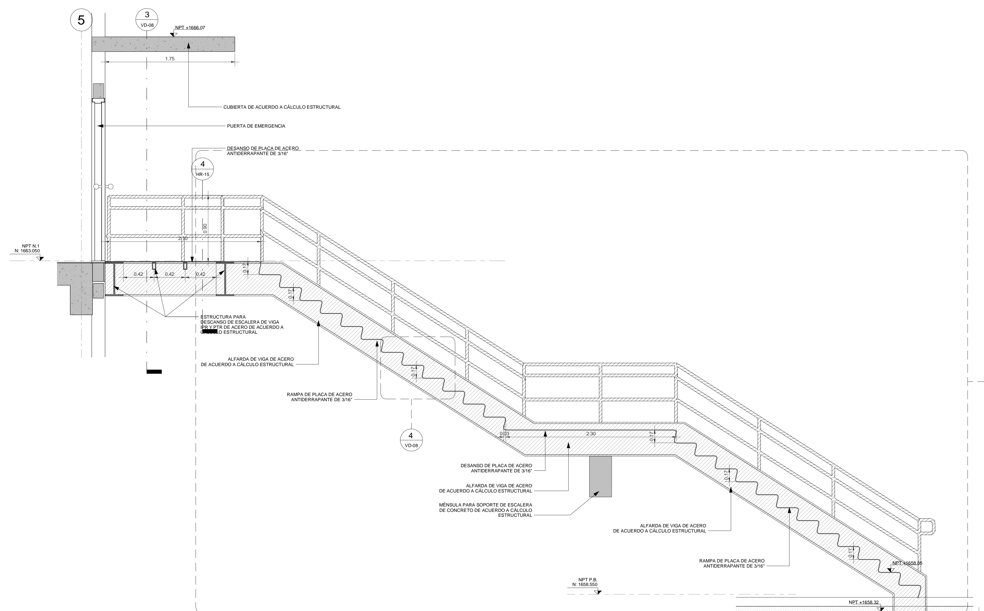
2 Sección a detalle escalera de emergencia -1 ESCALA 1 : 25
