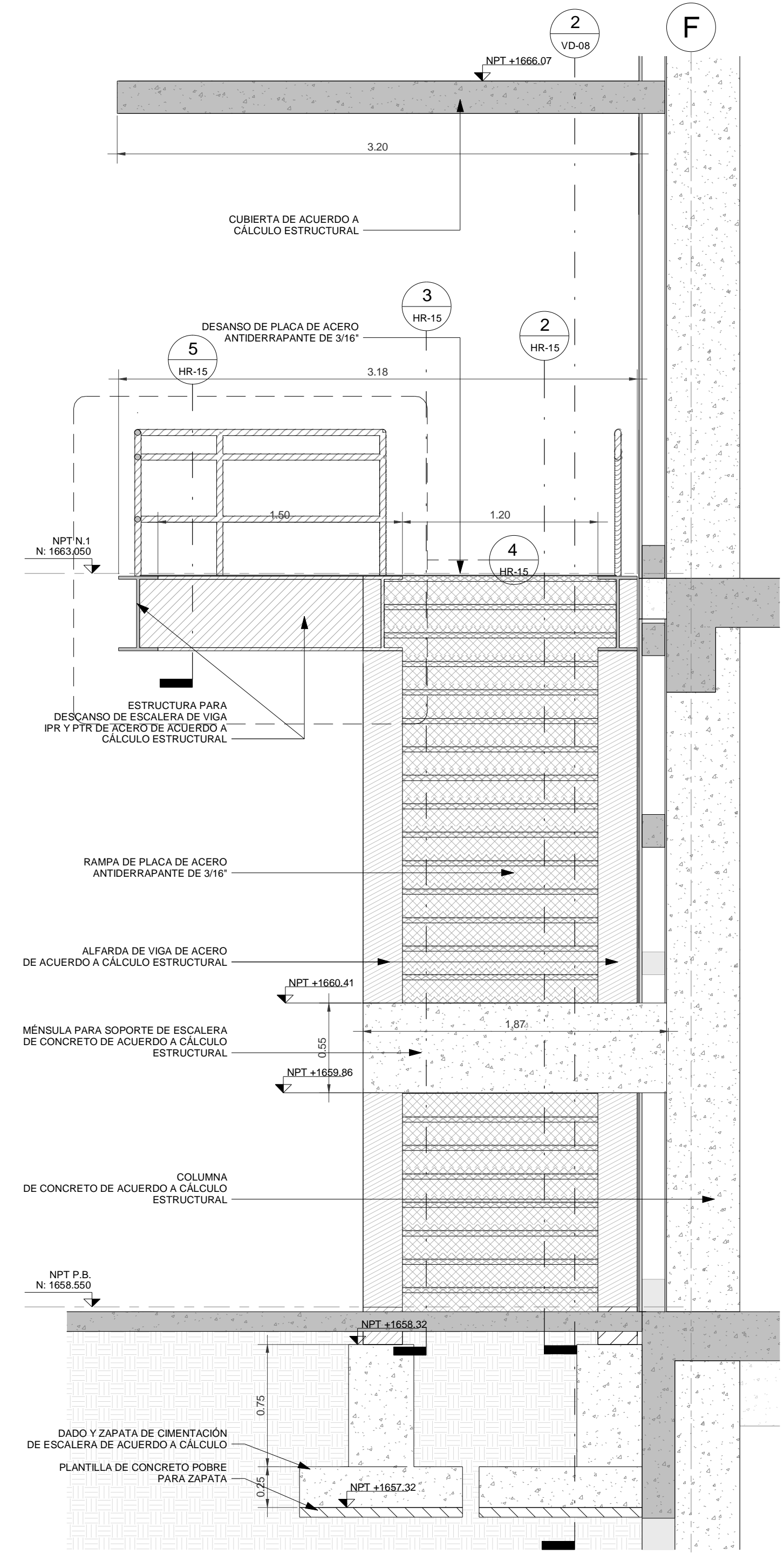
3 Sección a detalle escalera de emergencia -2 ESCALA 1 : 25
