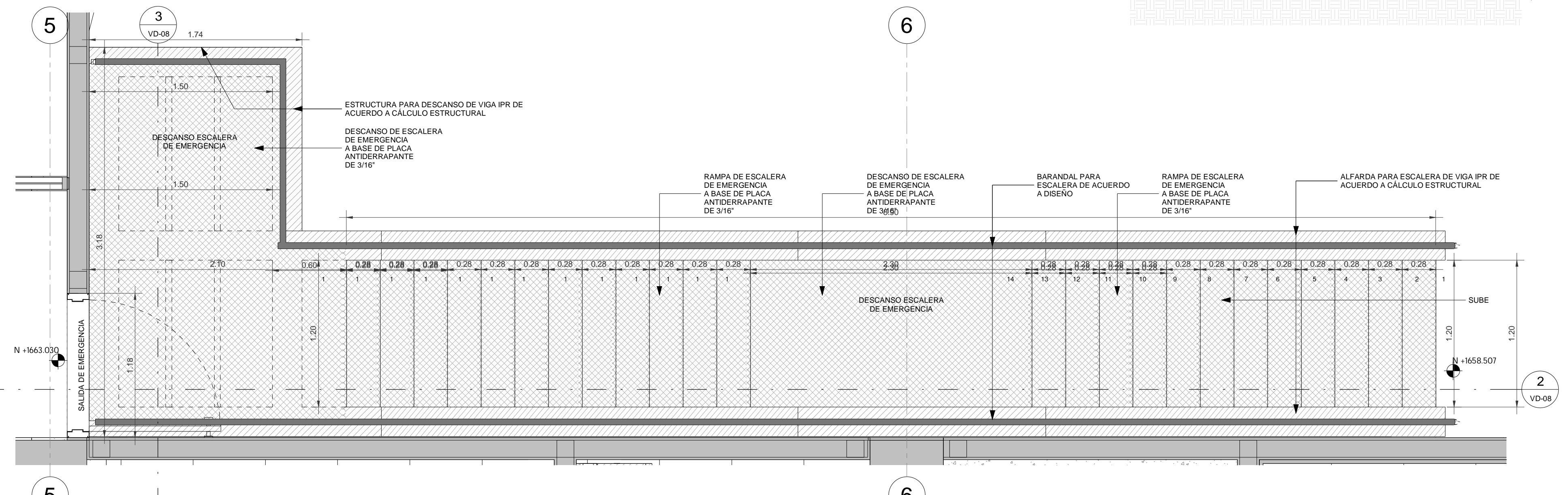
1 Vista a detalle escalera de emergencia ESCALA 1 : 25
