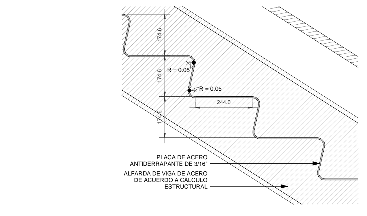
4 Detalle de escalones escalera de emergencia ESCALA 1 : 10
