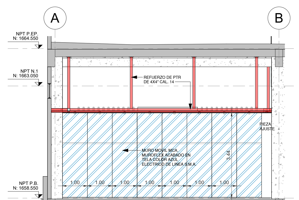
5 ALZADO-MURO MOVIL 3 ESCALA 1 : 75
