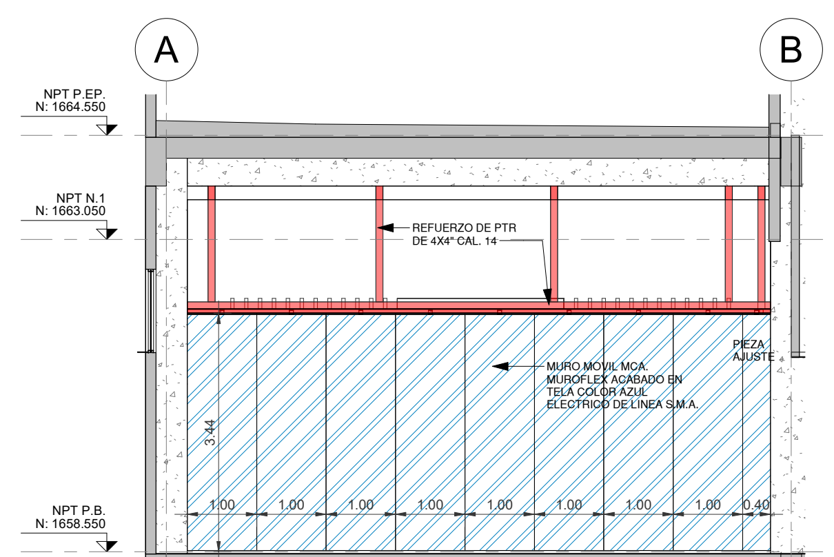
3 ALZADO-MURO MOVIL 1 ESCALA 1 : 75
