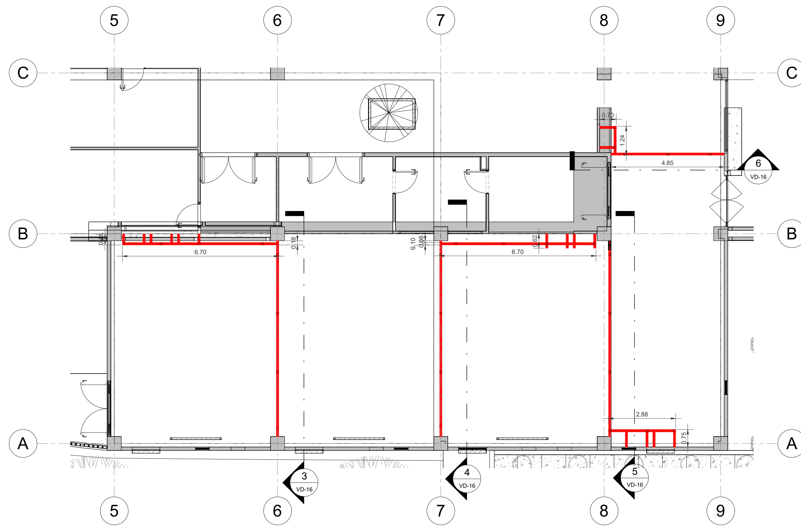
2 PLANTA-MUROS MOVILES REFEUERZOS ESCALA 1 : 100
