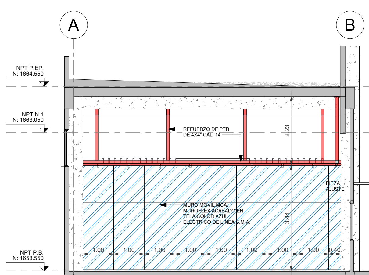
4 ALZADO-MURO MOVIL 2 ESCALA 1 : 75
