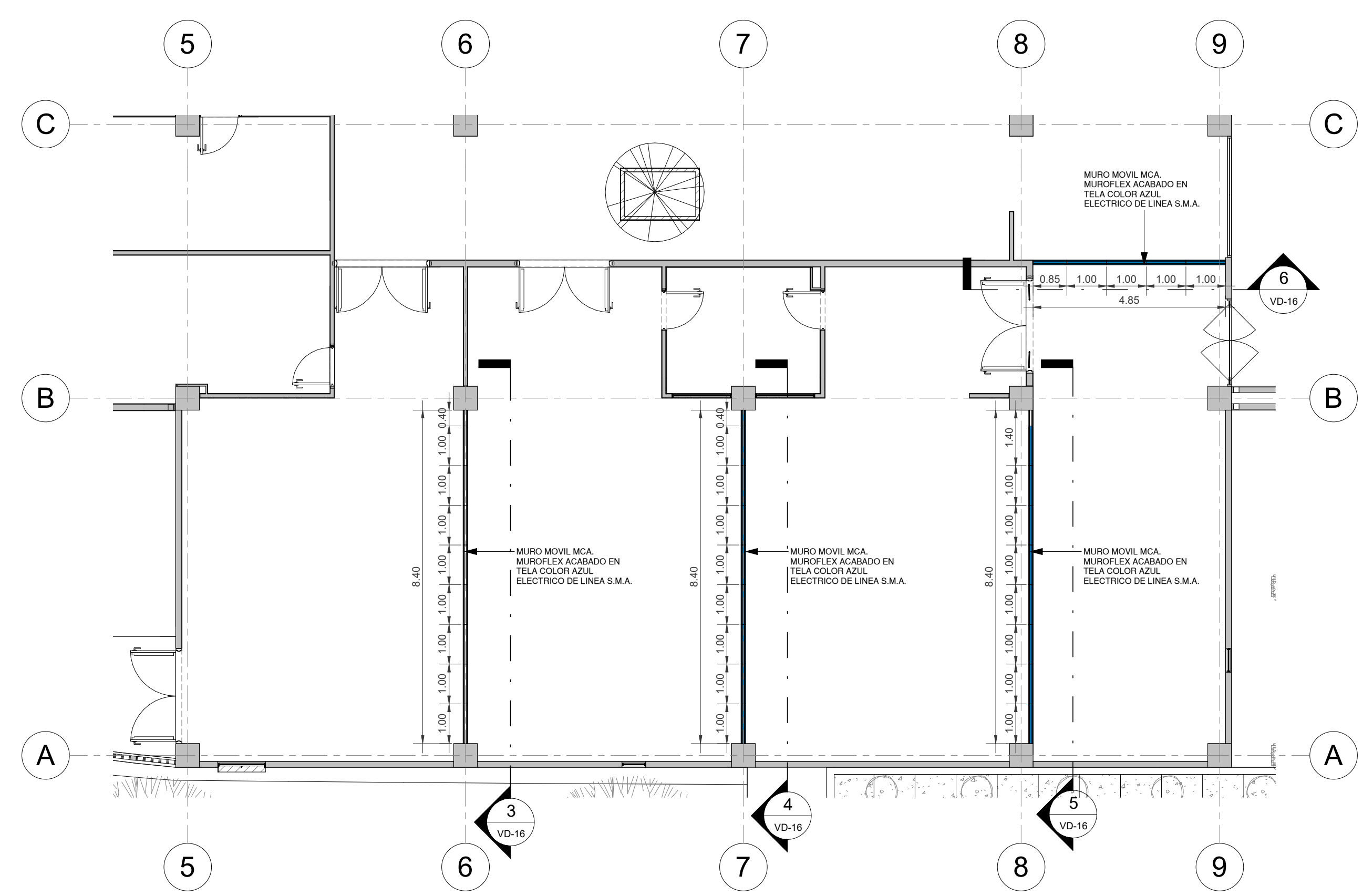
1 PLANTA-MUROS MOVILES ESCALA 1 : 100
