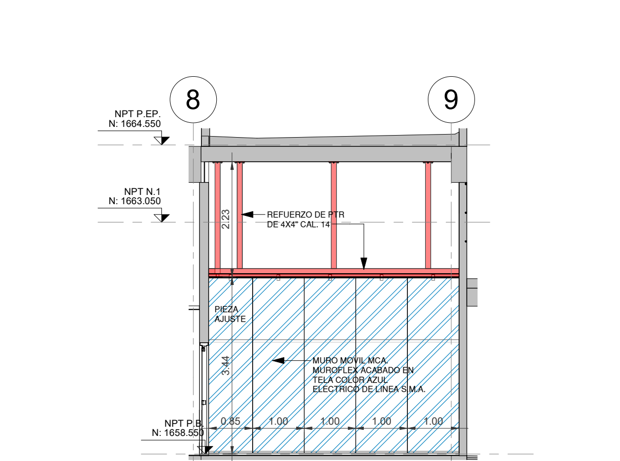
6 ALZADO-MURO MOVIL 4 ESCALA 1 : 75
