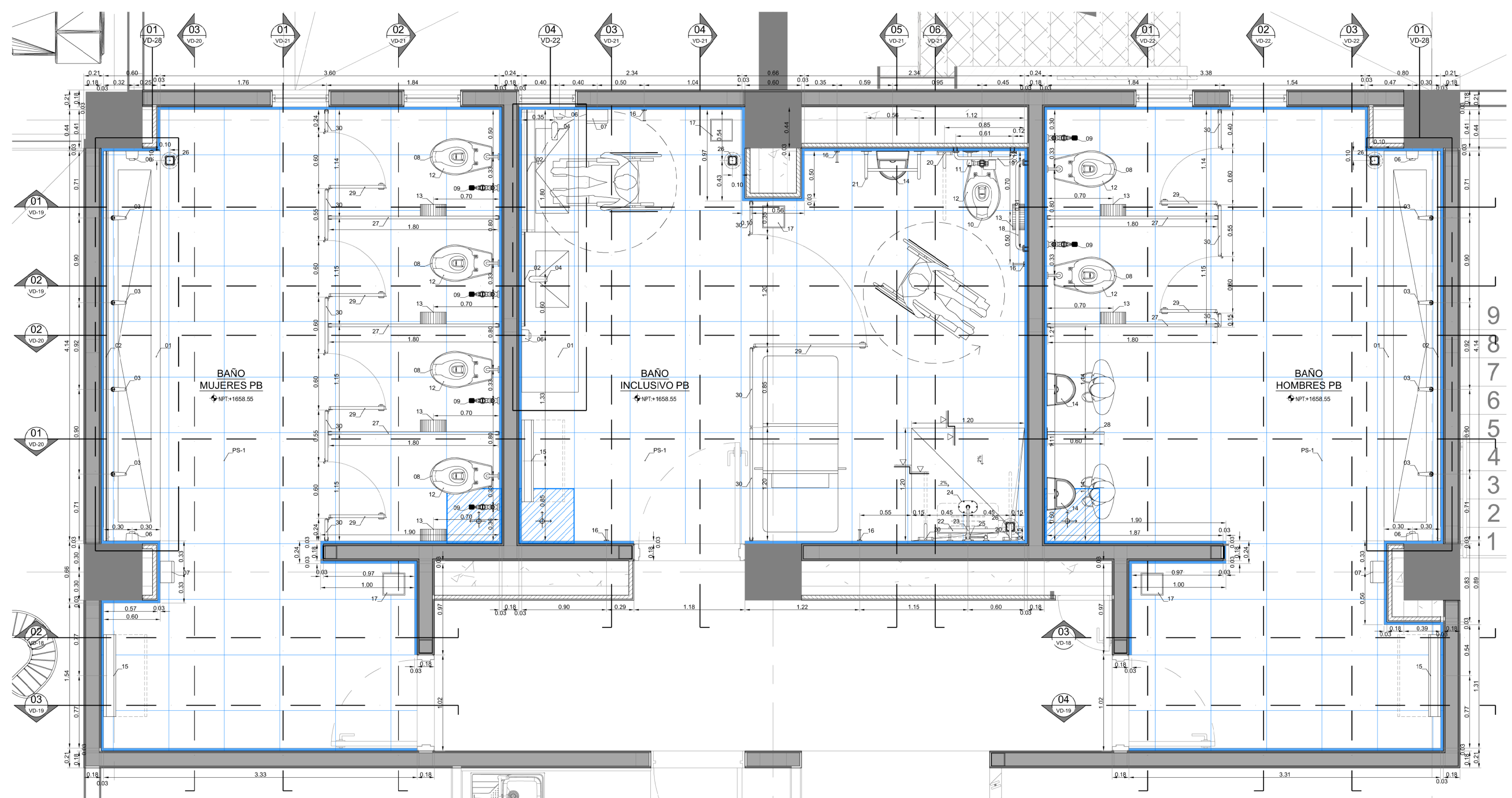
01 - VISTA A DETALLE - BAÑOS GENERALES PLANTA BAJA ESC: 1:25
