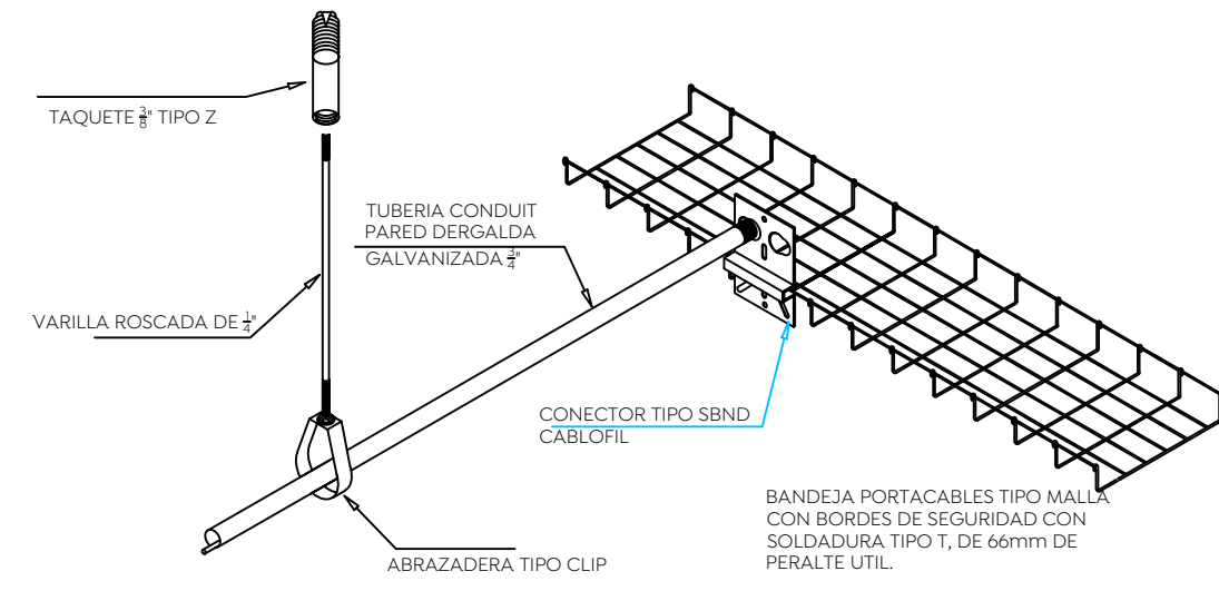
DETALLE FIJACIÓN DE TUBERIA
