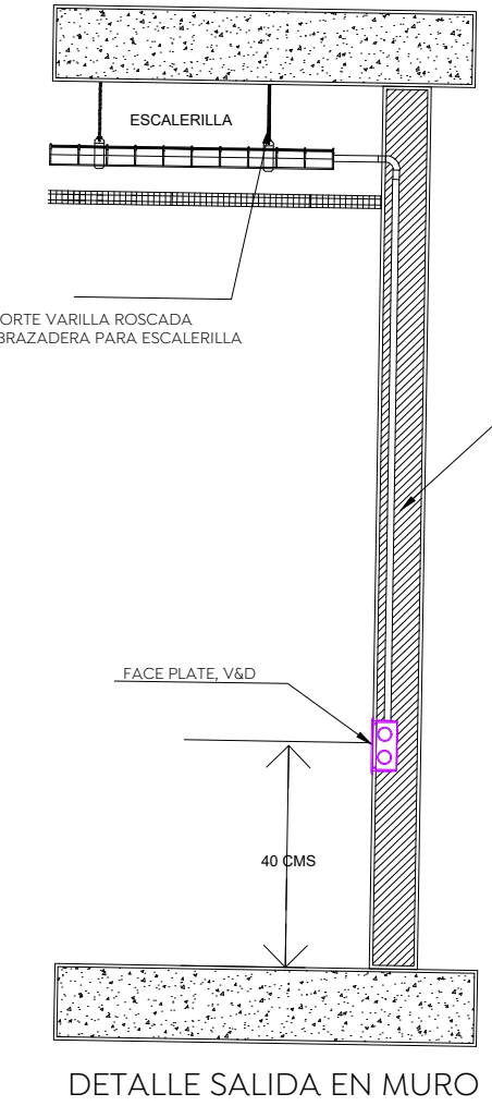
DETALLE SALIDA EN MURO
