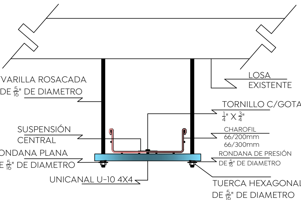
DETALLE FIJACIÓN DE CHAROLA
