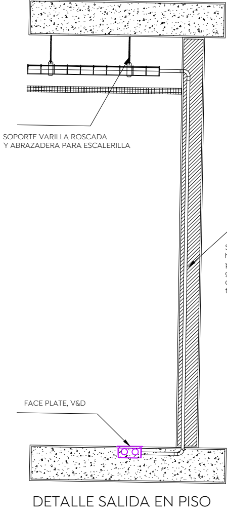
DETALLE SALIDA EN PISO
