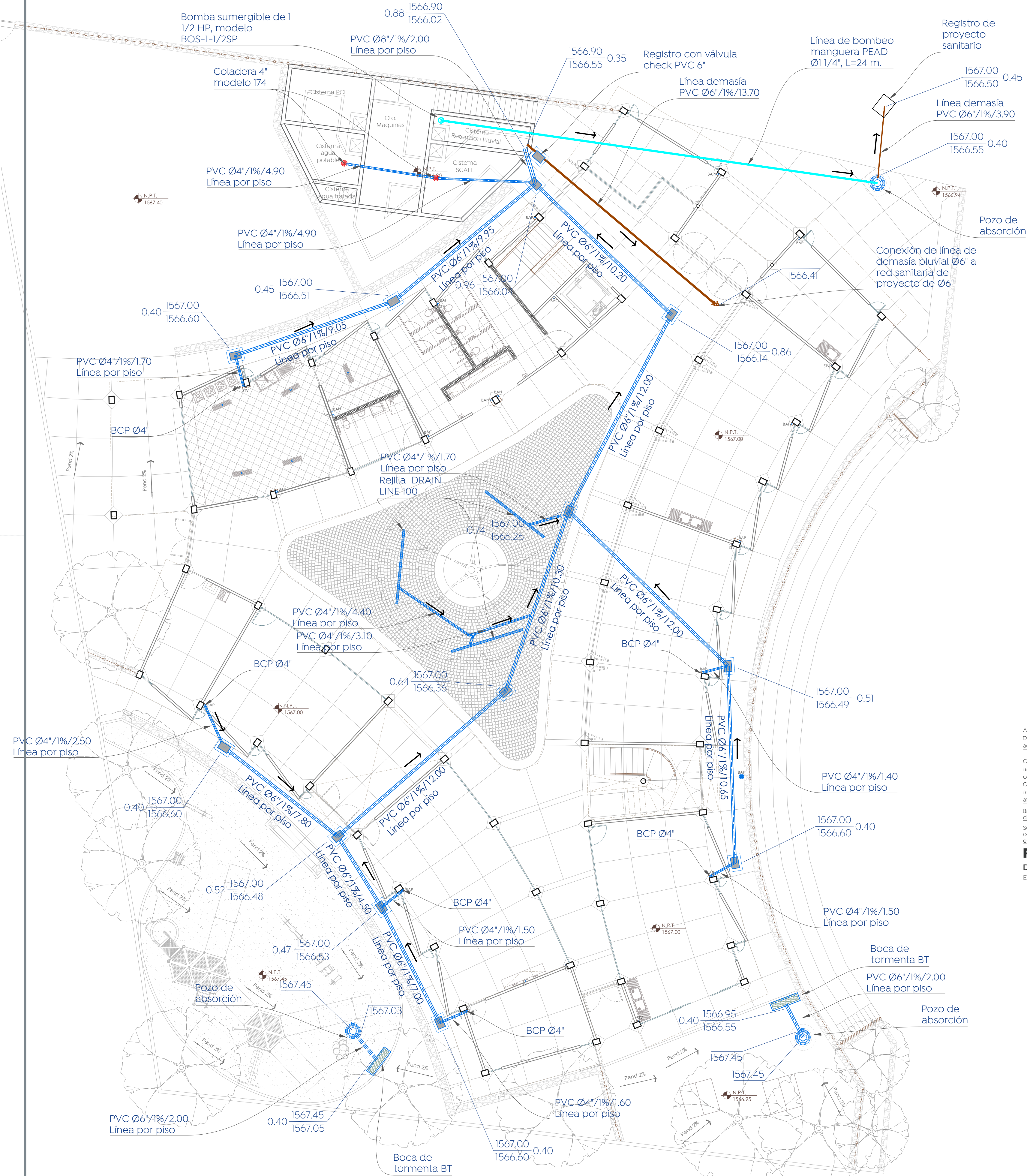
Planta baja Sistema pluvial Esc. 1:125
