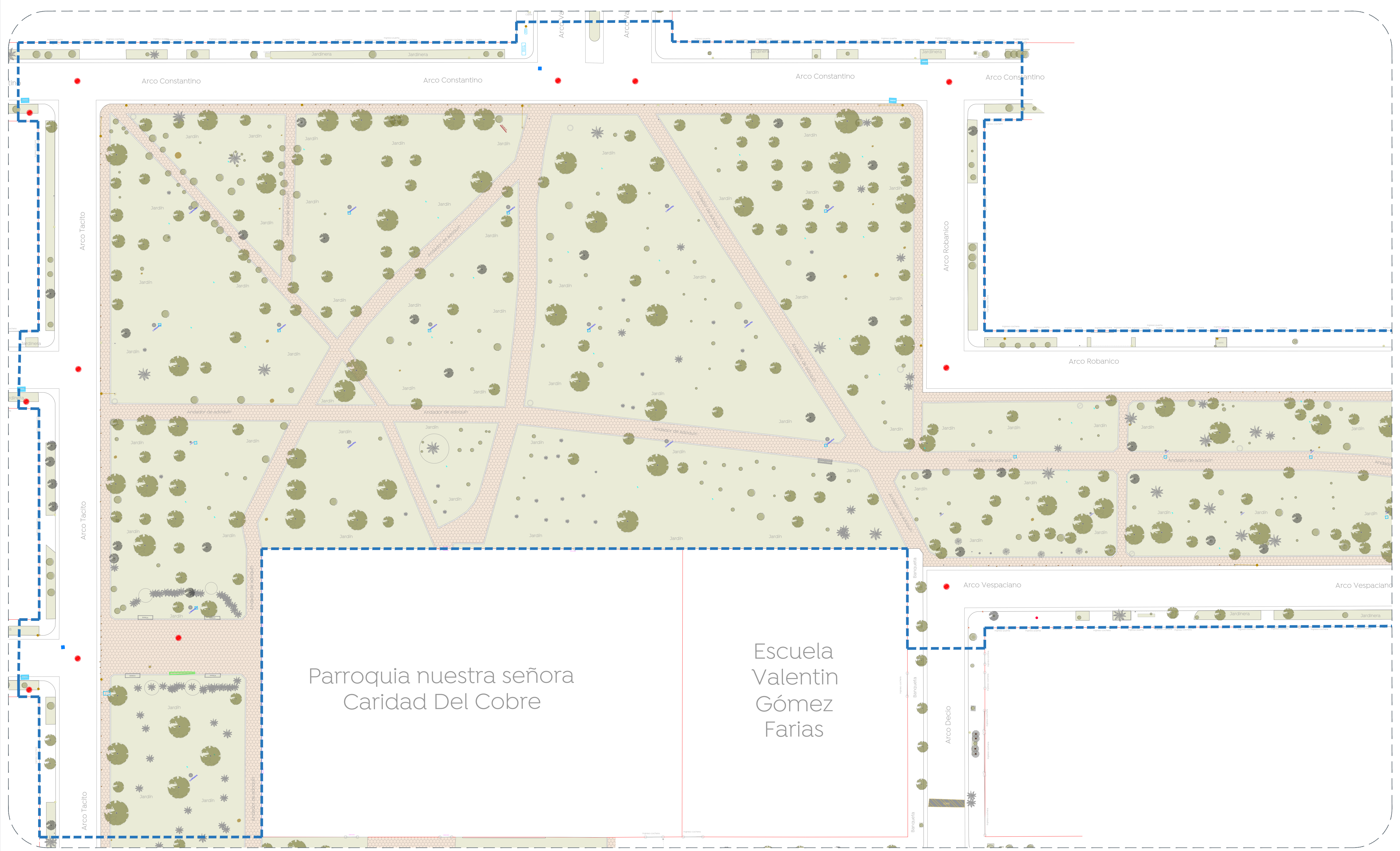
01 Planta tramo 2 Estado actual 1:300
