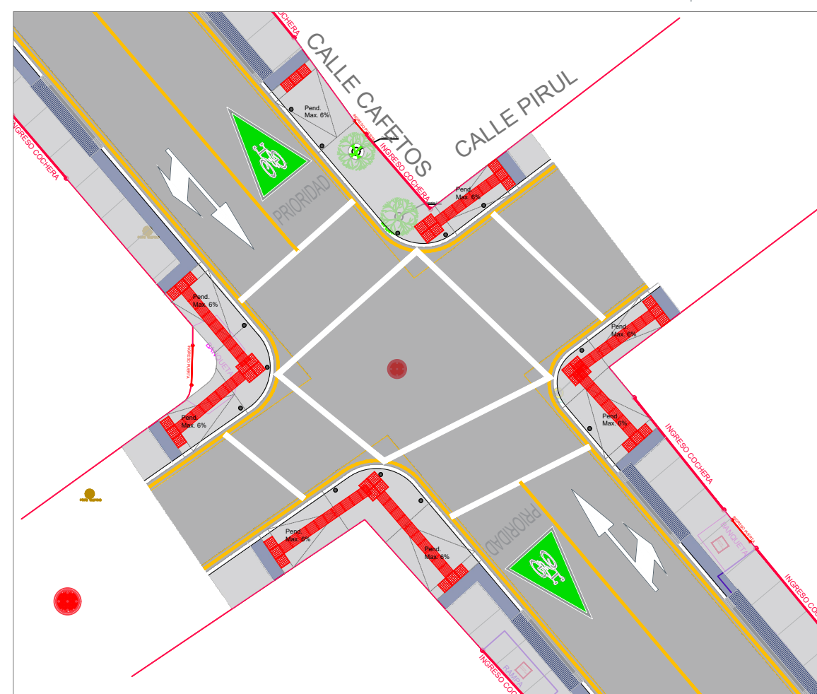
4 Calle Cafetos y Calle Pirul Escala 1:200
