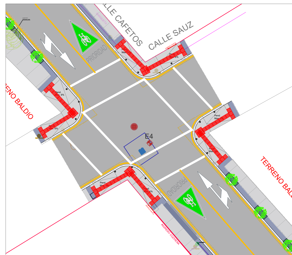
2 Calle Cafetos y Calle Sauz Escala 1:200
