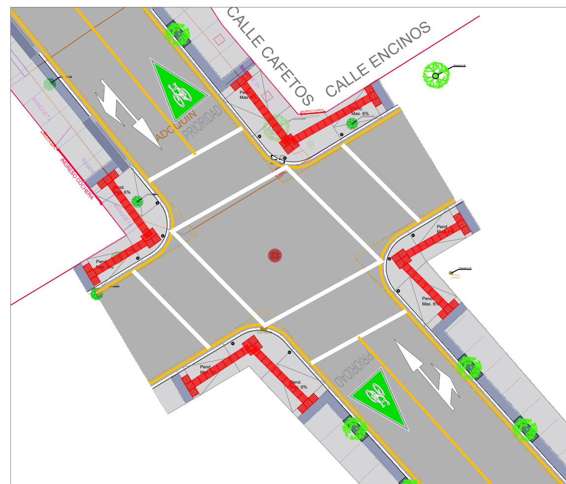
3 Calle Cafetos y Calle Encinos Escala 1:200
