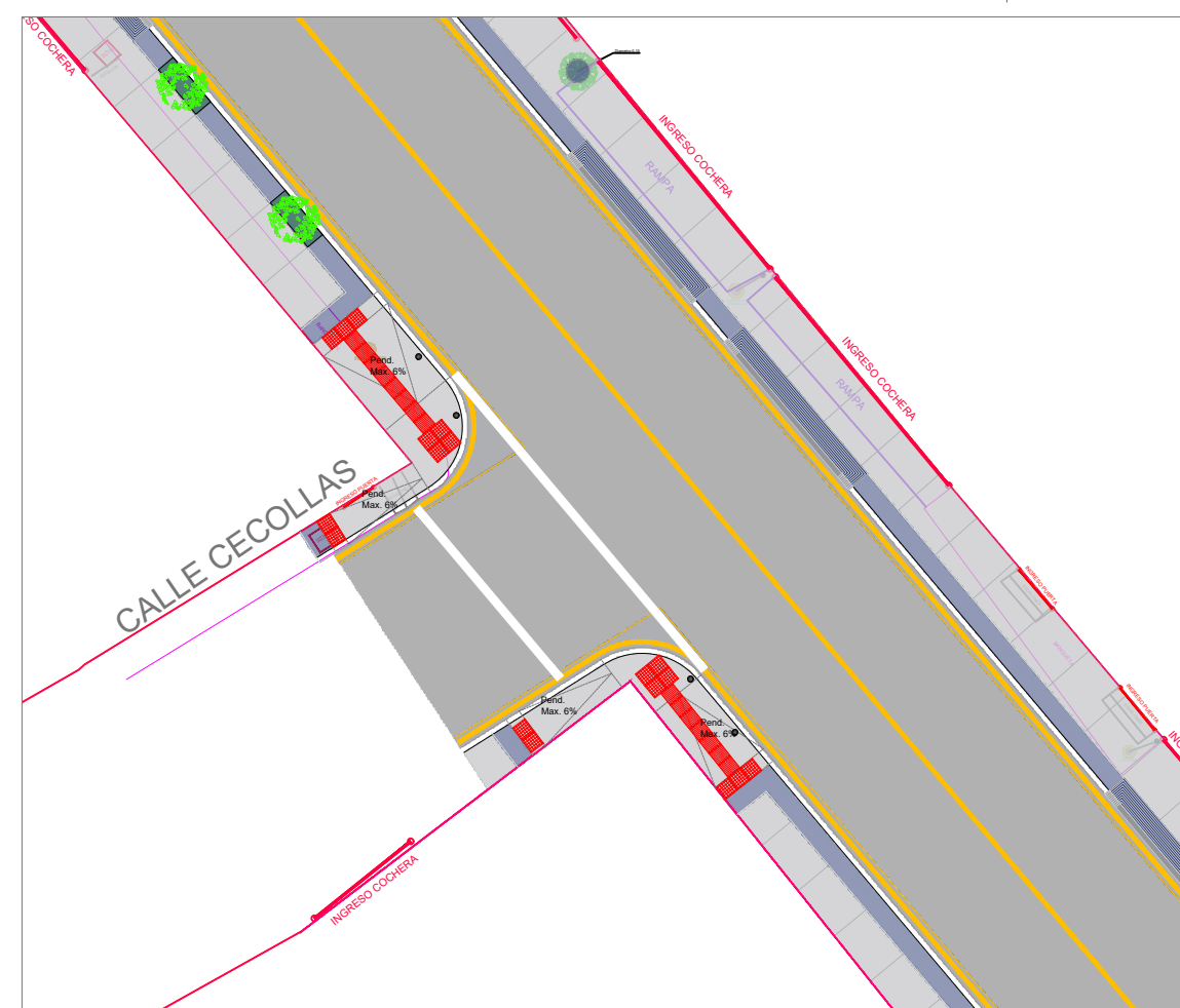
6 Calle Cafetos y Calle Cecollas Escala 1:200
