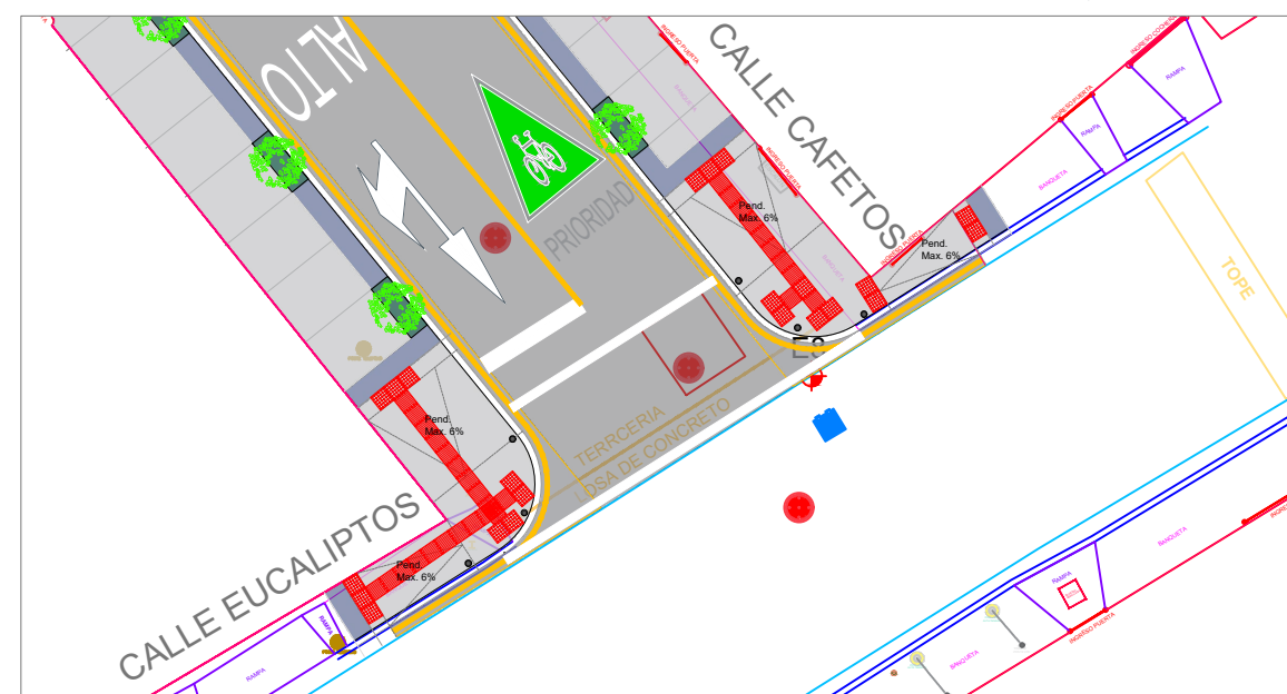
7 Calle Cafetos y Calle Eucaliptos Escala 1:200
