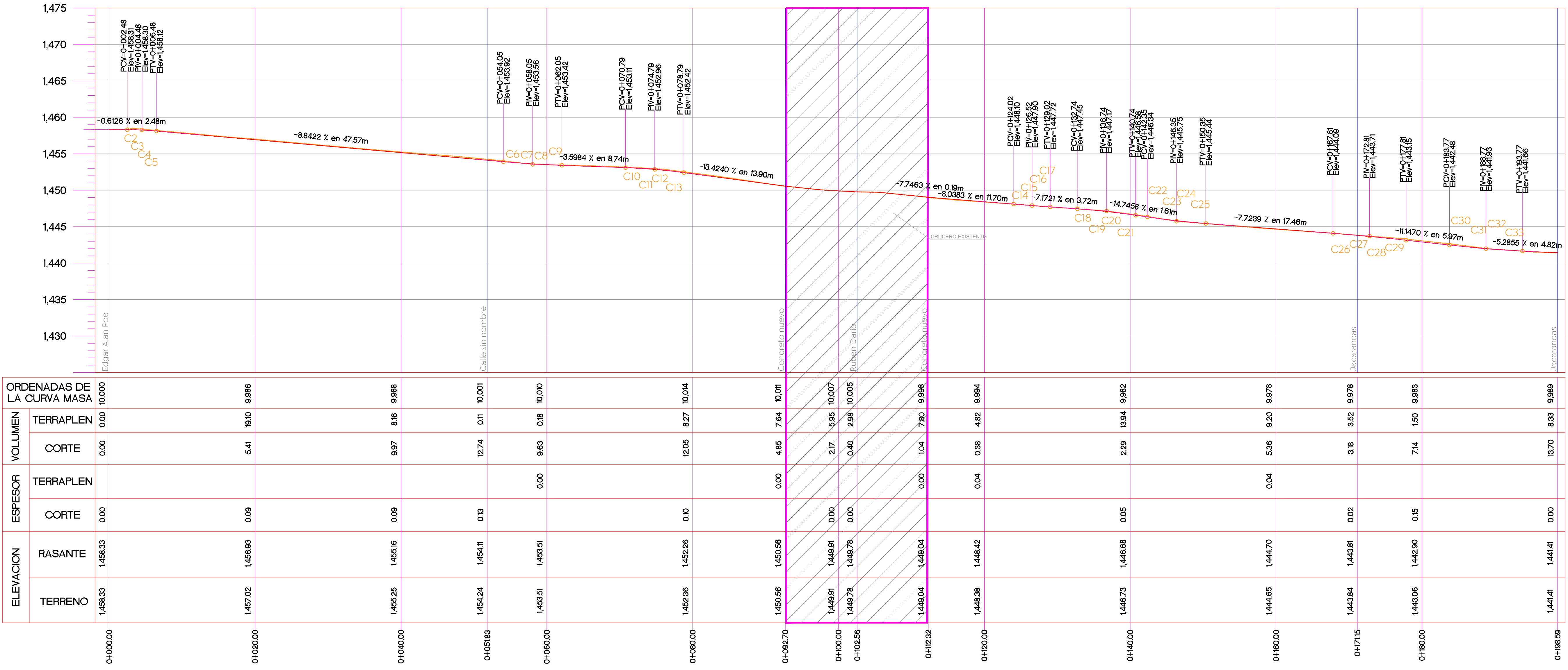
Perfil Calle Arturo Rivas Zainz De 0+000.00 a 0+198.59 Escala 1:300
