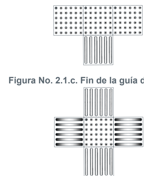
Figura No. 2.1.d. Cambios de dirección.
