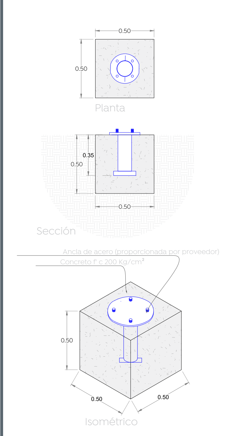
02 Detalle de ancla MOBILIARIO 1:20
