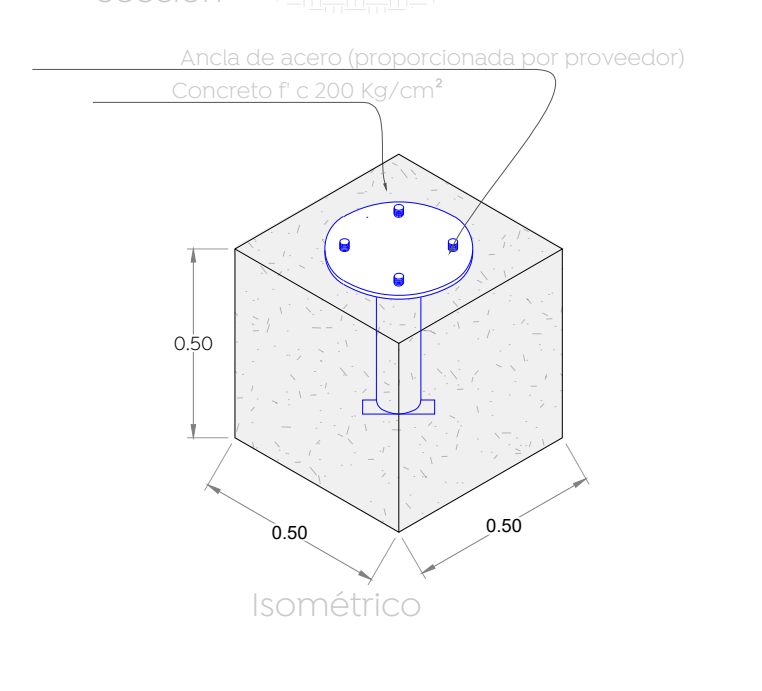
02 Detalle de ancla MOBILIARIO 1:20
