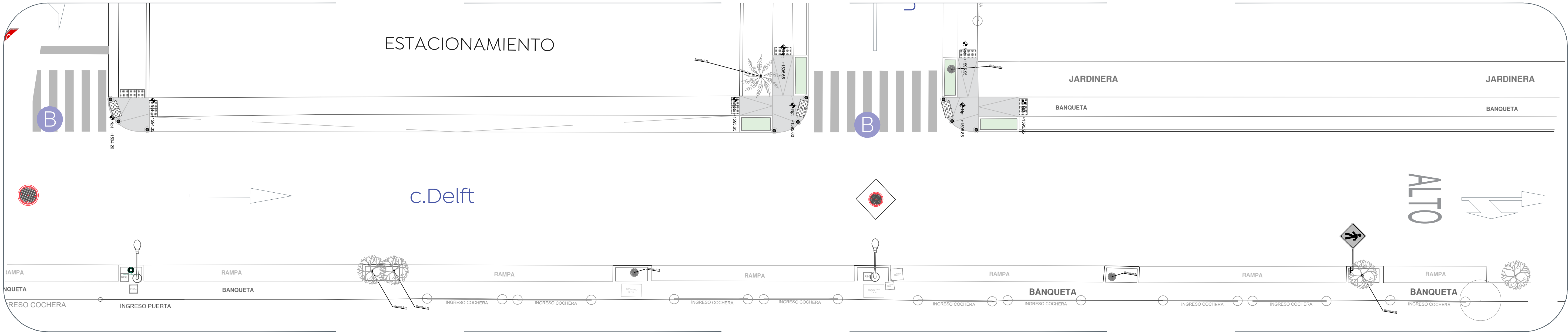
01 Planta de Conjunto - Tramo 2 Alcances 1:100
