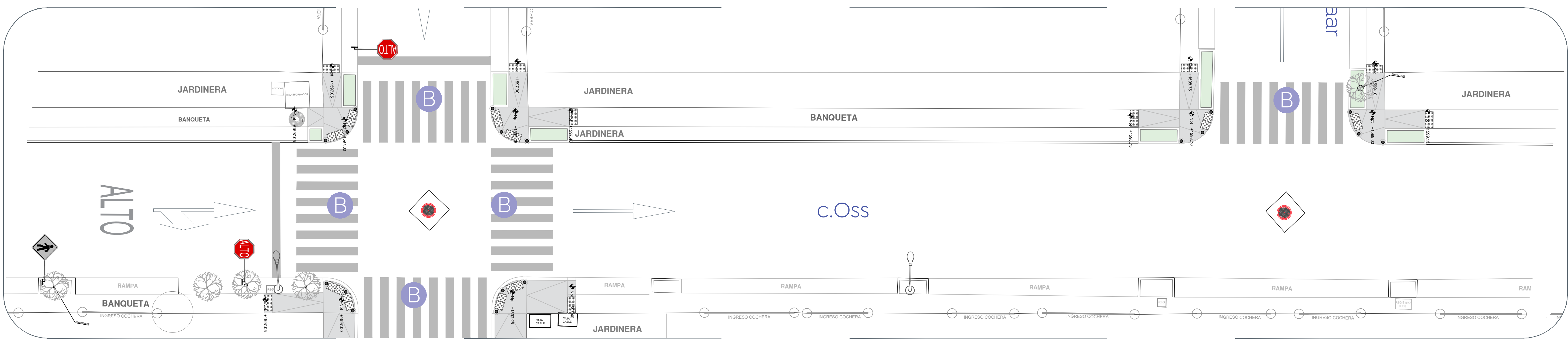
02 Planta de Conjunto - Tramo 3 Alcances 1:100
