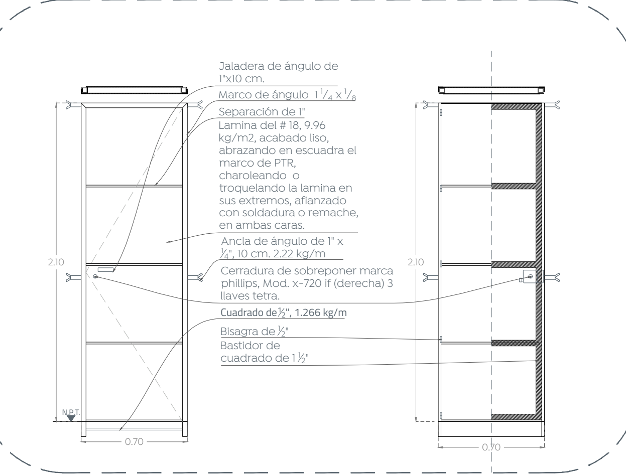
04 PH-2 Detalle de herrerías 1:25
