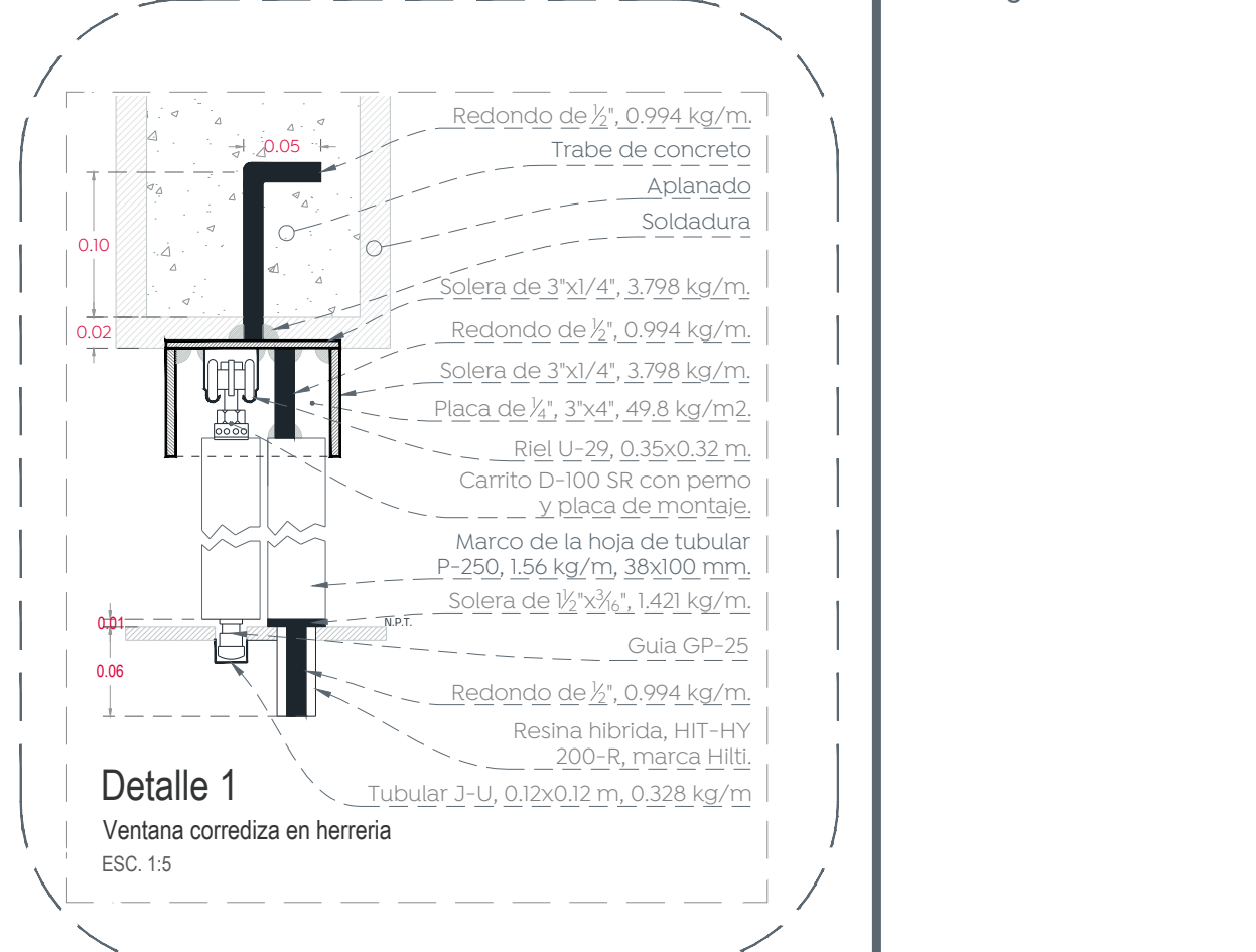
08 Detalle 1 Ventana corredera en herrería ESC. 1:5
