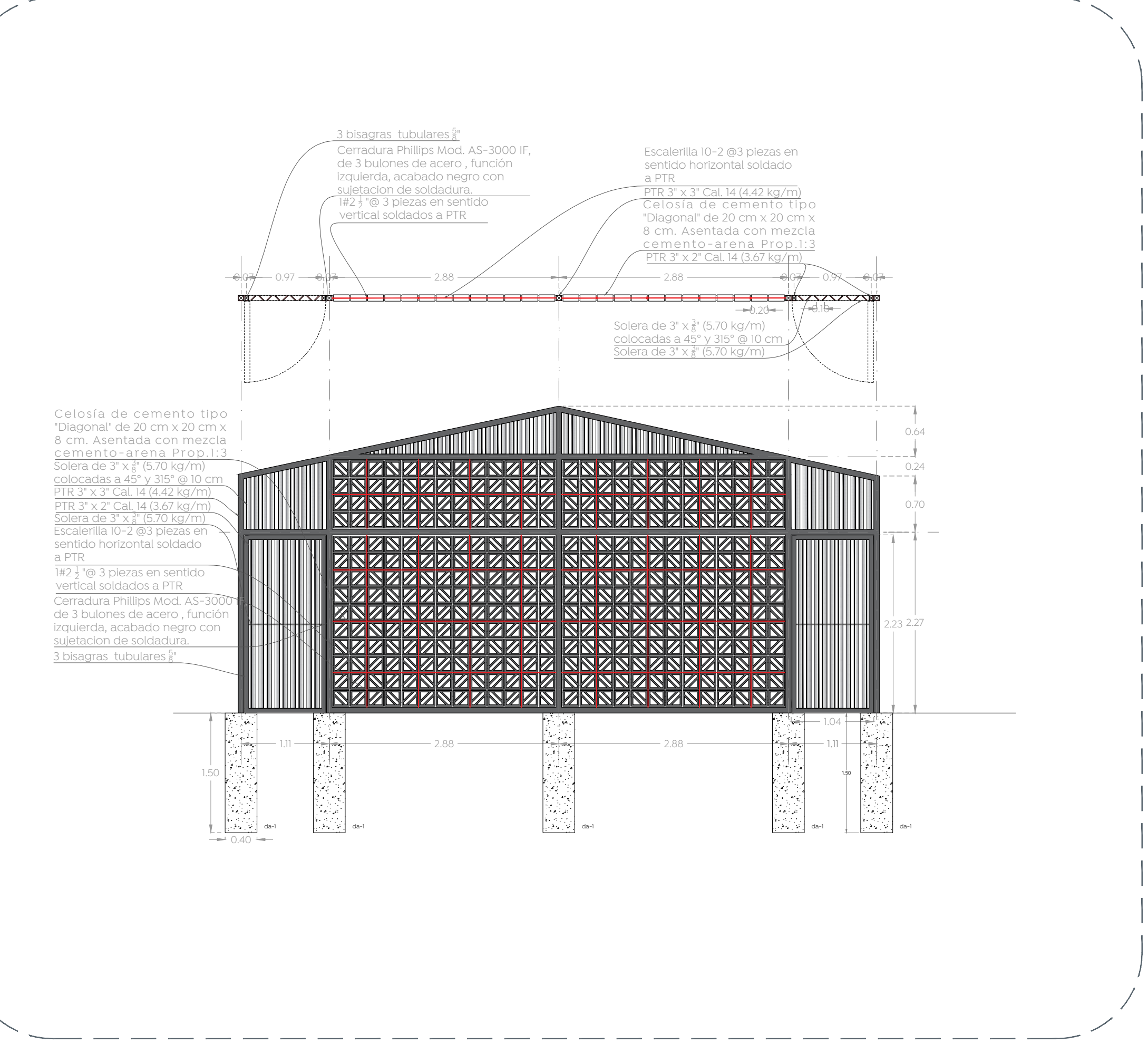
09 CH-1 Detalles de herrerías 1:50
