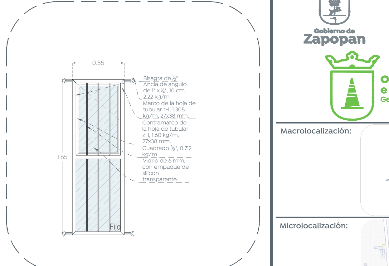
07 VH-3 Detalle de herrerías 1:25
