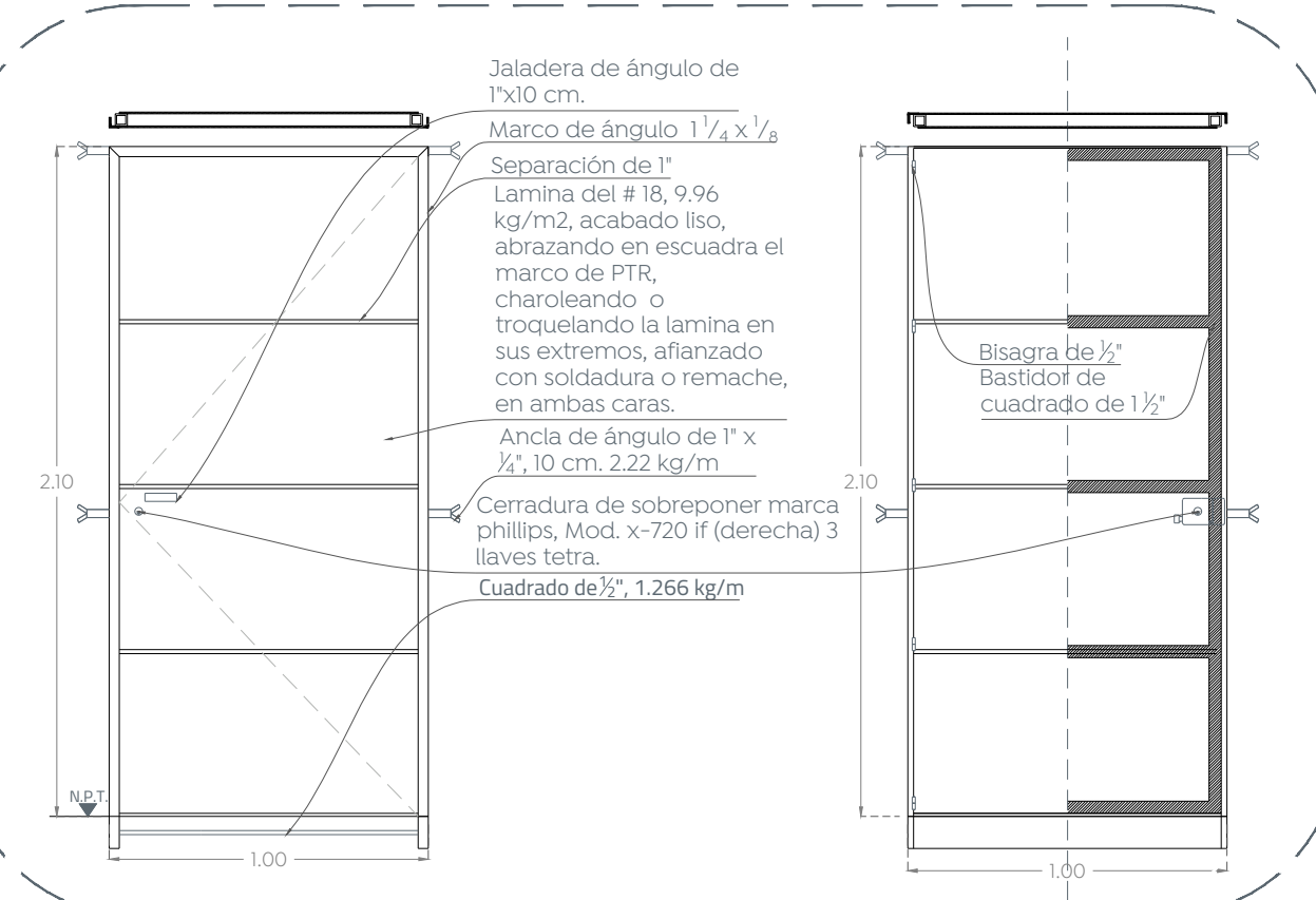
03 PH-1 Detalle de herrerías 1:25
