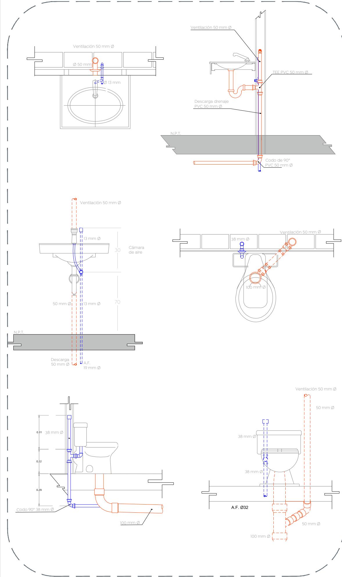
01 Instalación hidrosanitaria Planta de baños 1:20
