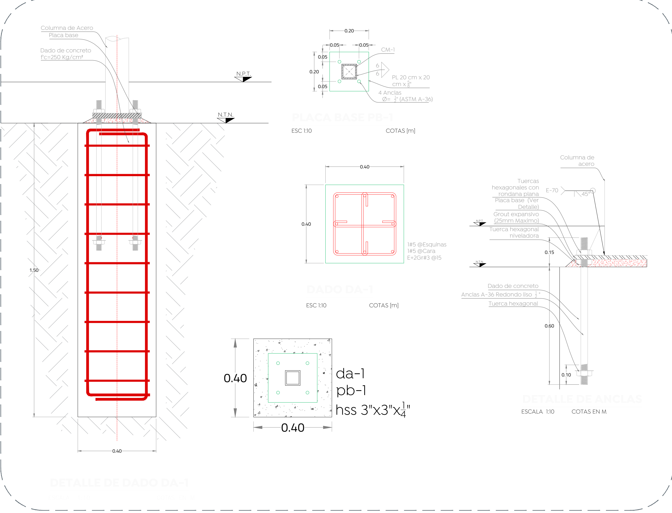
DETALLE DE DADO DA-1 1:50
