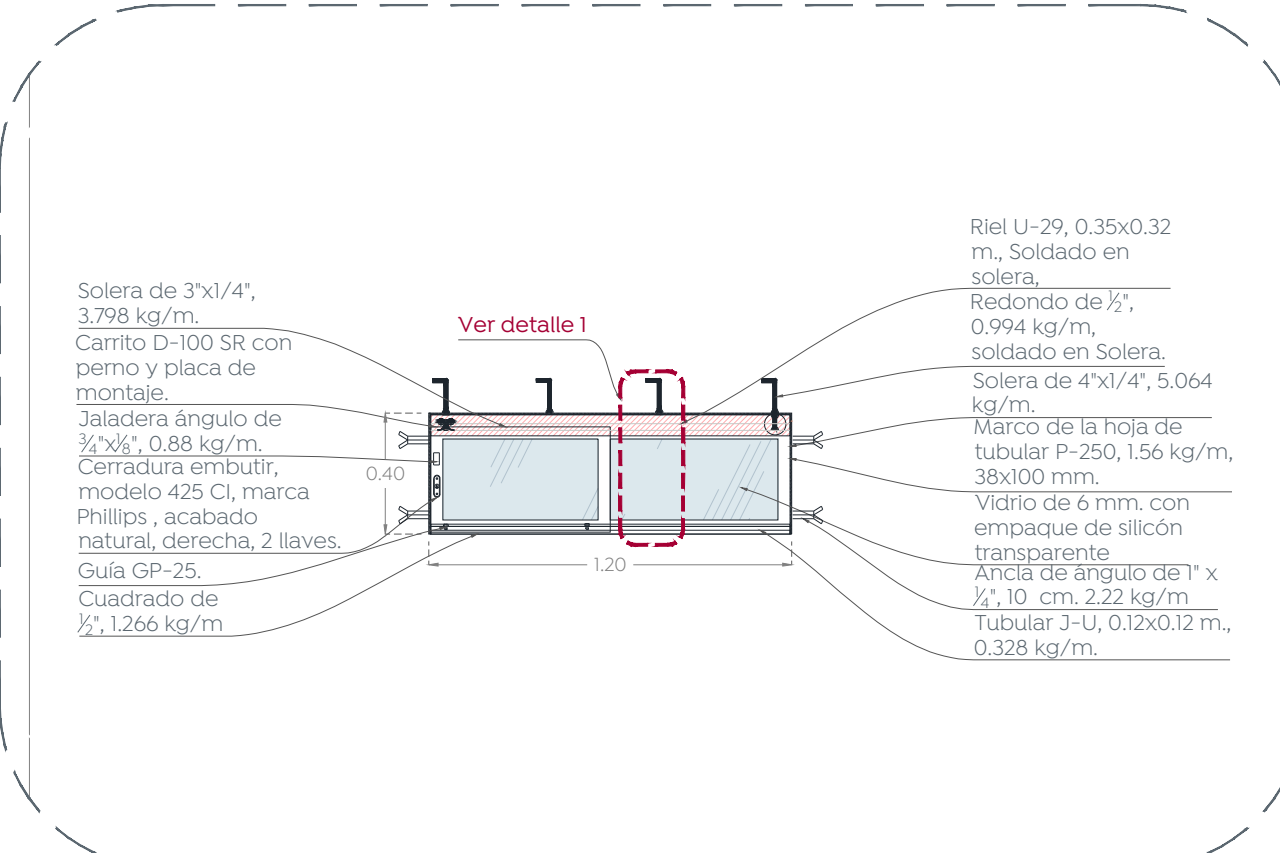
05 VH-1 Detalle de herrerías 1:25
