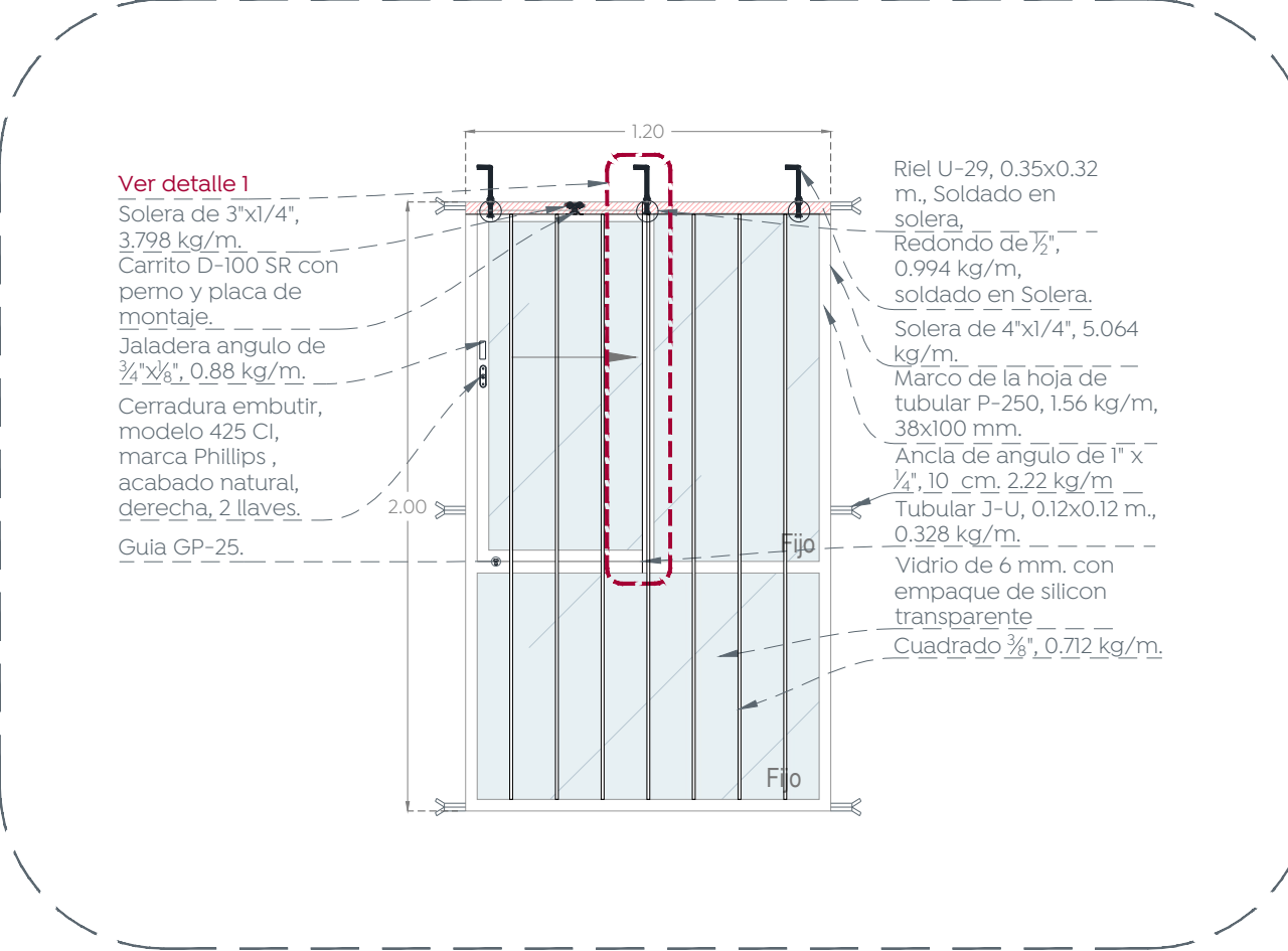
06 VH-2 Detalle de herrerías 1:25
