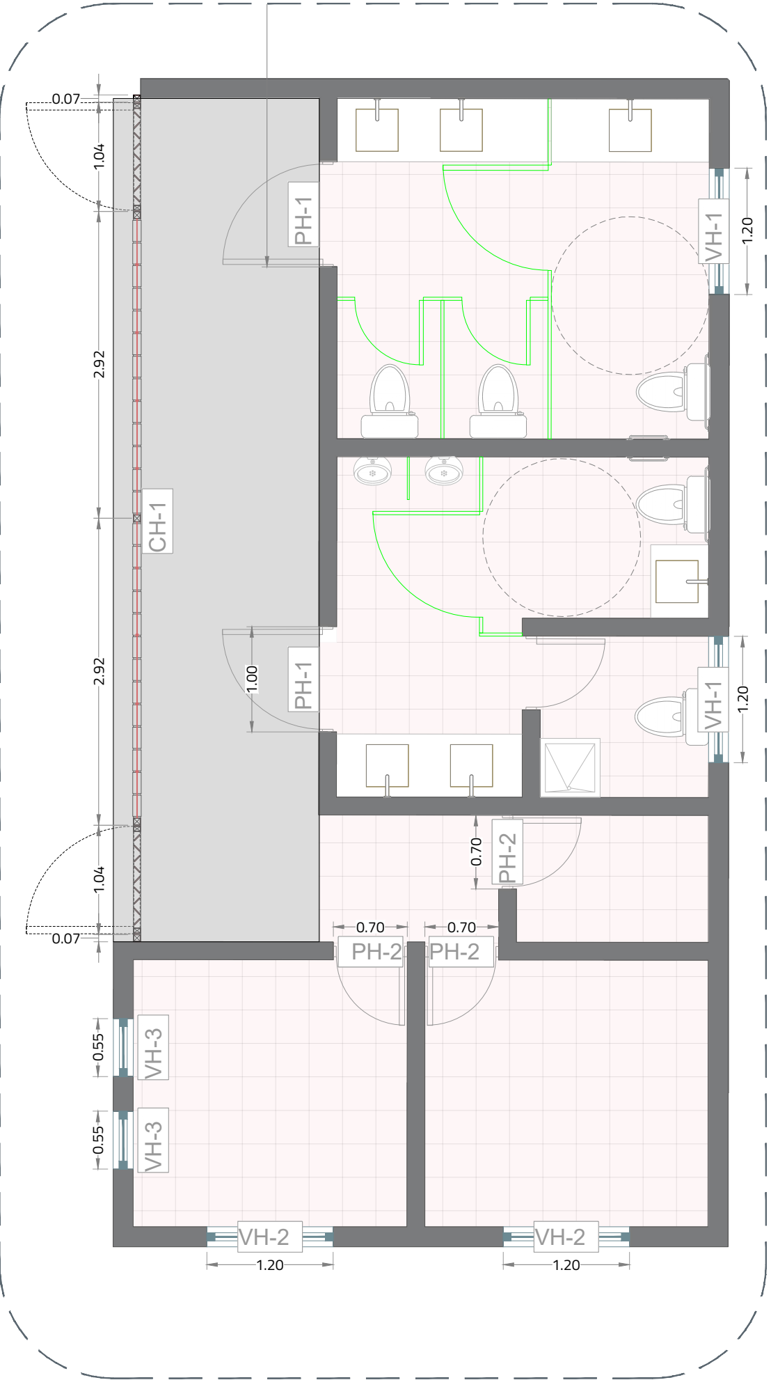
02 Herrerías Planta de baños 1:50
