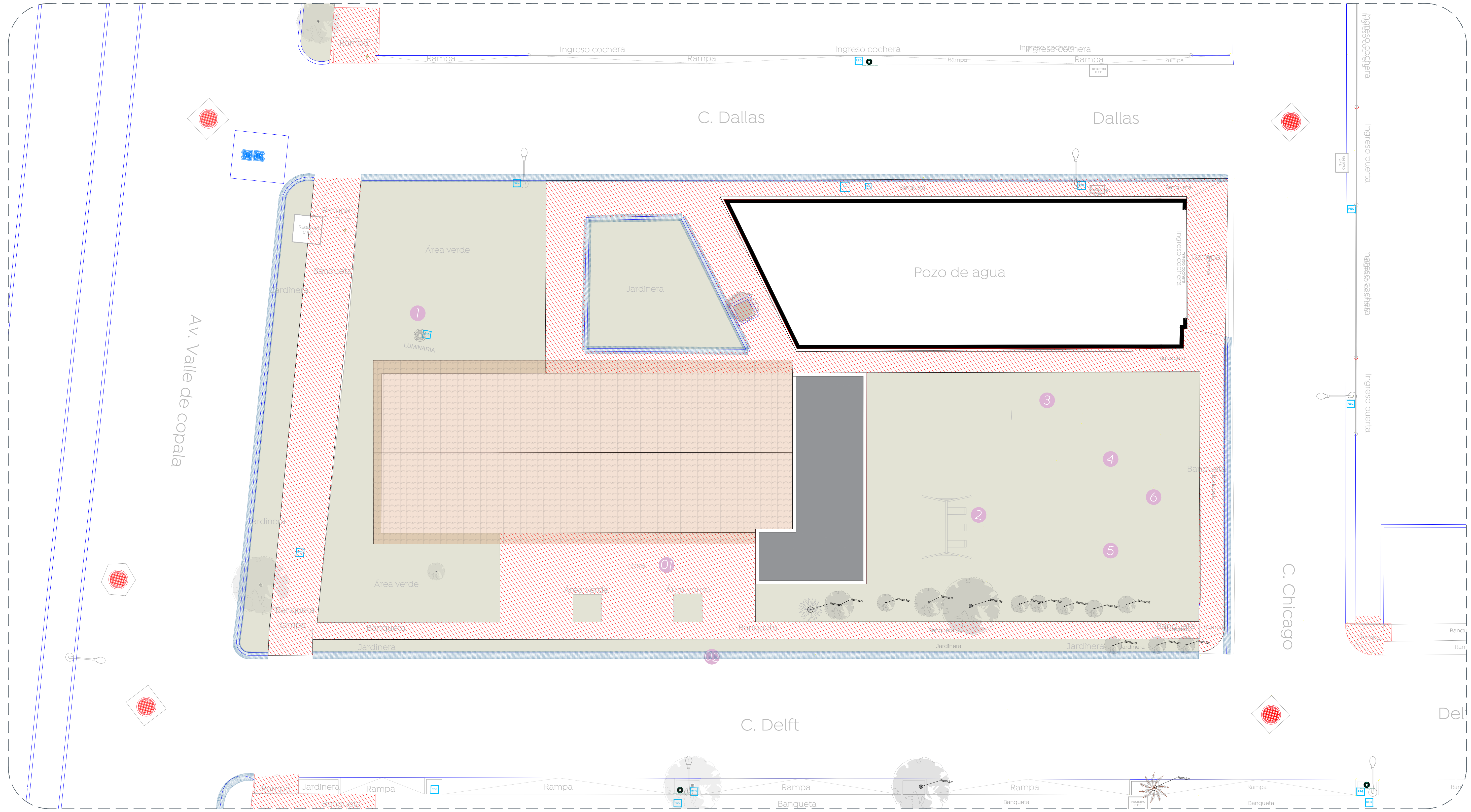
01 Planta de Conjunto - Tramo I Estado Actual - Demoliciones y retiros 1:100
