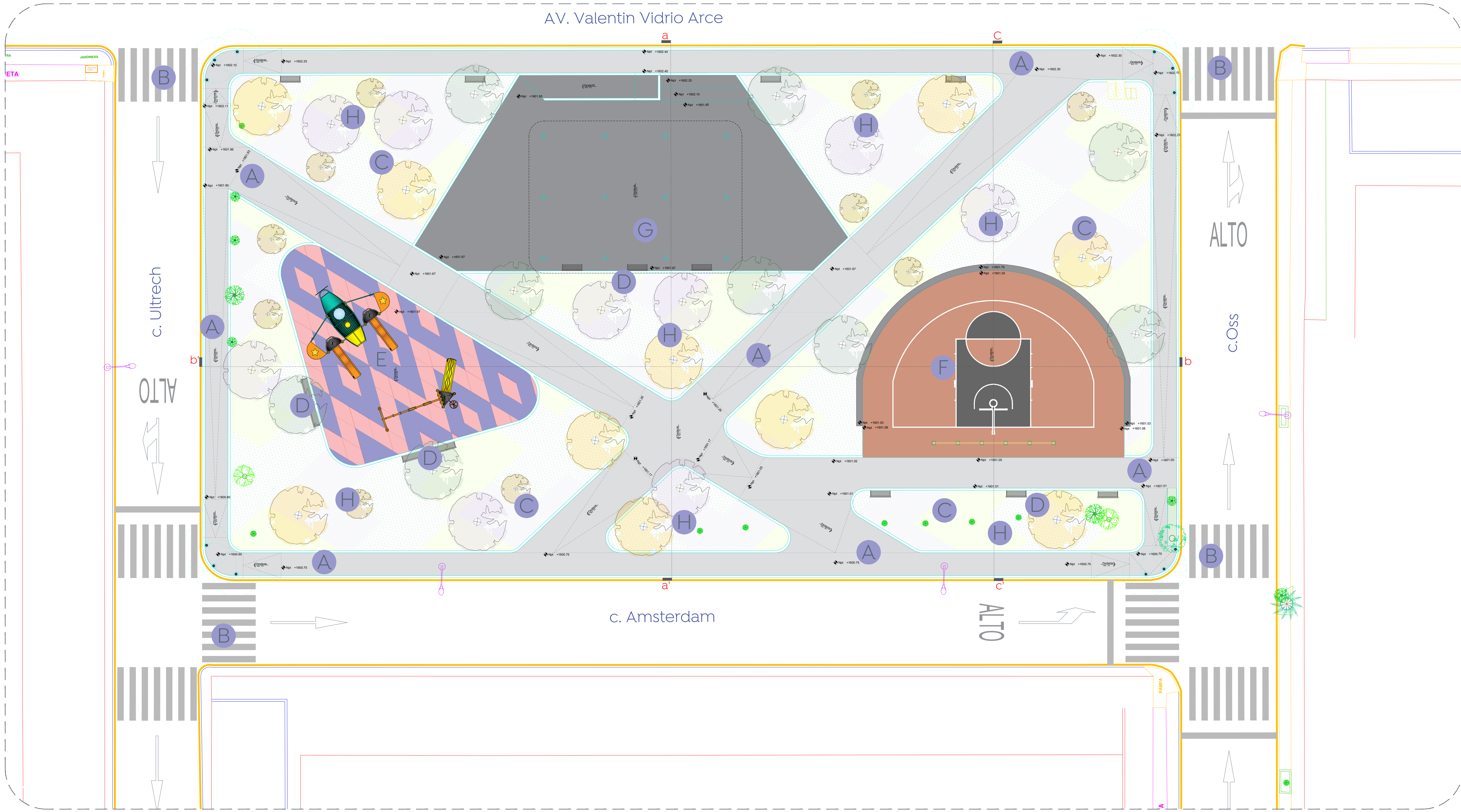
01 Planta de conjunto Alcances generales 1:125
