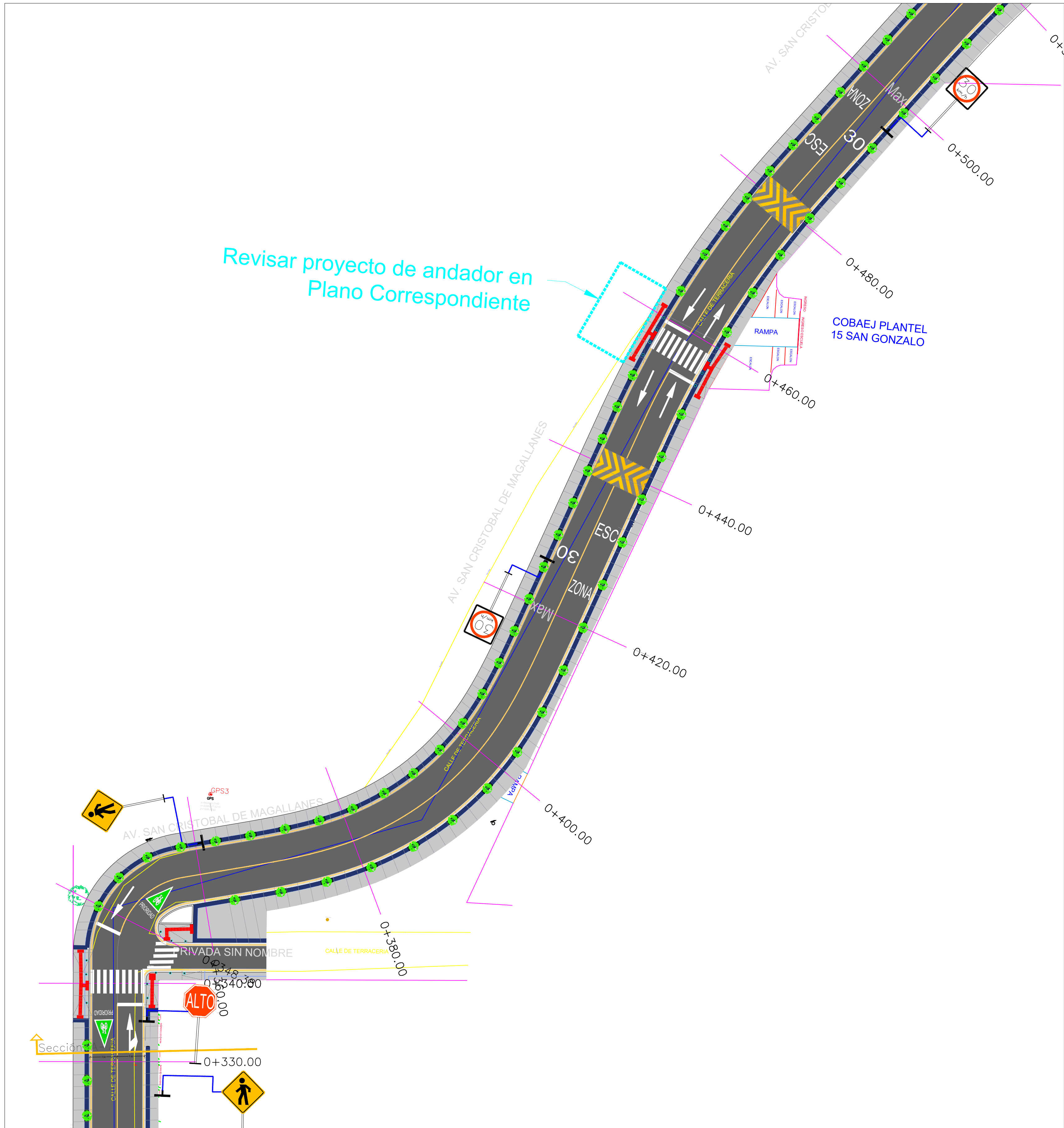
1 0+330.00 a 0+500.00 Escala 1:300
