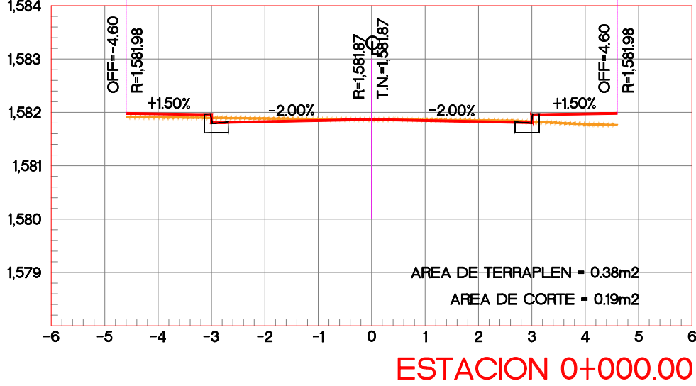
Secciones Escala 1:100
