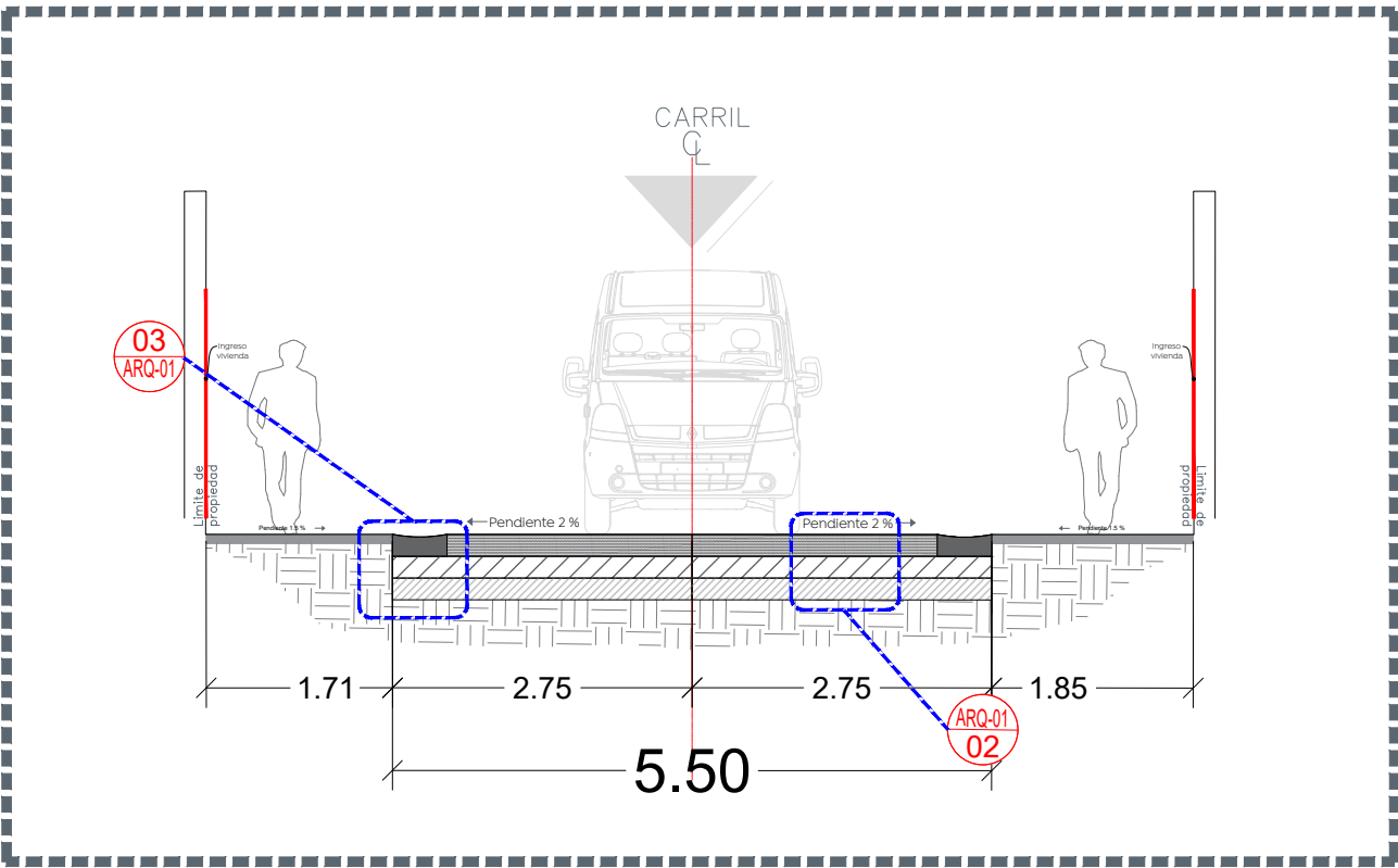
1 Sección A-A' Escala 1:75
