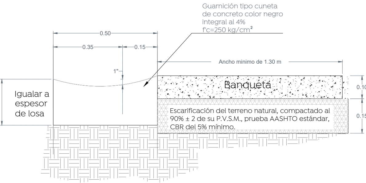
3 Detalle de guarnición Escala 1:10
