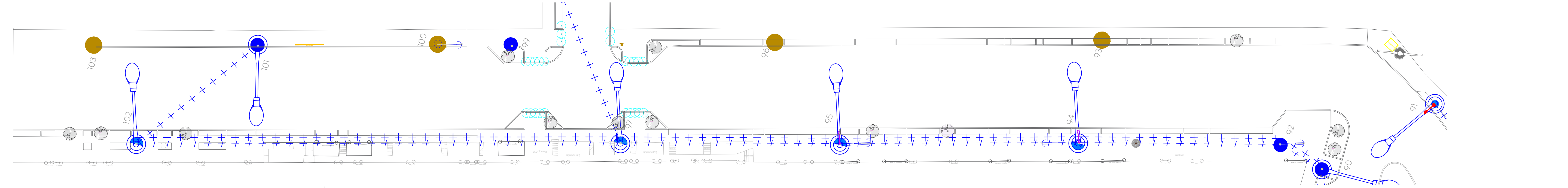
01 Levantamiento eléctrico Calle Santa Laura LEV-01 Escala 1:300
