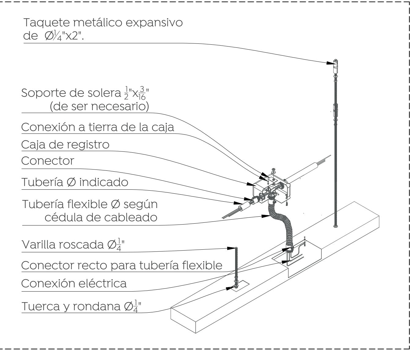
04 Conexión tipo lampara lineal. IE-01 S/E
