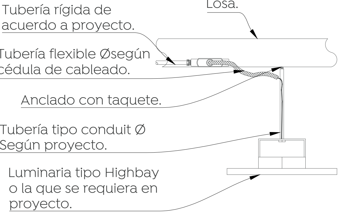
02 Fijación de luminaria suspendida. IE-01 S/E
