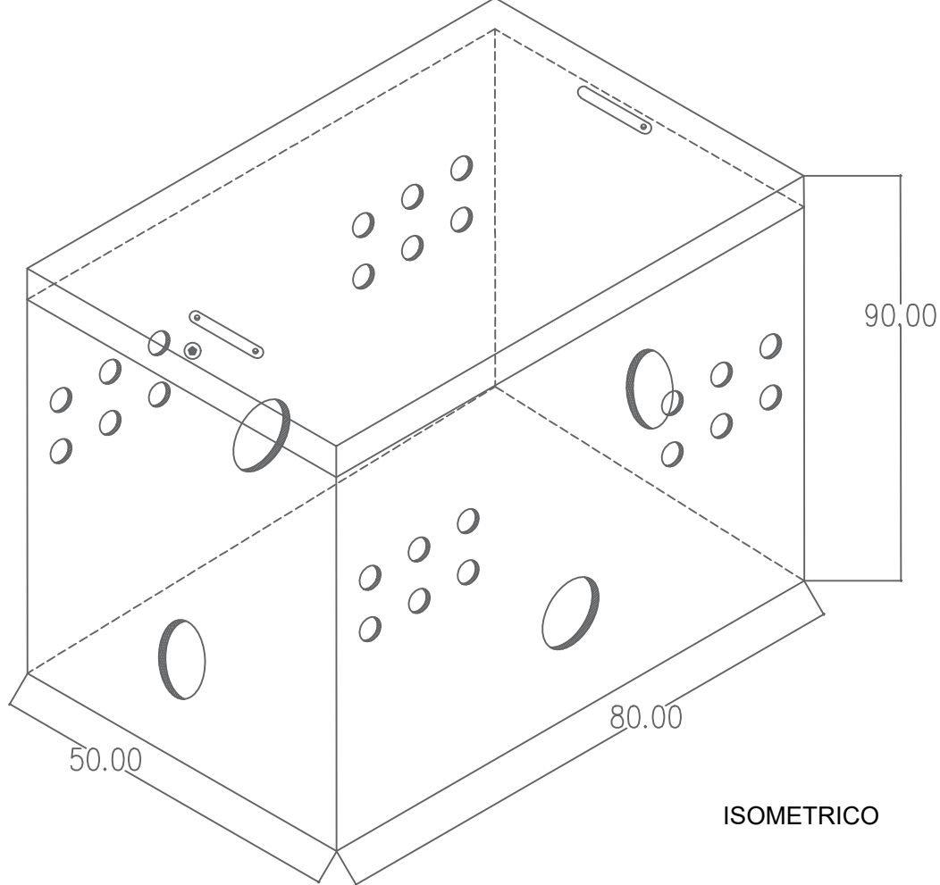
04 Detalle registro tipo 2 para BT IE-11 S/E
