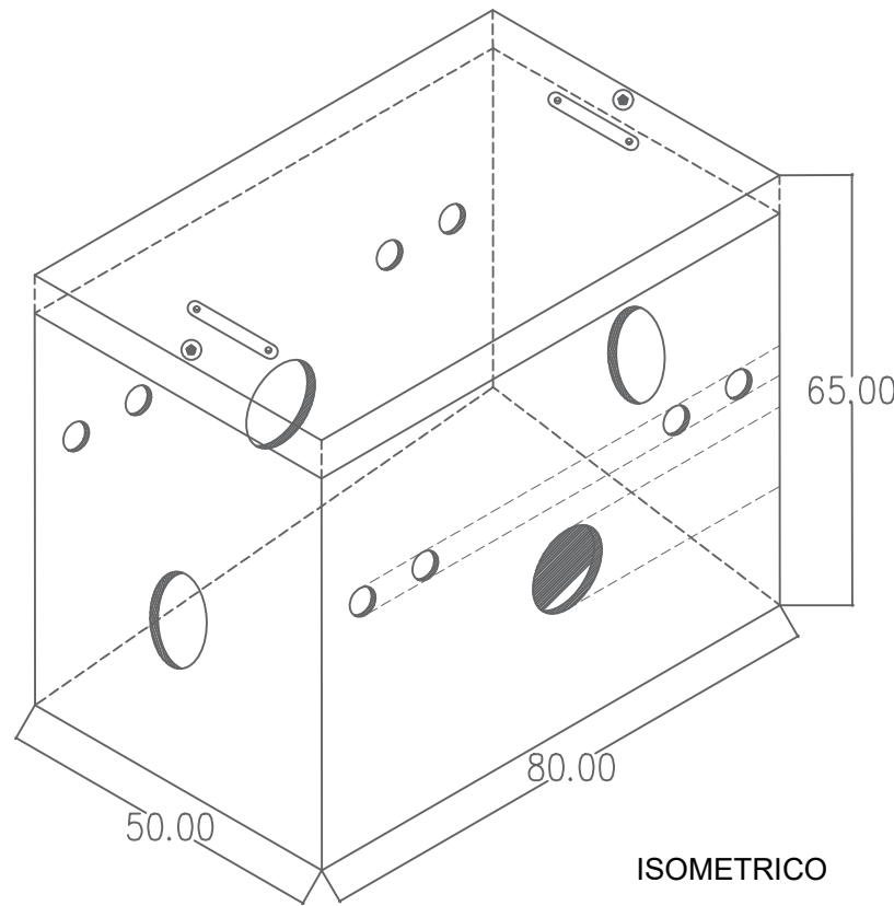
03 Detalle registro tipo 1 para BT IE-11 S/E
