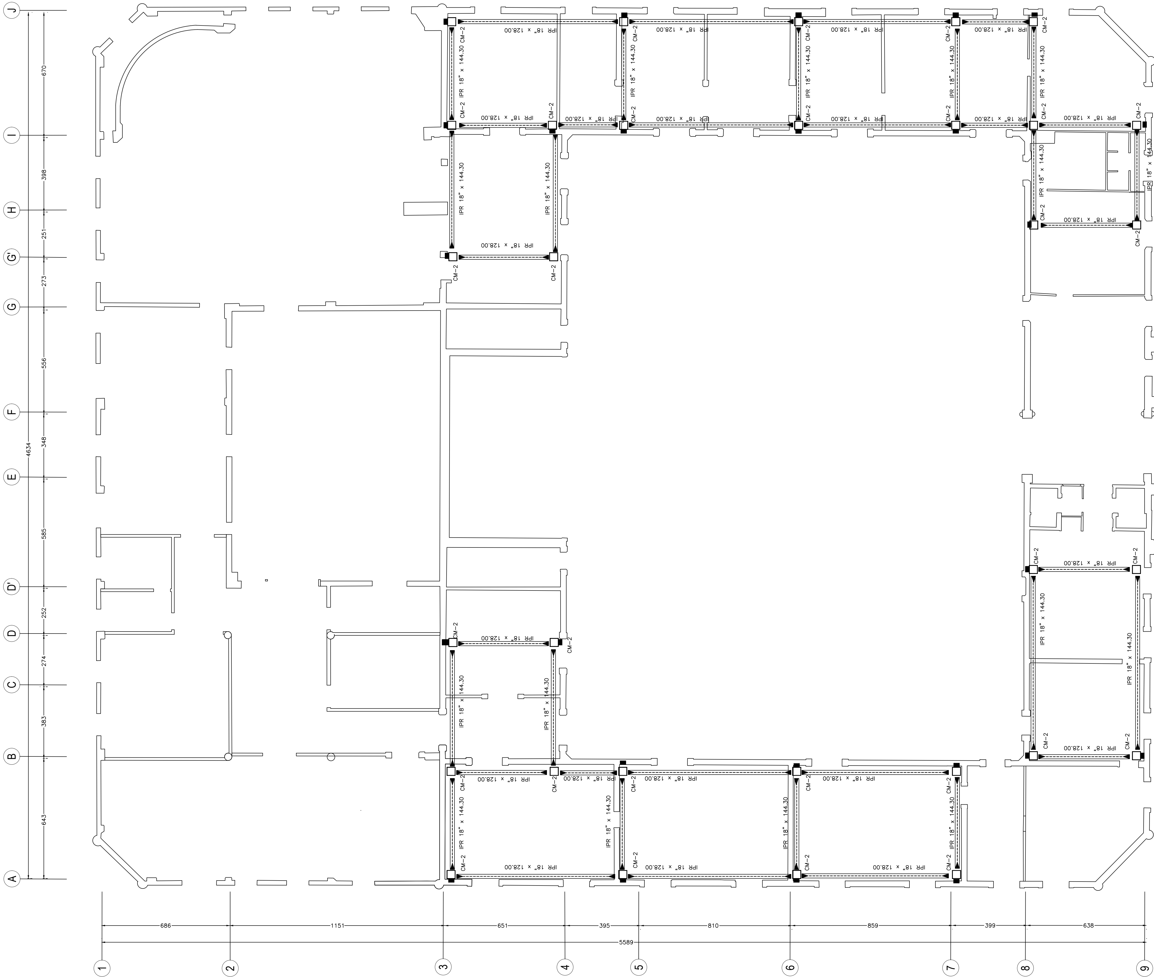
PLANTA ALTA REFUERZO ESTRUCTURAL PROPUESTO Esc: 1:100
