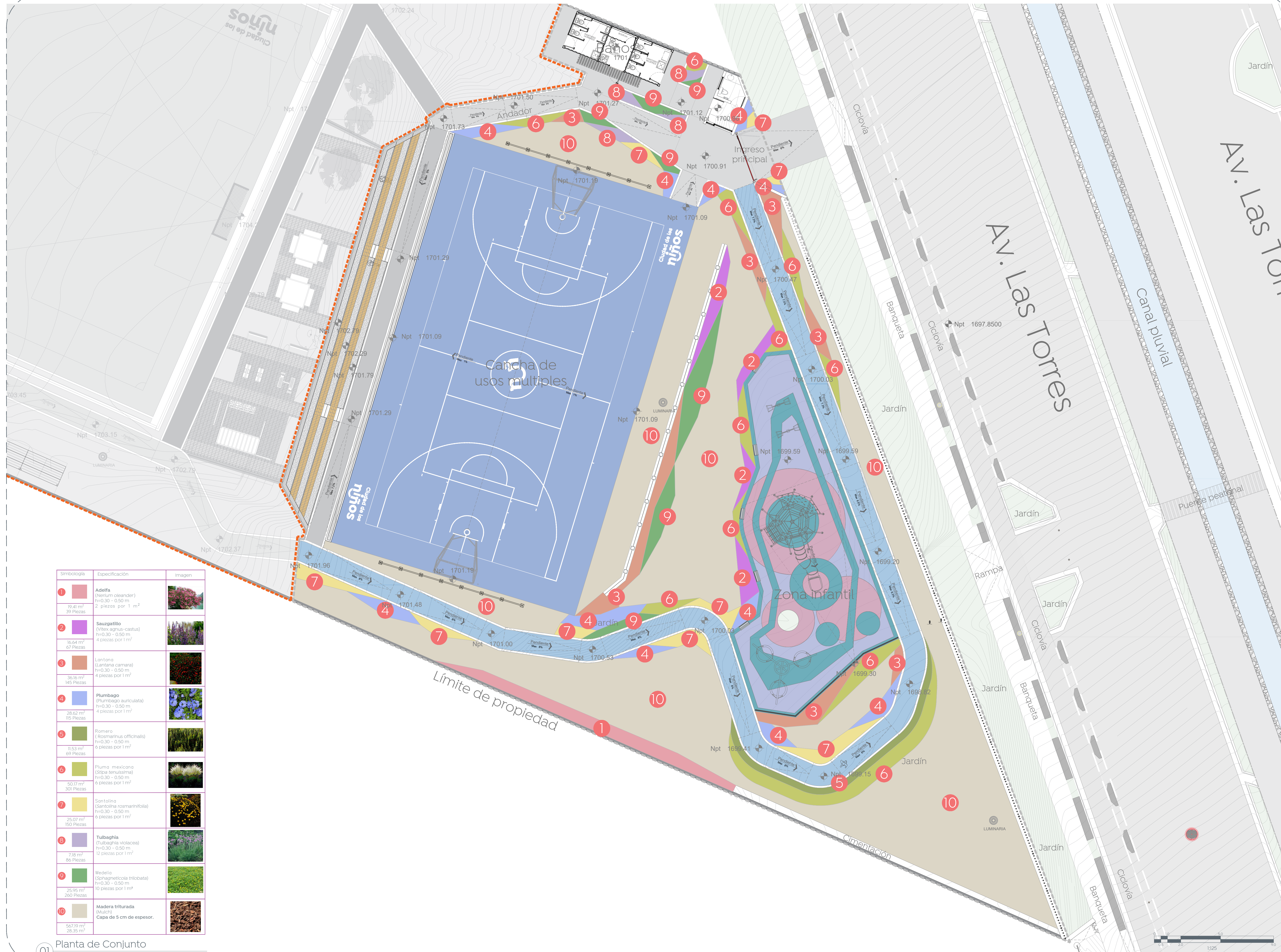
01 Planta de Conjunto
