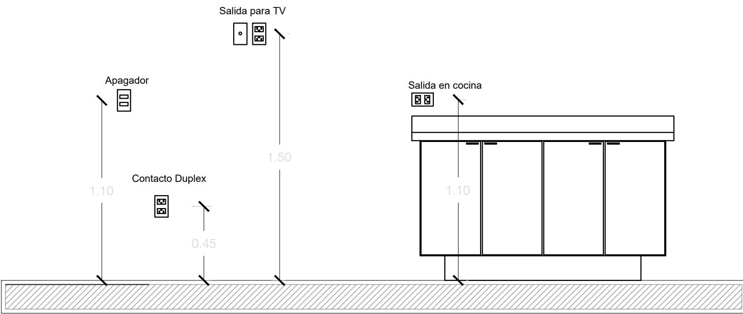
Detalle Altura de accesorios electricos
