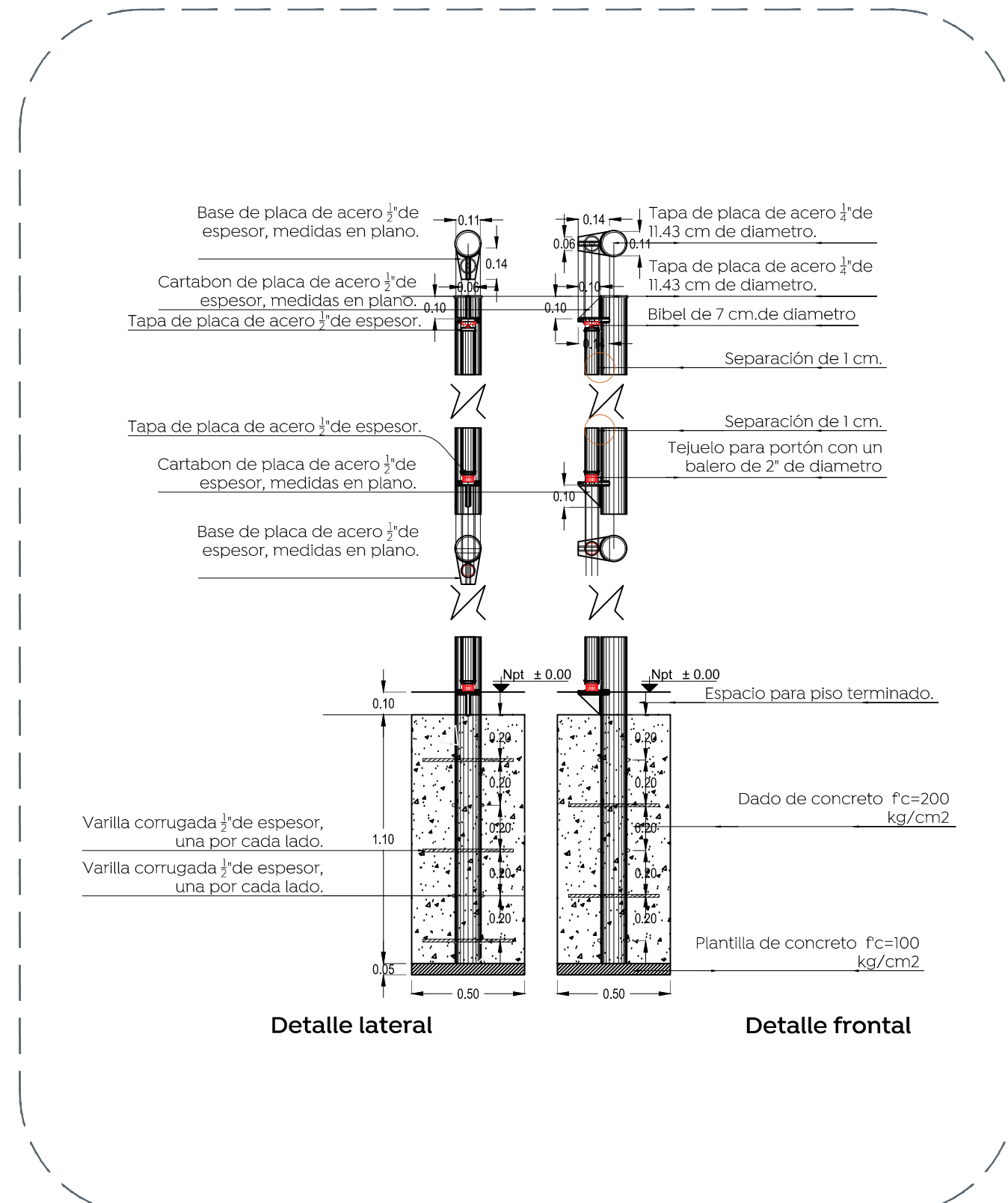
02 d-2 Detalle de instalación de Tejuelo y Bibel Albañilerías
