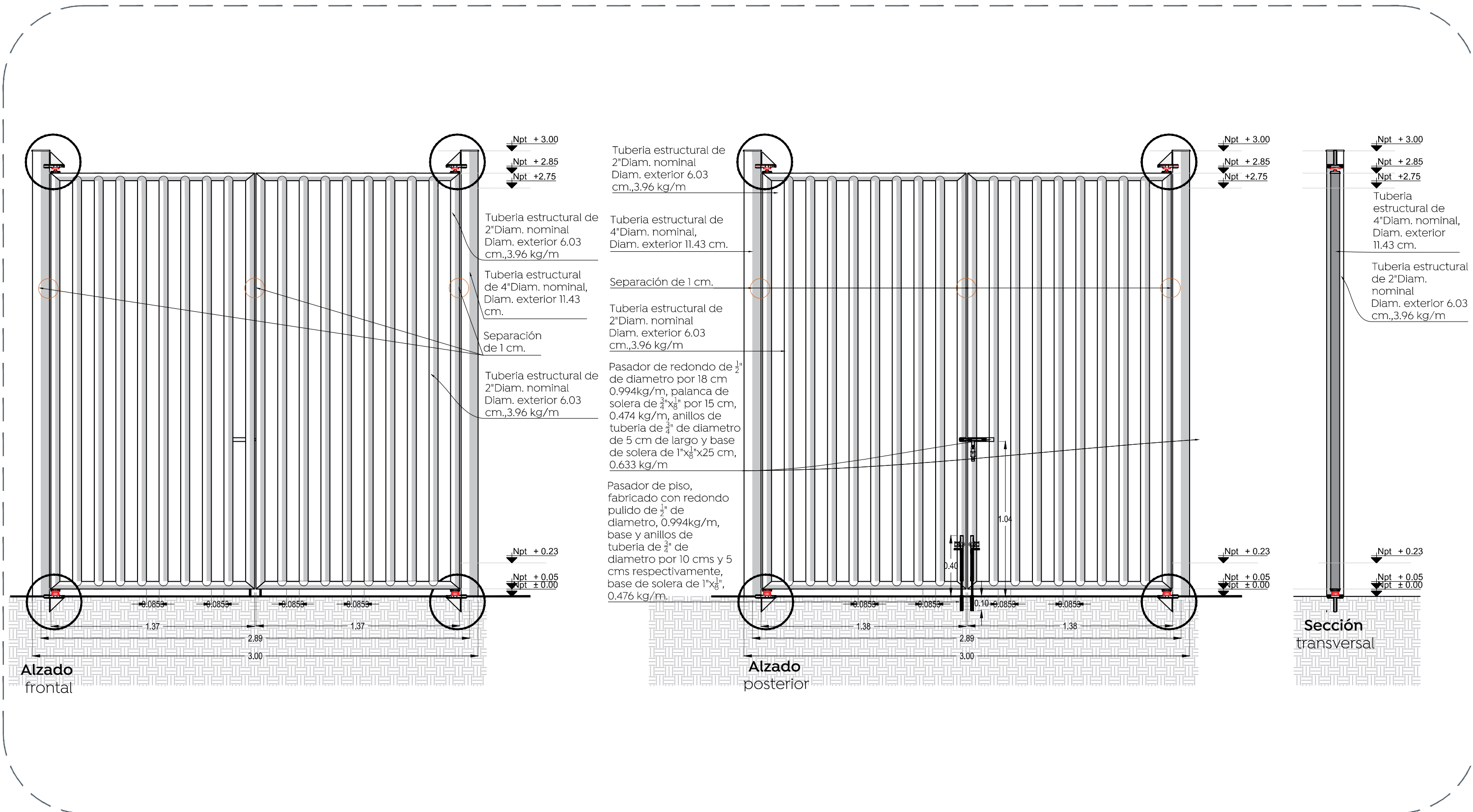
02 d-2 Portón de ingreso Albañilerías
