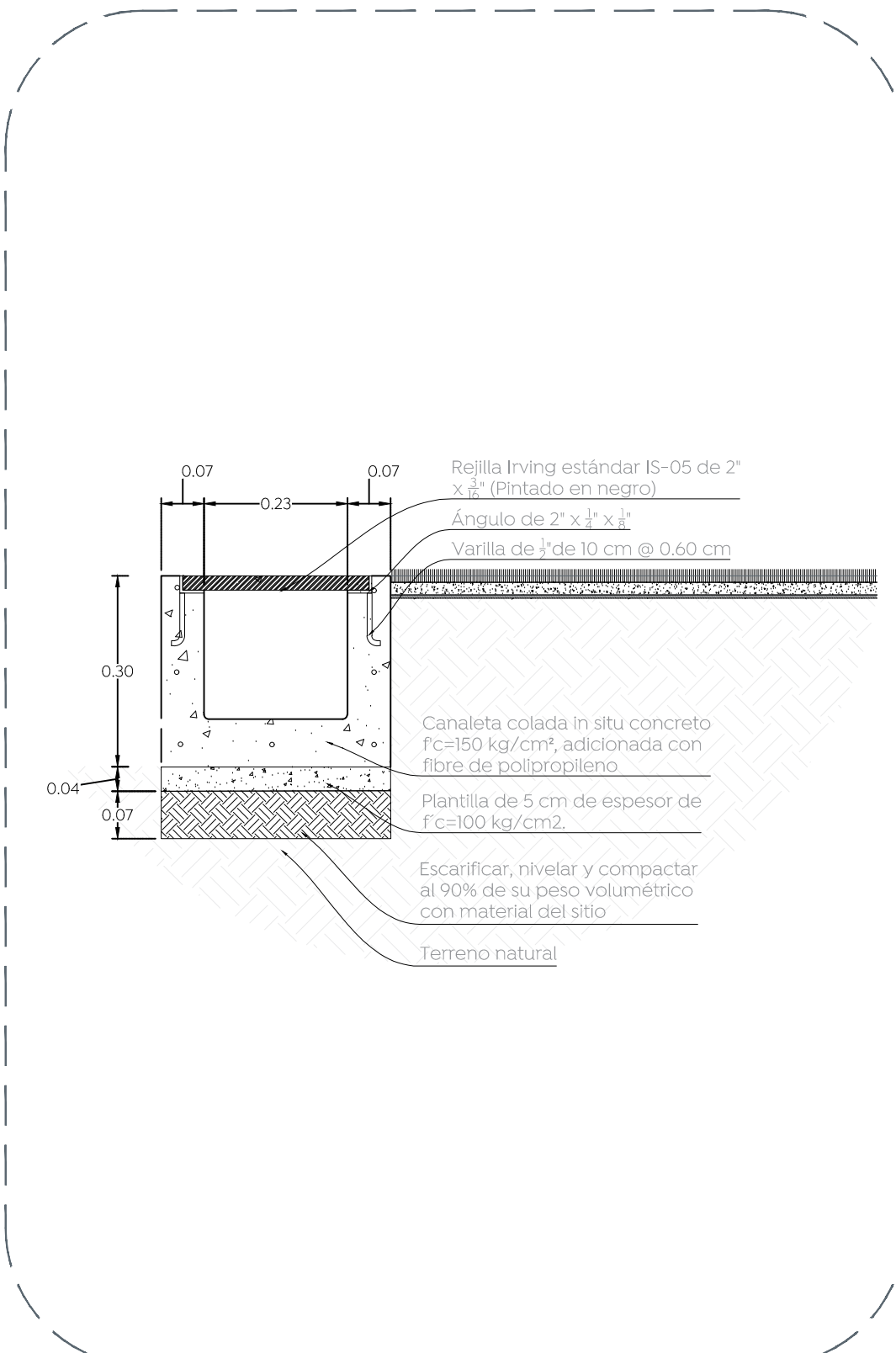
03 d-3 Detalle de canaleta en cancha Albañilerías
