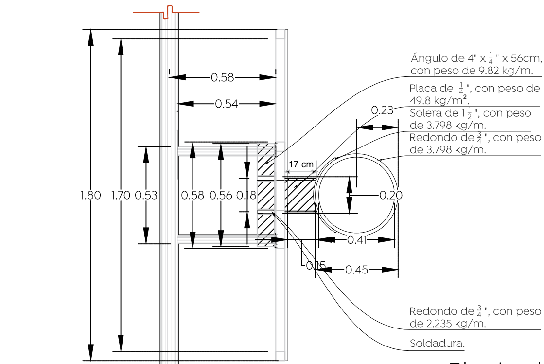
Planta de tablero
