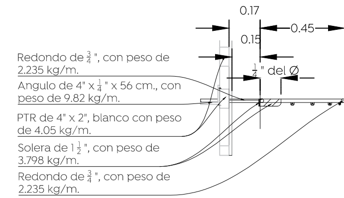
04 d-7 Detalle cancha de usos múltiples
