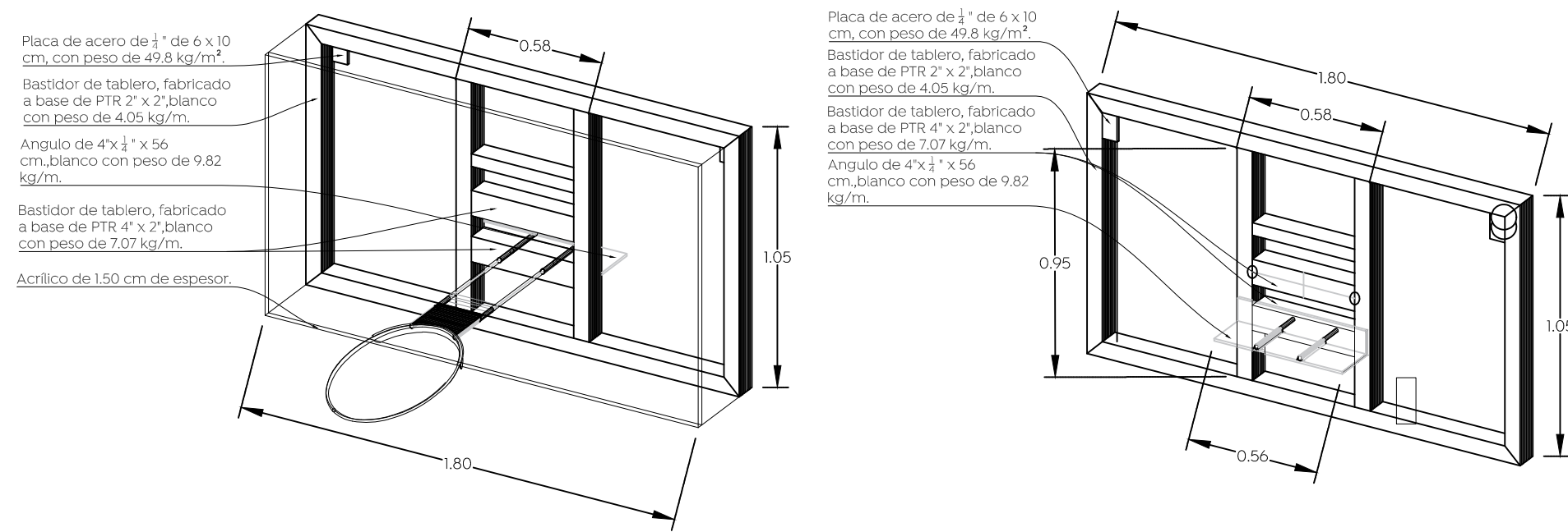
03 d-7 Detalle de tablero
