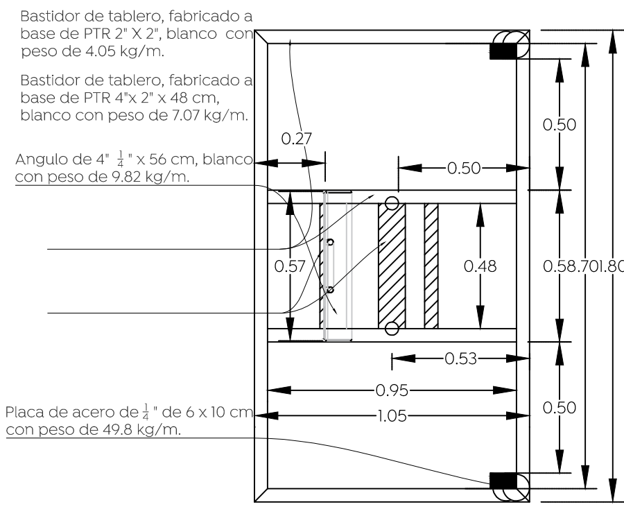
Planta de vista Posterior del tablero
