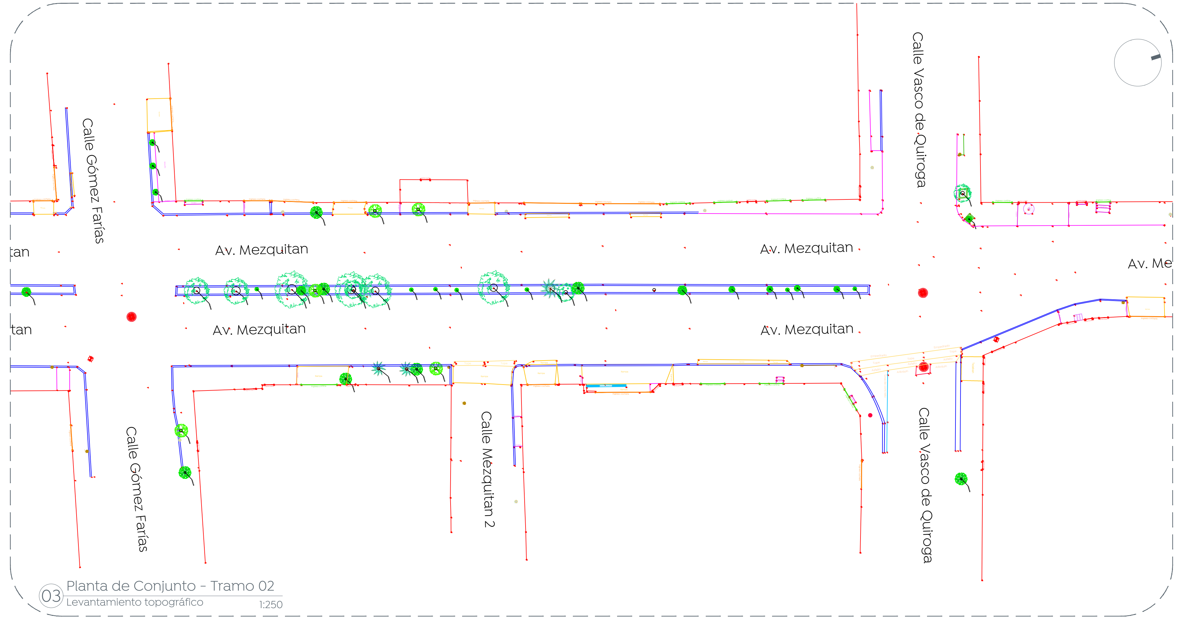
03 Planta de Conjunto - Tramo 02 Levantamiento topográfico 1:250
