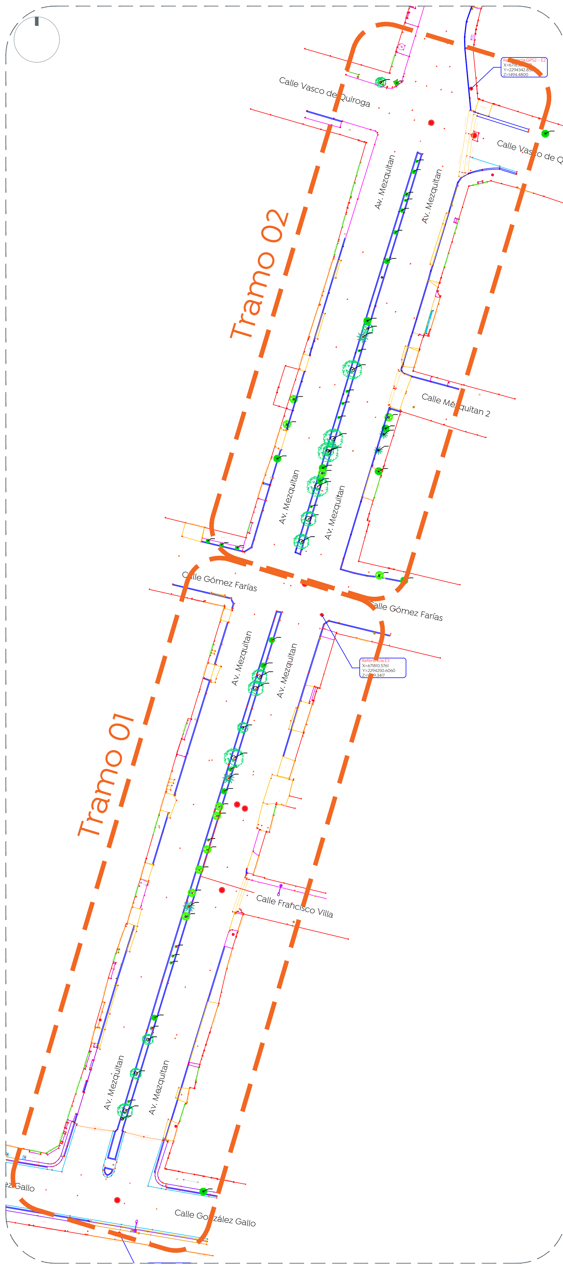
01 Planta de Conjunto - Ilave Levantamiento topográfico 1:400
