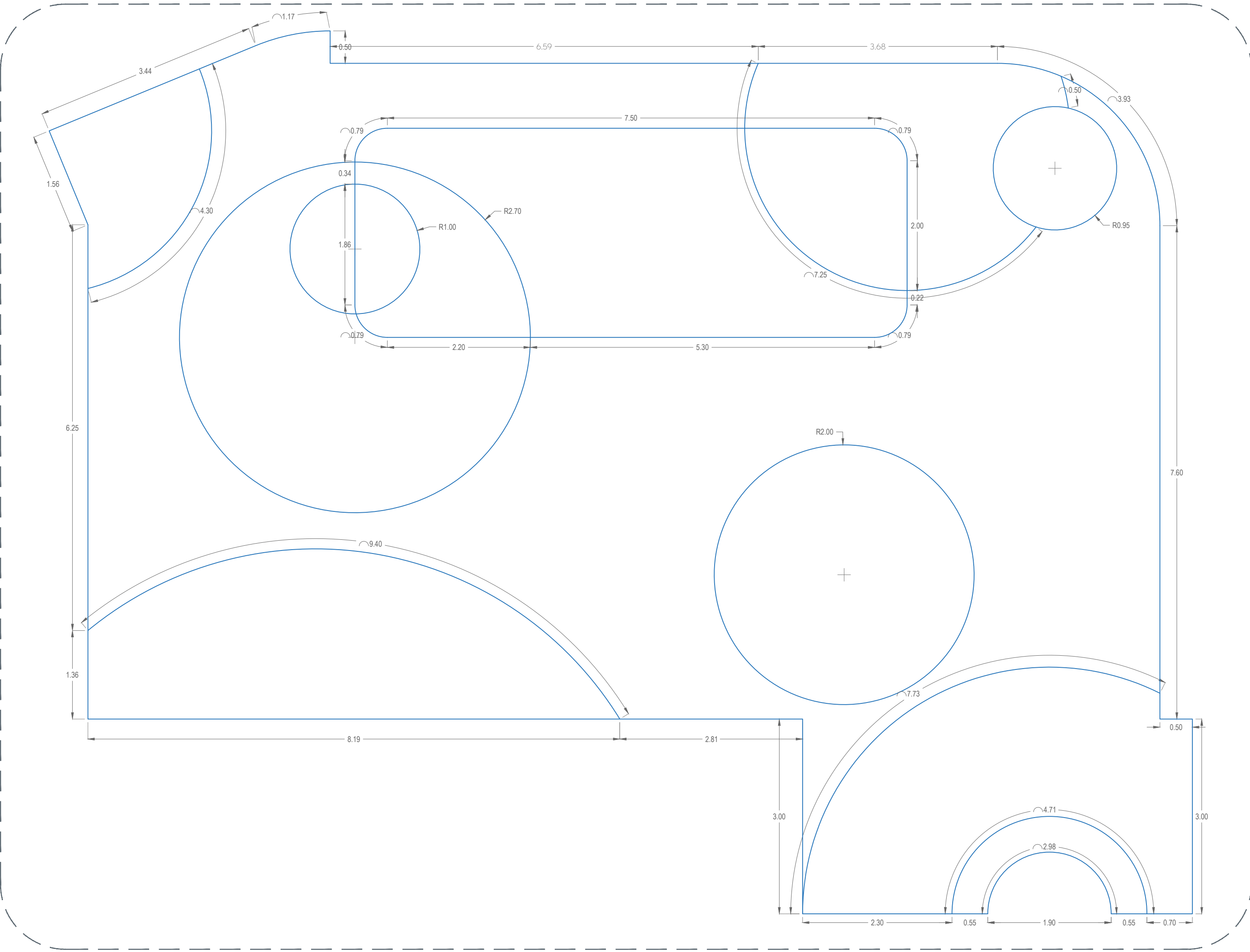
05 Trazo de piso amortiguante Acabados 1:50
