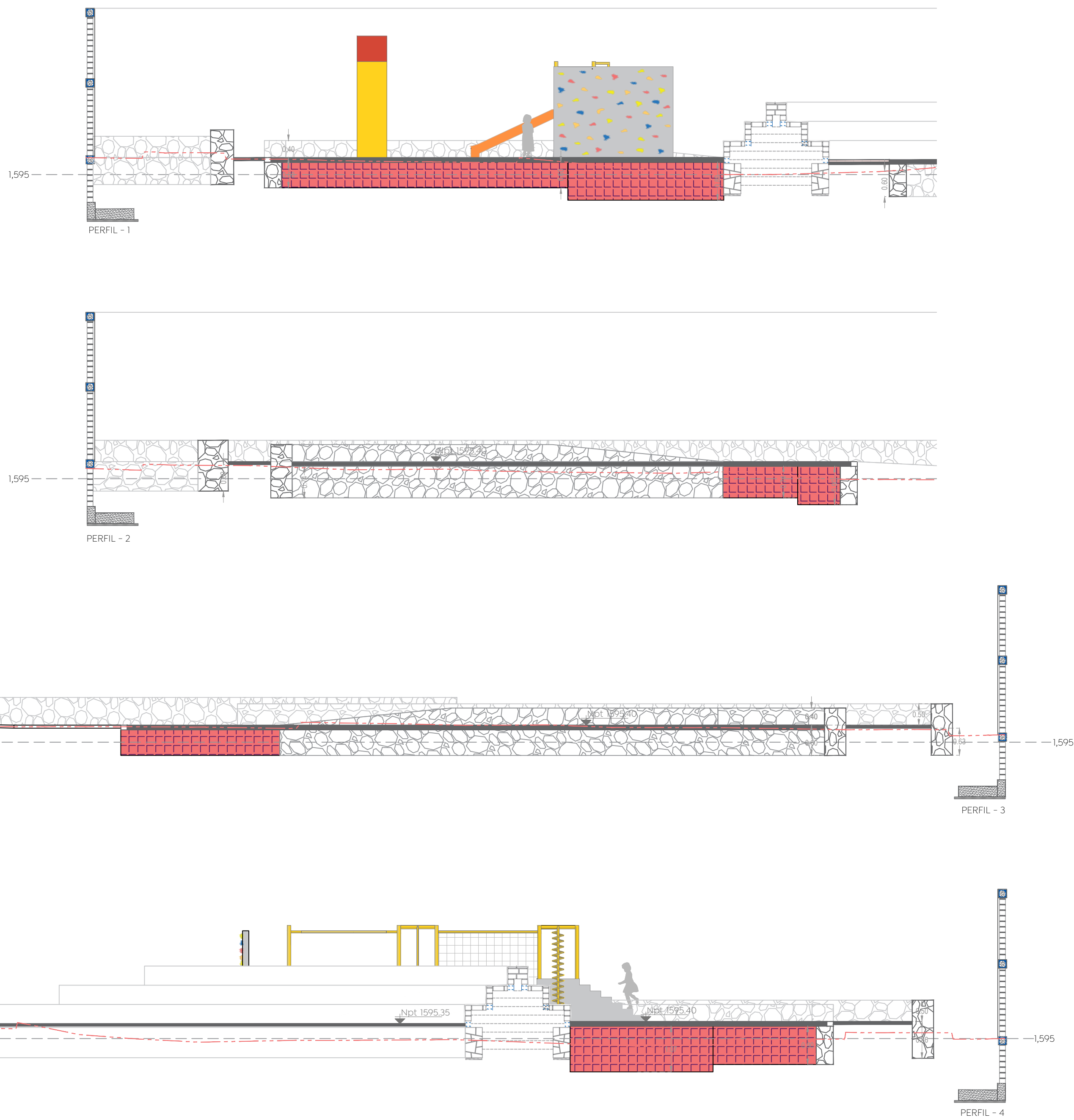
46 Secciones de muros de contención - área infantil Albañilerías 1:75
