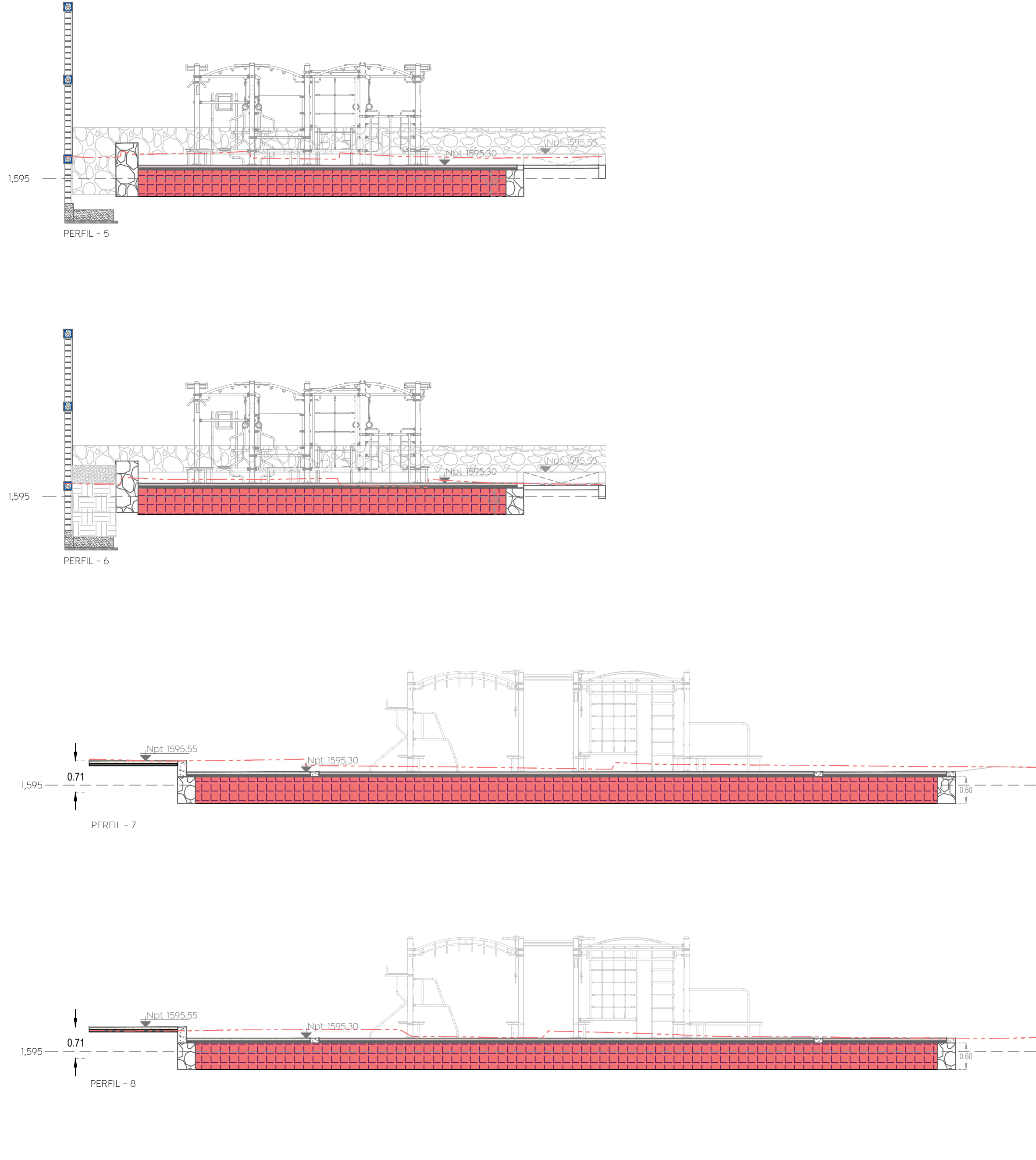
47 Secciones de muros de contención - GYM aire libre Albañilerías 1:75
