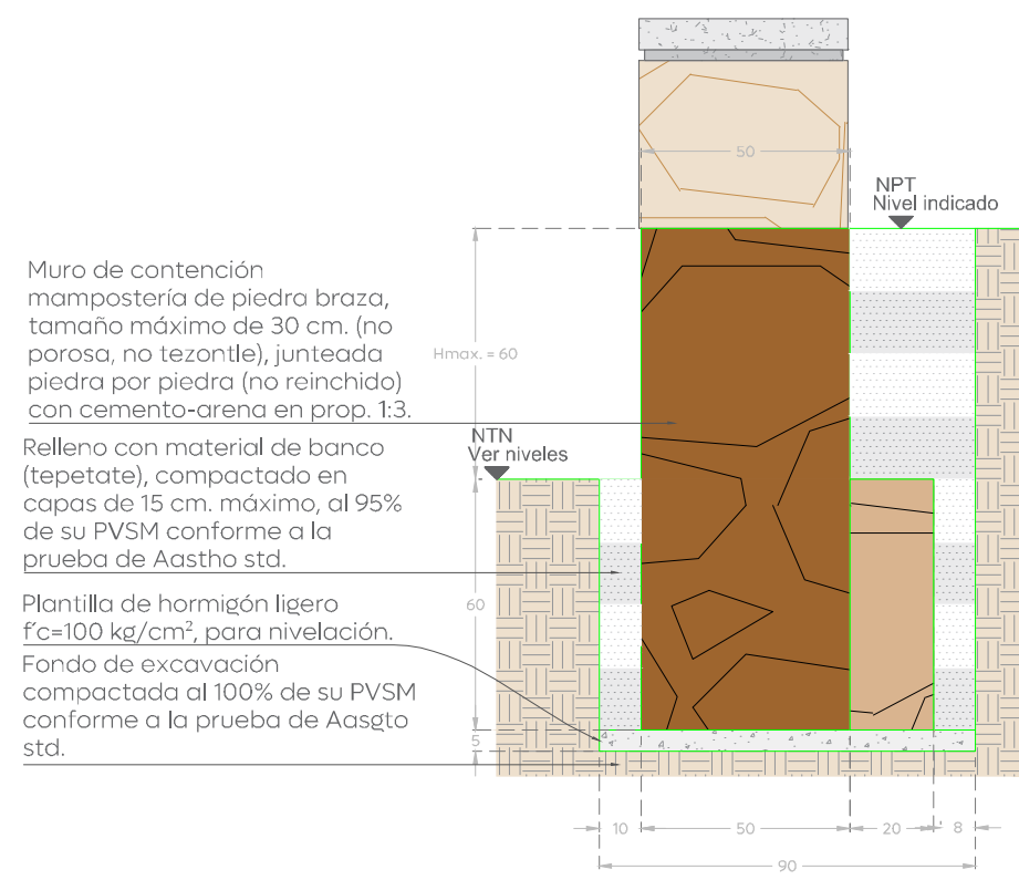
Muro de contención H. Max. =60 cm. Mampostería piedra braza Esc 1:20 Cotas: cm
