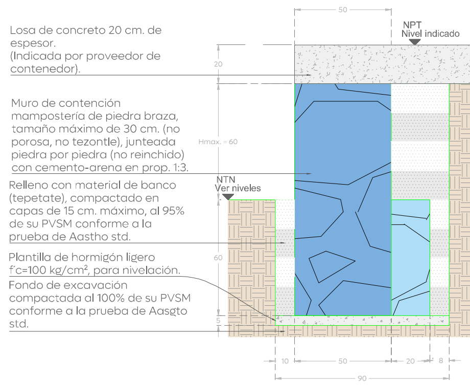
Muro de contención H. Max. =60 cm. Mampostería piedra braza Esc 1:20 Cotas: cm
