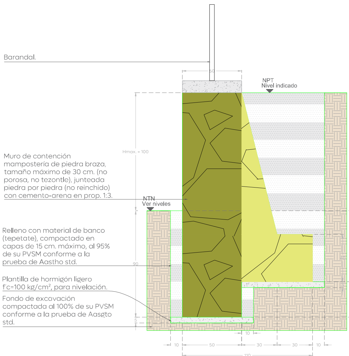
Muro de contención H. Max. =100cm. Mampostería piedra braza Esc 1:20 Cotas: cm
