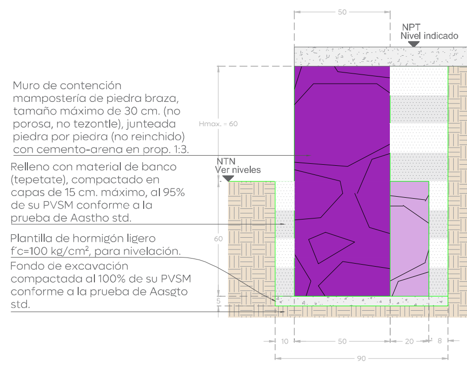
Muro de contención H. Max. =60 cm. Mampostería piedra braza Esc 1:20 Cotas: cm
