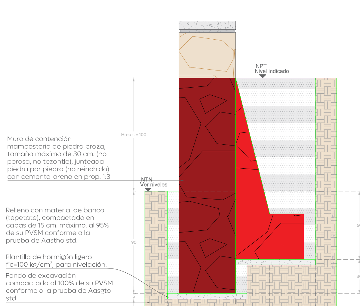
Muro de contención H. Max. =100cm. Mampostería piedra braza Esc 1:20 Cotas: cm
