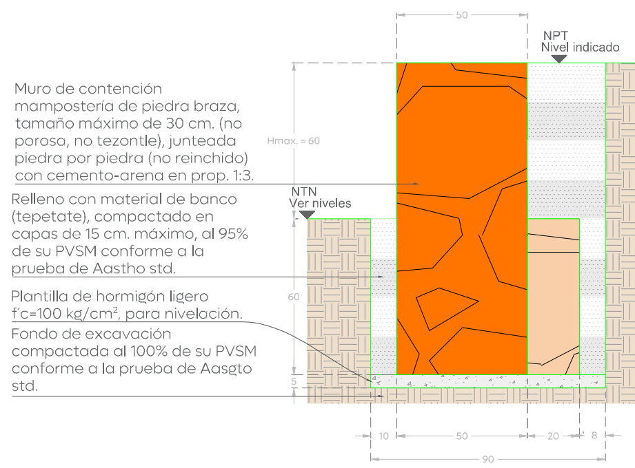
Muro de contención H. Max. =60 cm. Mampostería piedra braza Esc 1:20 Cotas: cm
