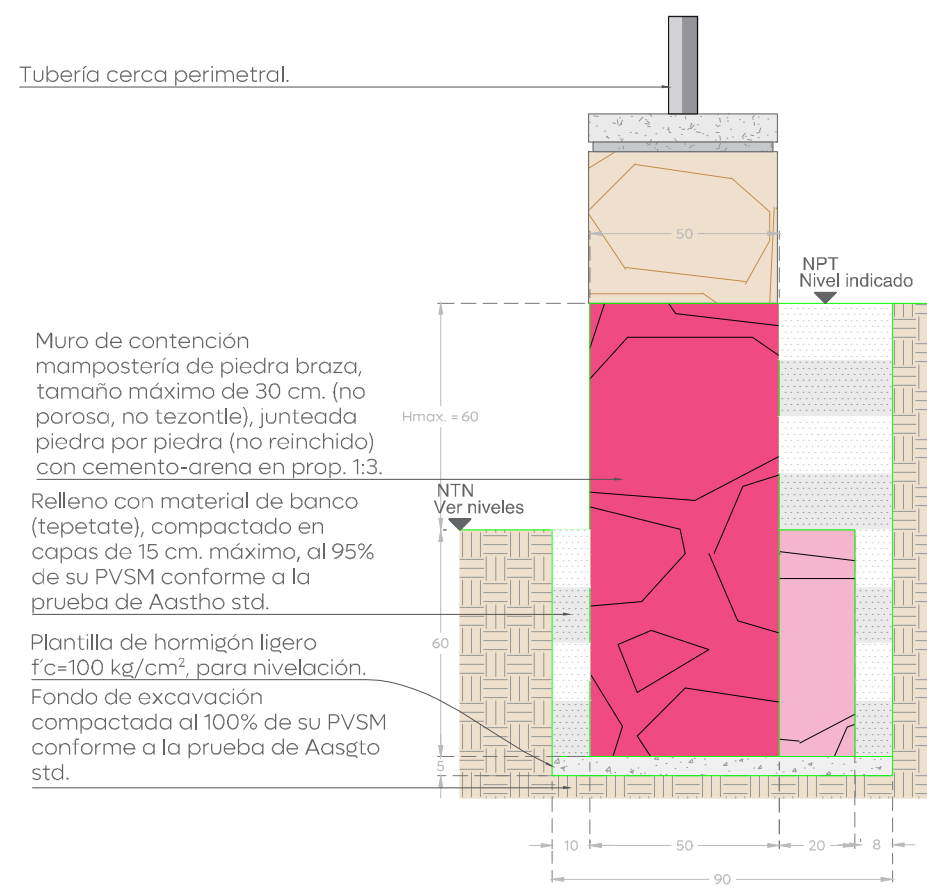
Muro de contención H. Max. =60 cm. Mampostería piedra braza Esc 1:20 Cotas: cm
