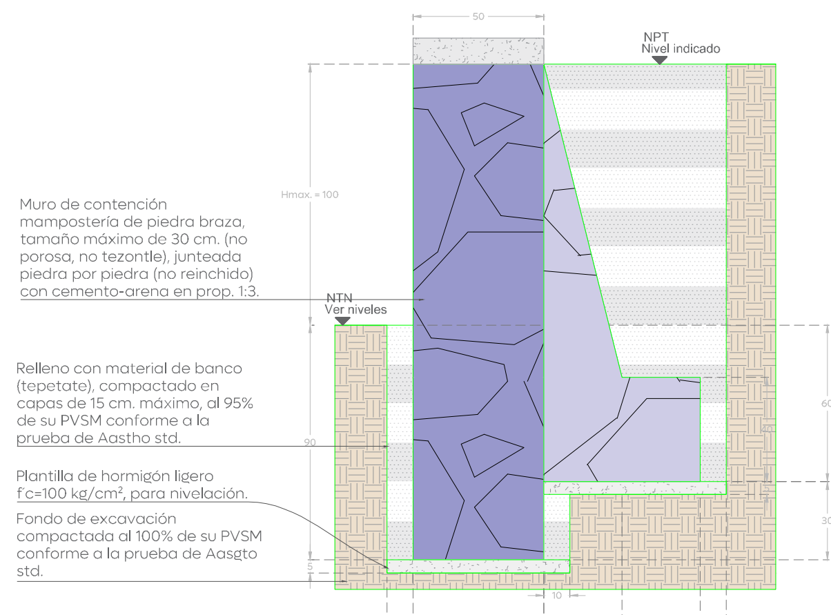
Muro de contención H. Max. =100cm. Mampostería piedra braza Esc 1:20 Cotas: cm
