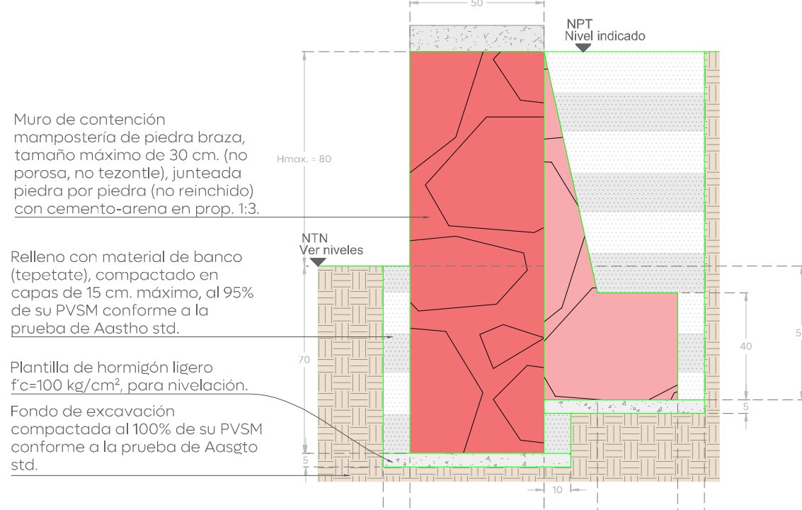
Muro de contención H. Max. =60 cm. Mampostería piedra braza Esc 1:20 Cotas: cm
