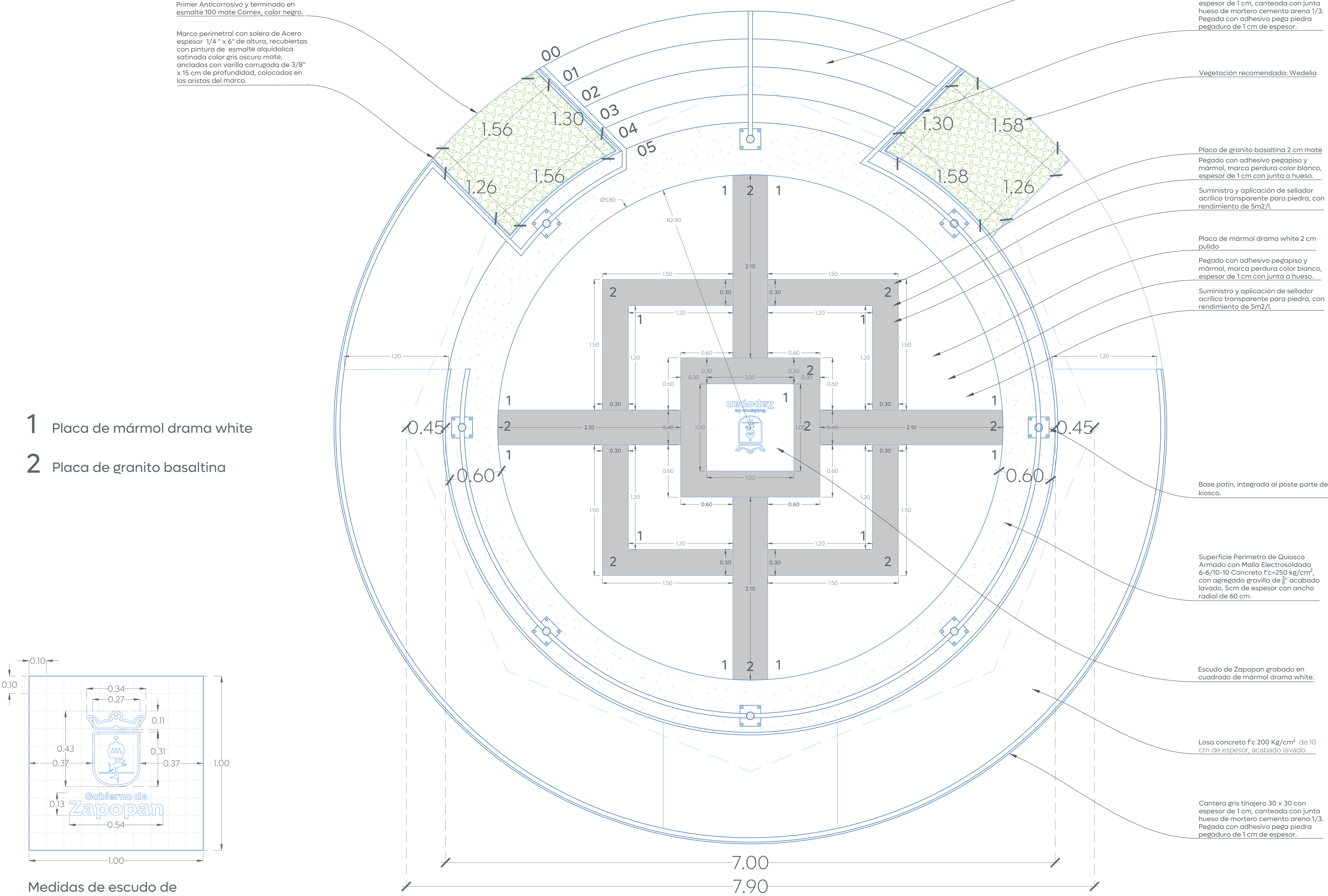
Medidas de escudo de Zapopan grabado Esc. 1:50
